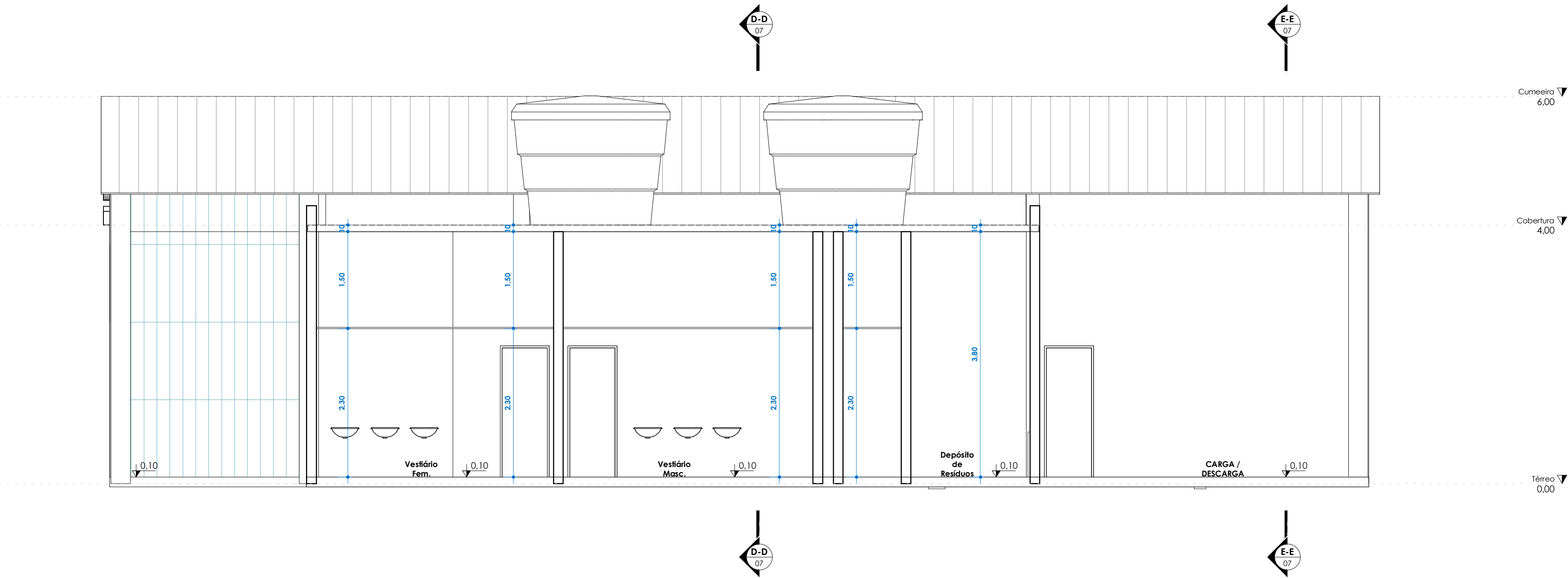
1 C-C 1 : 50
