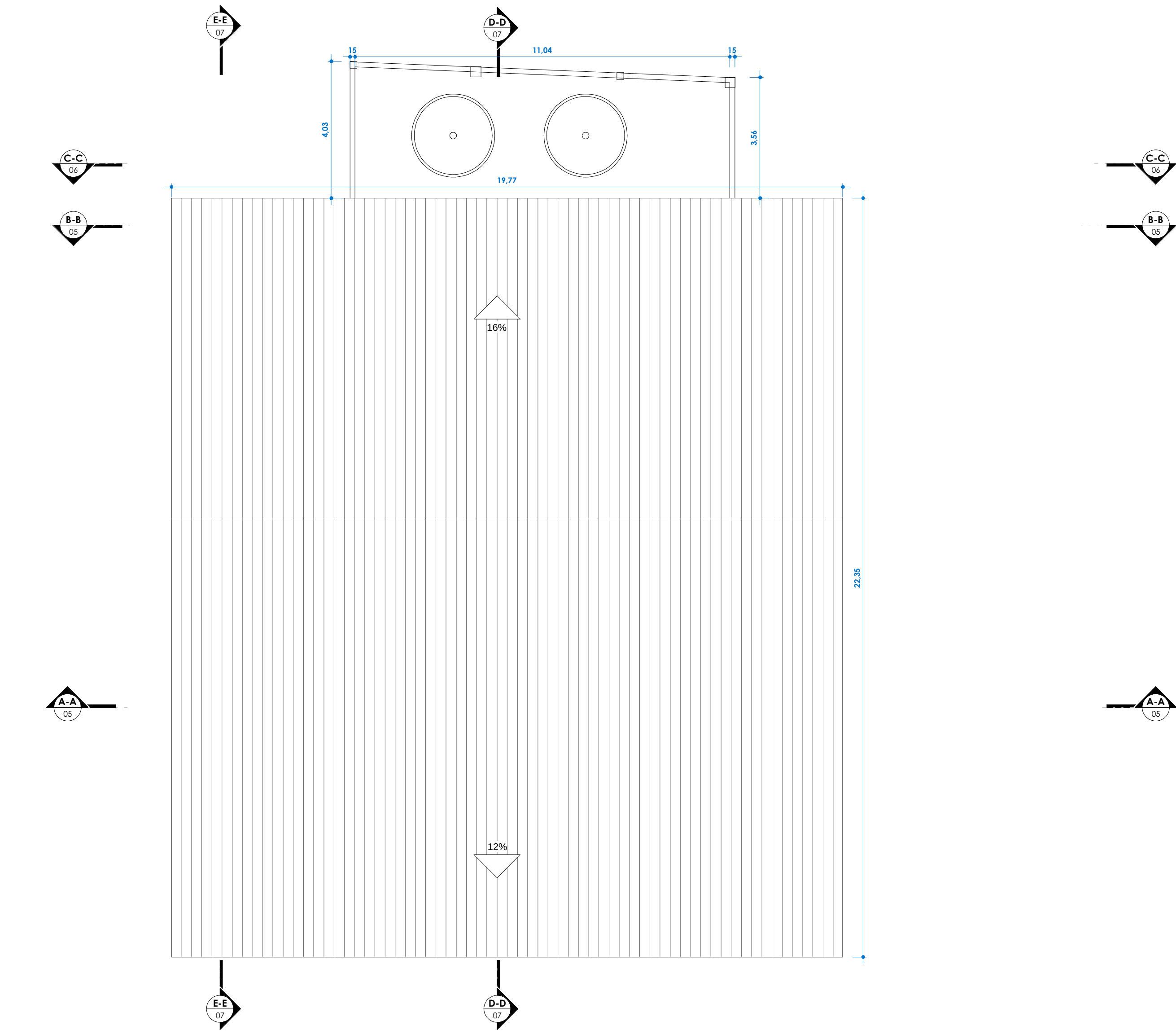
1 Cobertura 1 : 100
