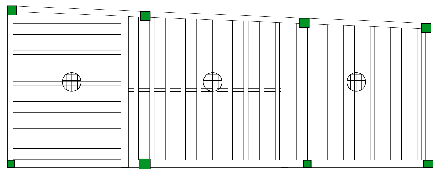
Planta de vigotas pré-moldadas
