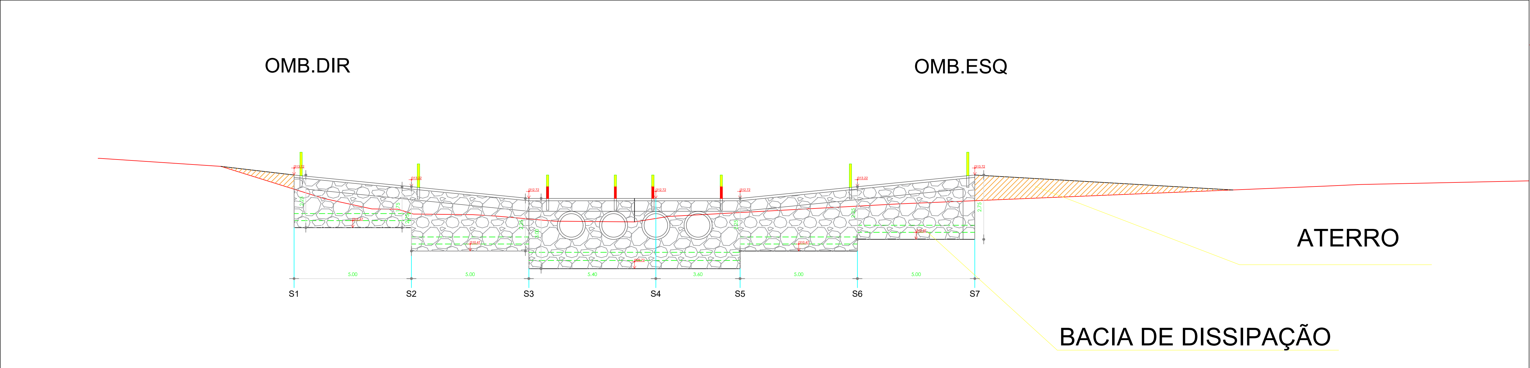
PERFIL LONGITUDINAL DO EIXO DA PASSAGEM MOLHADA ESCALA - V: 1/100 H: 1/100
