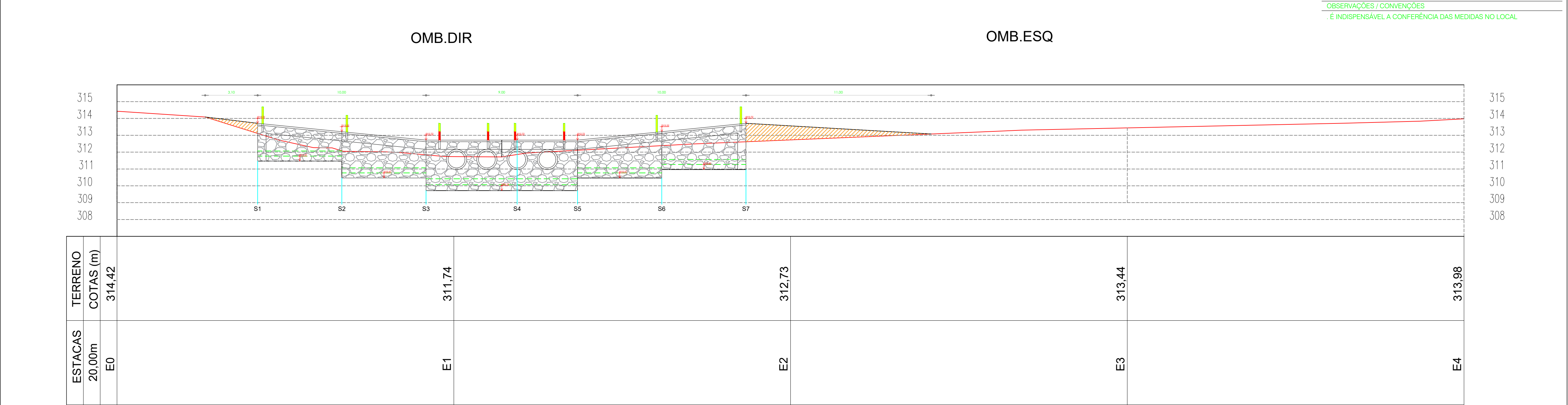
PERFIL LONGITUDINAL DO EIXO DA PASSAGEM MOLHADA ESCALA - V: 1/100 H: 1/100
