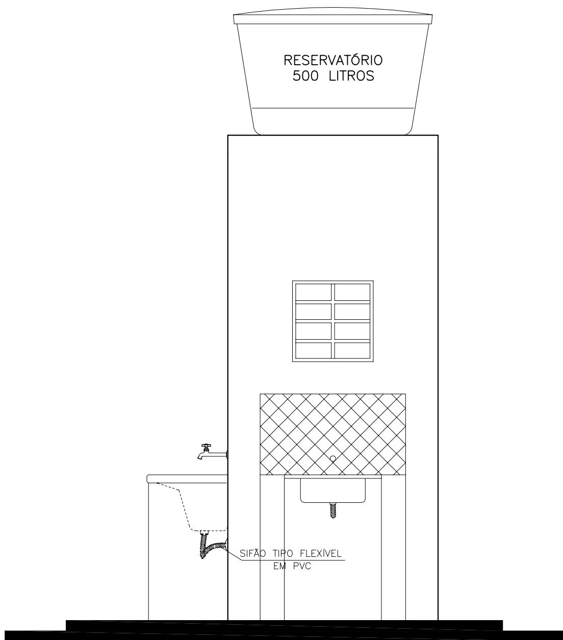
FACHADA C
