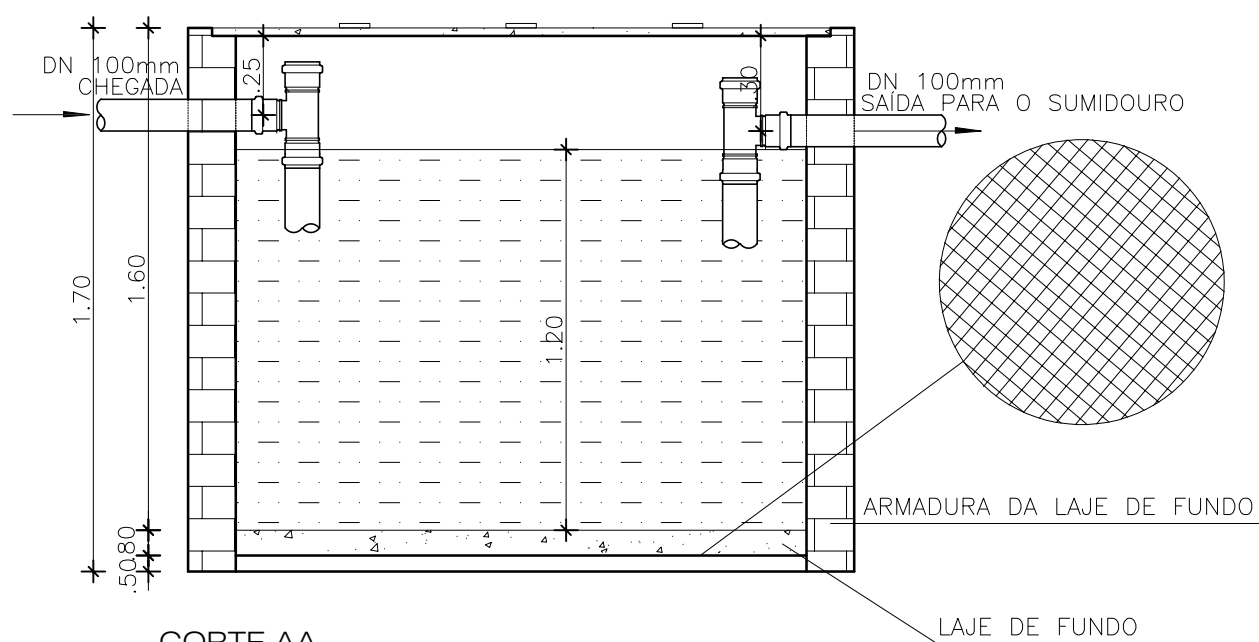
CORTE AA
