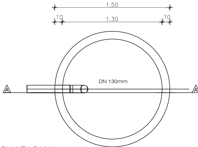
PLANTA BAIXA
