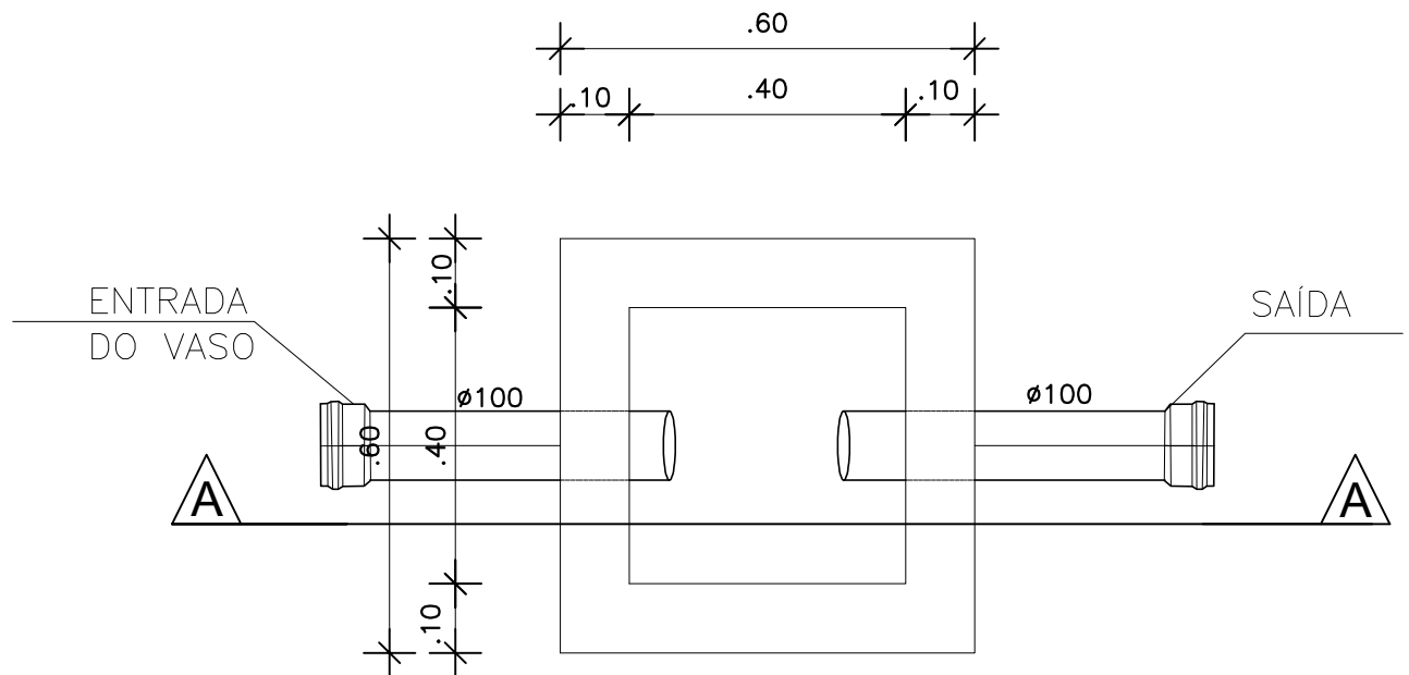
PLANTA BAIXA
