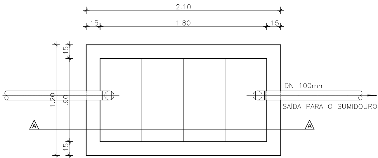
PLANTA BAIXA
