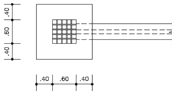
VISTA SUPERIOR
