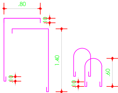
ARMAÇÃO CAIXA DE REGISTRO
