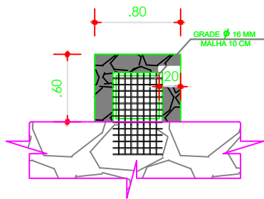
VISTA SUPERIOR CAIXA DA MONTANTE
