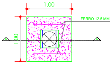
VISTA SUPERIOR CAIXA DE REGISTRO
