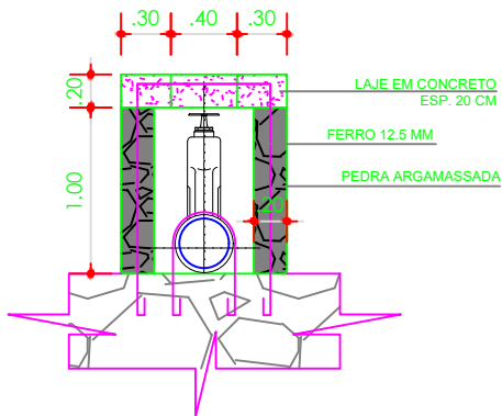
CORTE AA CAIXA DE REGISTRO
