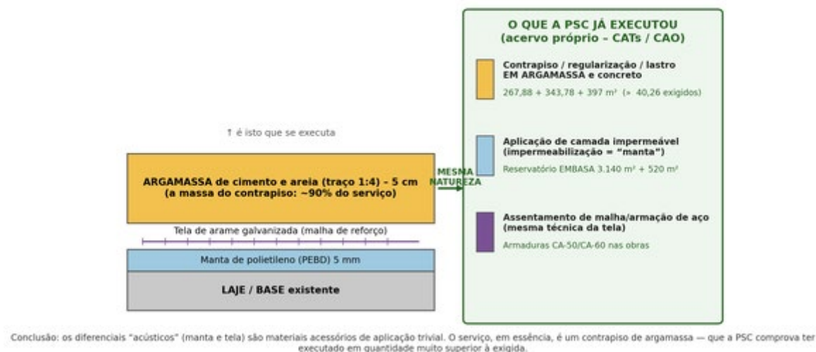
Figura 1 – Composição real do “contrapiso acústico” (SINAPI 90932) e correspondência com o acervo da Recorrente.
