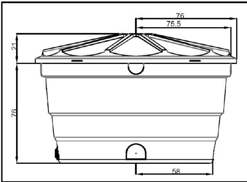
Fig. 2: Dimensões da caixa d'água de 1000 L
