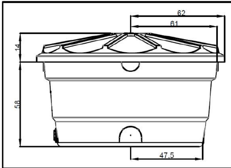
Fig. 1: Dimensões da caixa d'água de 500 L
