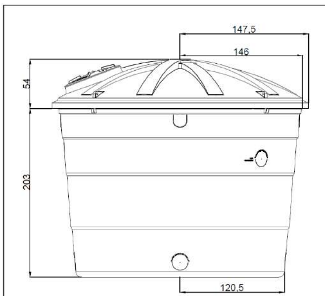
Fig. 4: Dimensões da caixa d'água de 10000 L
