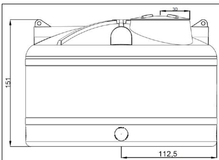
Fig. 5: Dimensões do tanque de 5000 L
