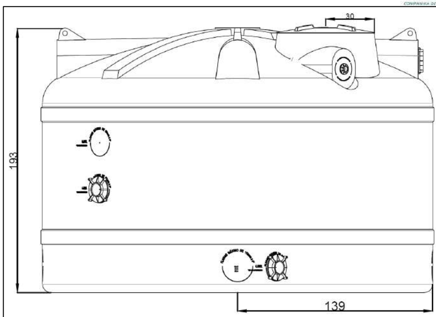
Fig. 6: Dimensões do tanque de 10000 L
