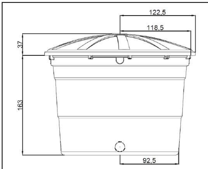
Fig. 3: Dimensões da caixa d'água de 5000 L
