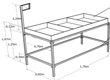
DIMENSIONAMENTO ESTRUTURAL ESCALA 1/50
