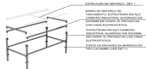
DIAGRAMA DE MONTAGEM ESCALA 1/50
