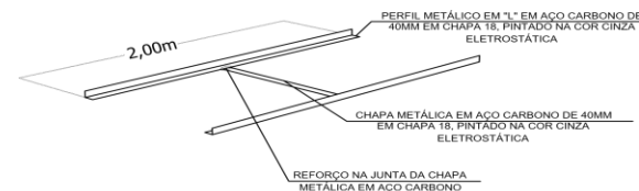
ESTRUTURA DE REFORÇO - DET. 01 S/ ESCALA
