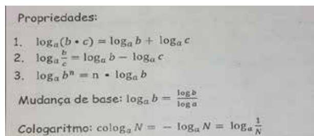
Figura 3: Propriedades operatórias dos logaritmos
