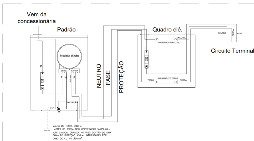
Figura 03 – Esquema TN-S_Detalhe da instalação do medidor de energia e do Quadro de distribuição Sistema Bifásico Fonte: Elaborado pelo autor, SUDESB (2023).
