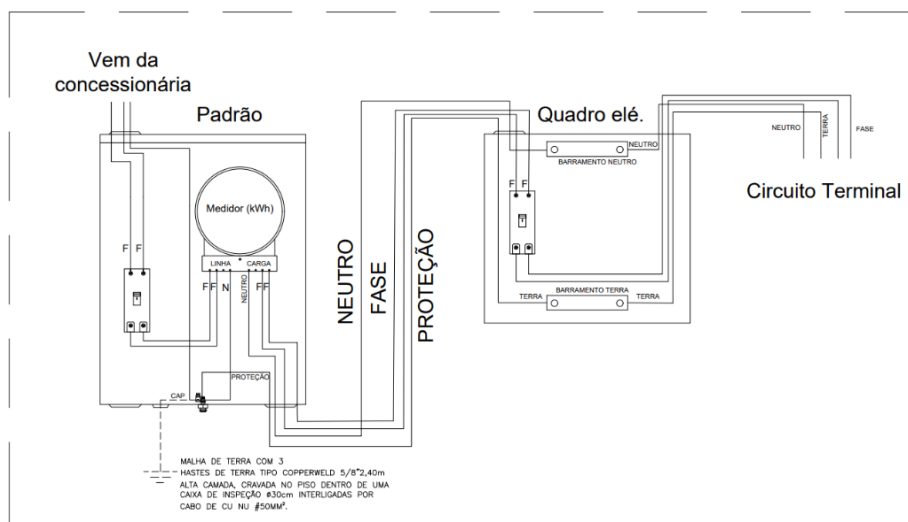
Figura 03 – Esquema TN-S_Detalhe da instalação do medidor de energia e do Quadro de distribuição Sistema Bifásico
