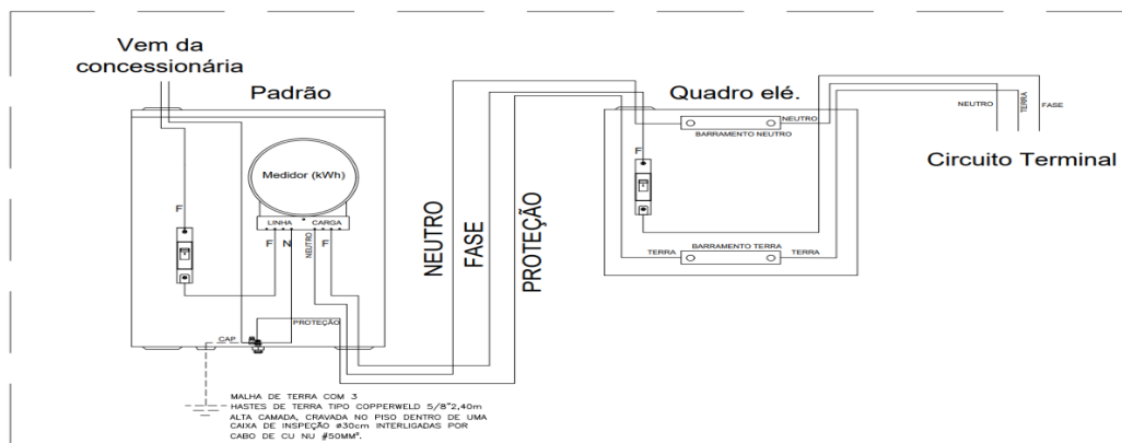
Figura 02– Esquema TN-S_Detalhe da instalação do medidor de energia e do Quadro de distribuição Sistema Monofásico
