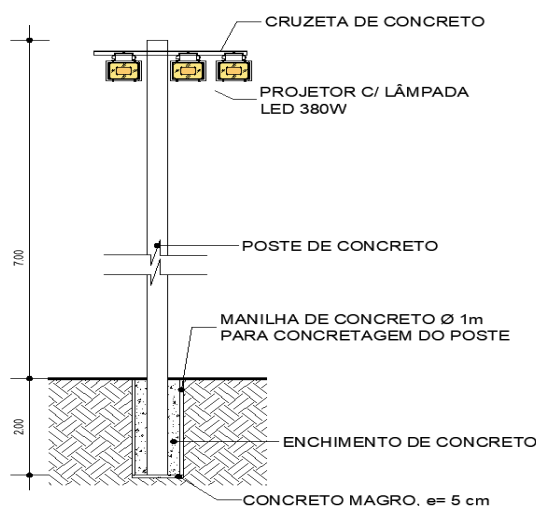
Figura 04– Vista frontal do sistema de iluminação em LED Fonte: Elaborado pelo autor, SUDESB (2023).
