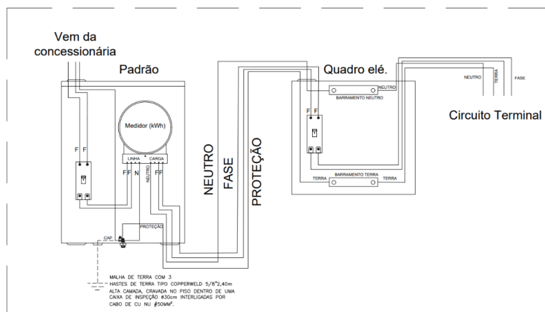
Figura 02– Esquema TN-S_Detalhe da instalação do medidor de energia e do Quadro de distribuição Sistema Monofásico Fonte: Elaborado pelo autor, SUDESB (2023).
