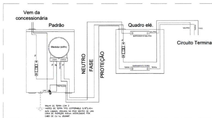
Figura 02- Esquema da instalação do
