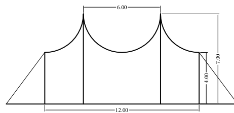
CORTE C-C
