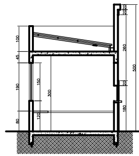
CORTE FF
