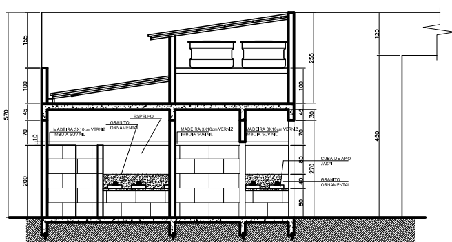
CORTE CC ESCALA 1:50
