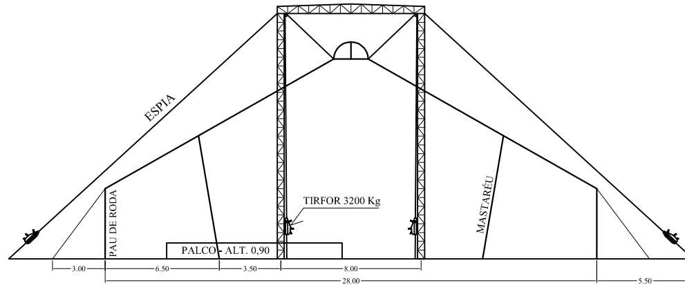
CORTE B-B
