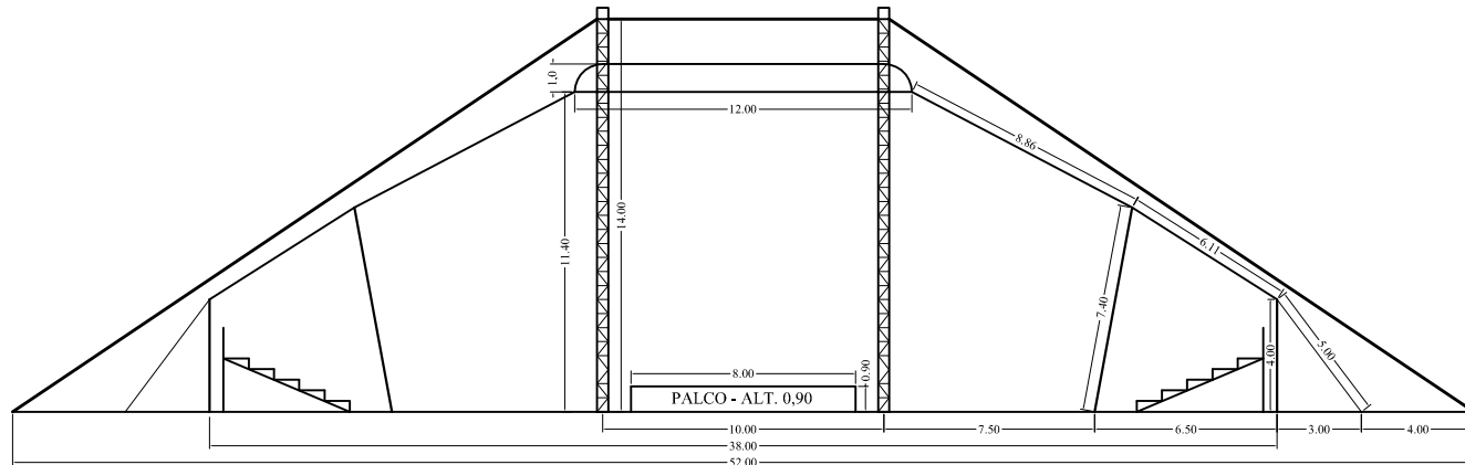
CORTE A-A
