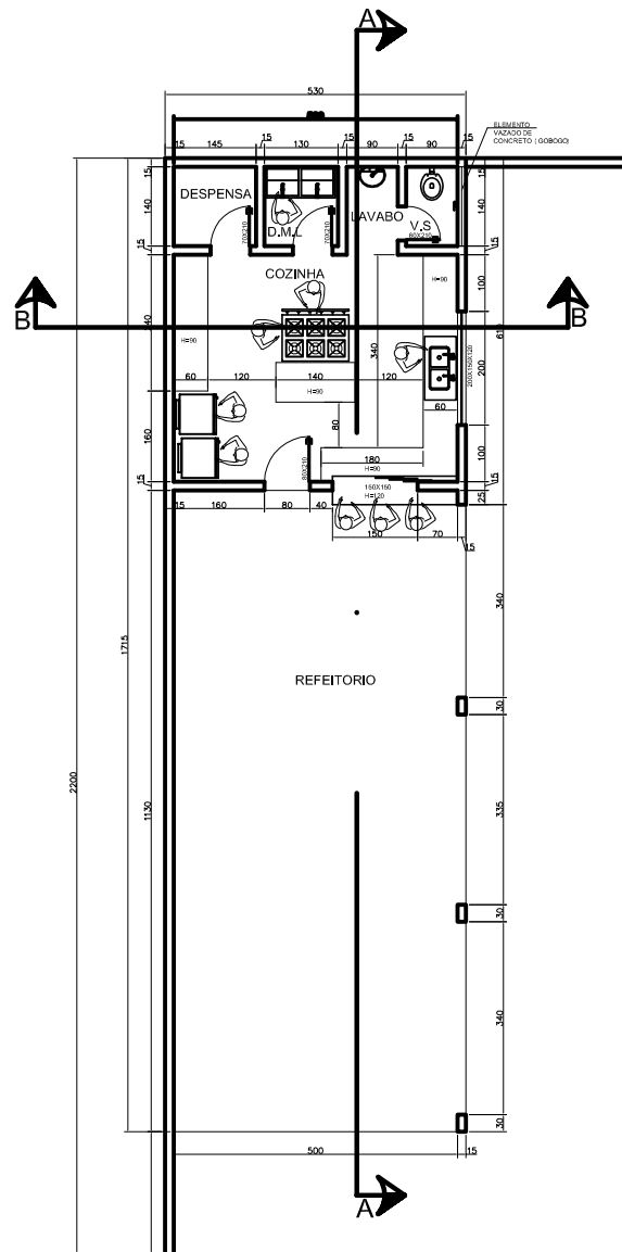
PLANTA BAIXA COZINHA/REFEITÓRIO ESC. 1:50 ÁREA = 90,89m 2
