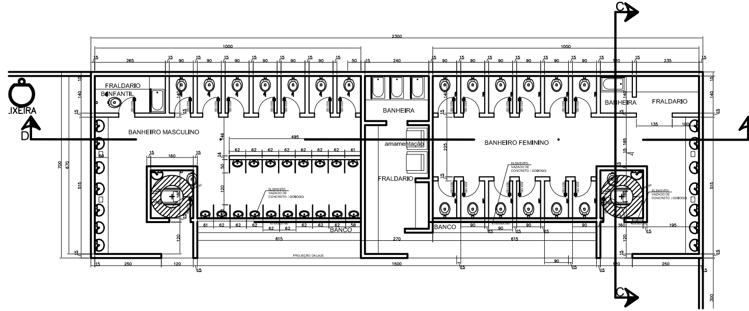
PLANTA BAIXA- BANHEIROS USUÁRIOS ESC. 1:50 ÁREA = 161,00m 2
