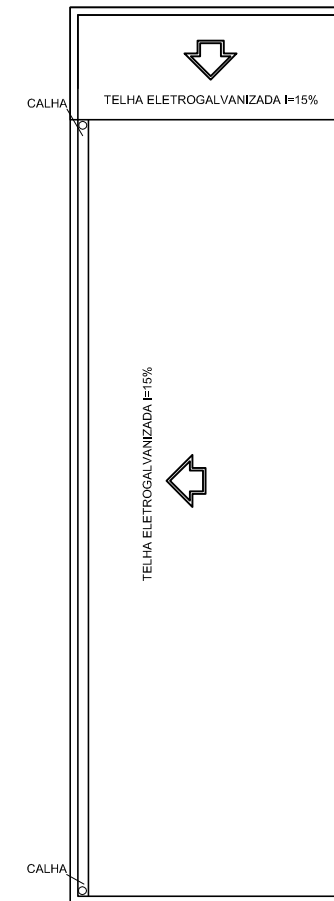
PLANTA DE COBERTURA DA COZINHA/REFEITÓRIO ESCALA 1:50
