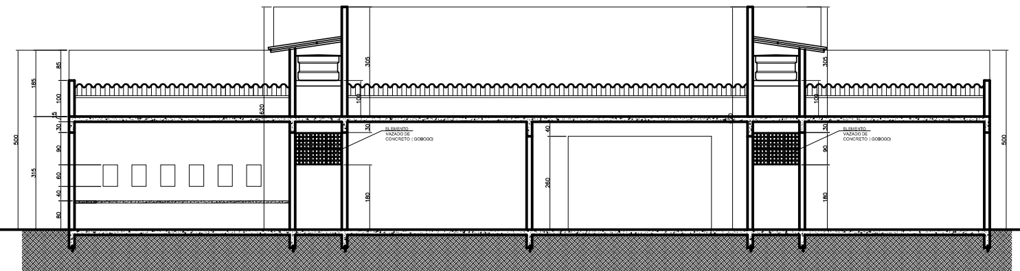
CORTE EE
