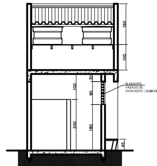
CORTE GG
