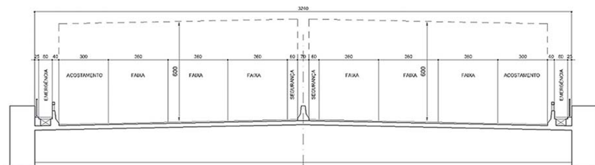
Perfil transversal tipo do tabuleiro – trecho convencional
