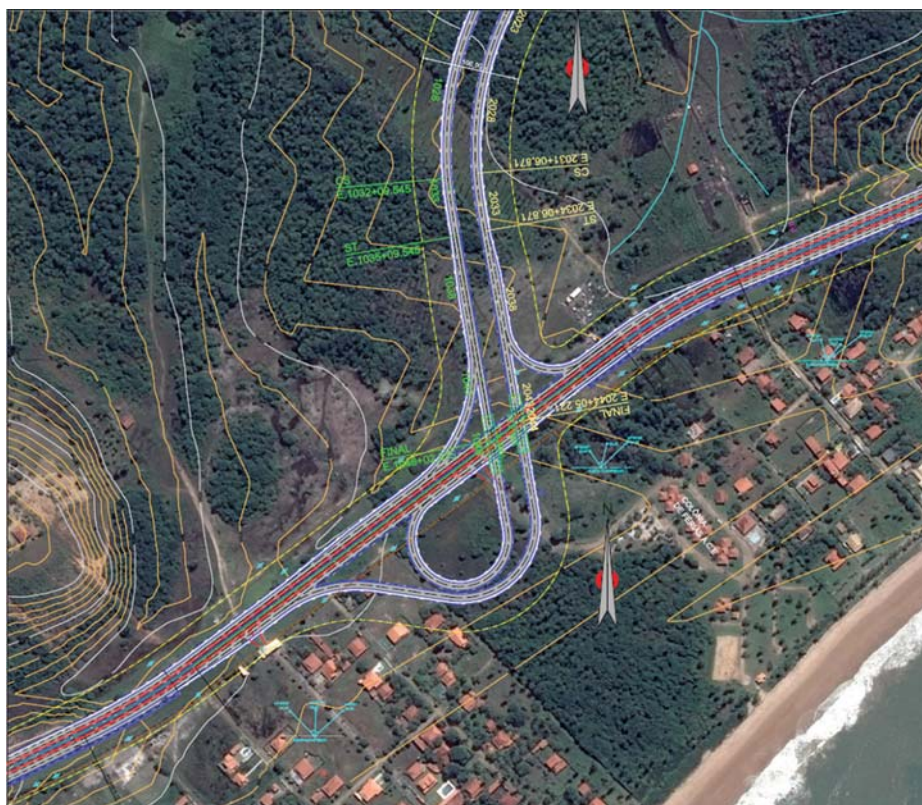
Planta da Interseção 3 (segmentos A/B/C)
