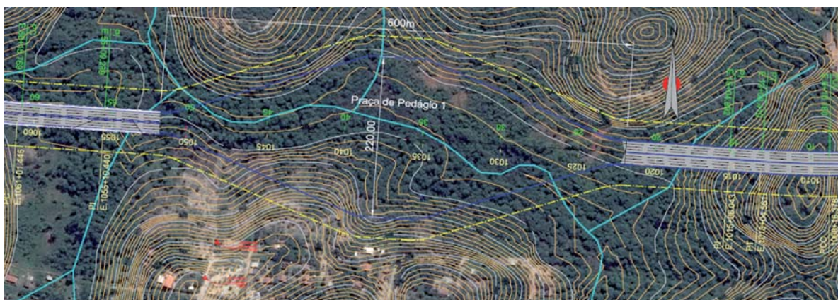
Fonte: Consórcio Enescil/COWI/Maia Melo Engenharia (2014b) Detalhe da Praça de pedágio 1 (segmento D)
