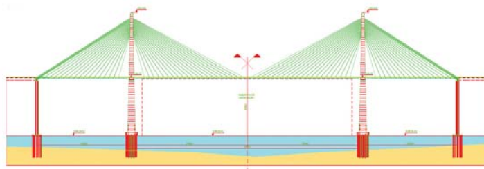
Perfil longitudinal do trecho estaiado da ponte Estacas dos apoios dos pilares ficarão submersas de forma permanente
