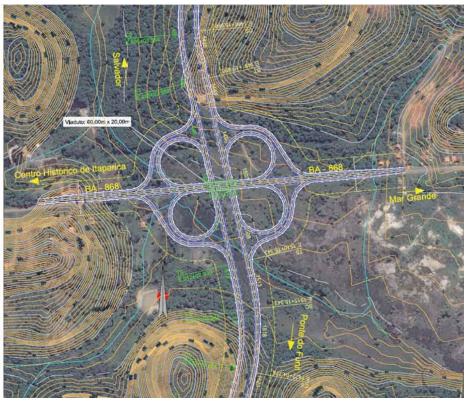
Planta da Interseção 2 (segmento B)
