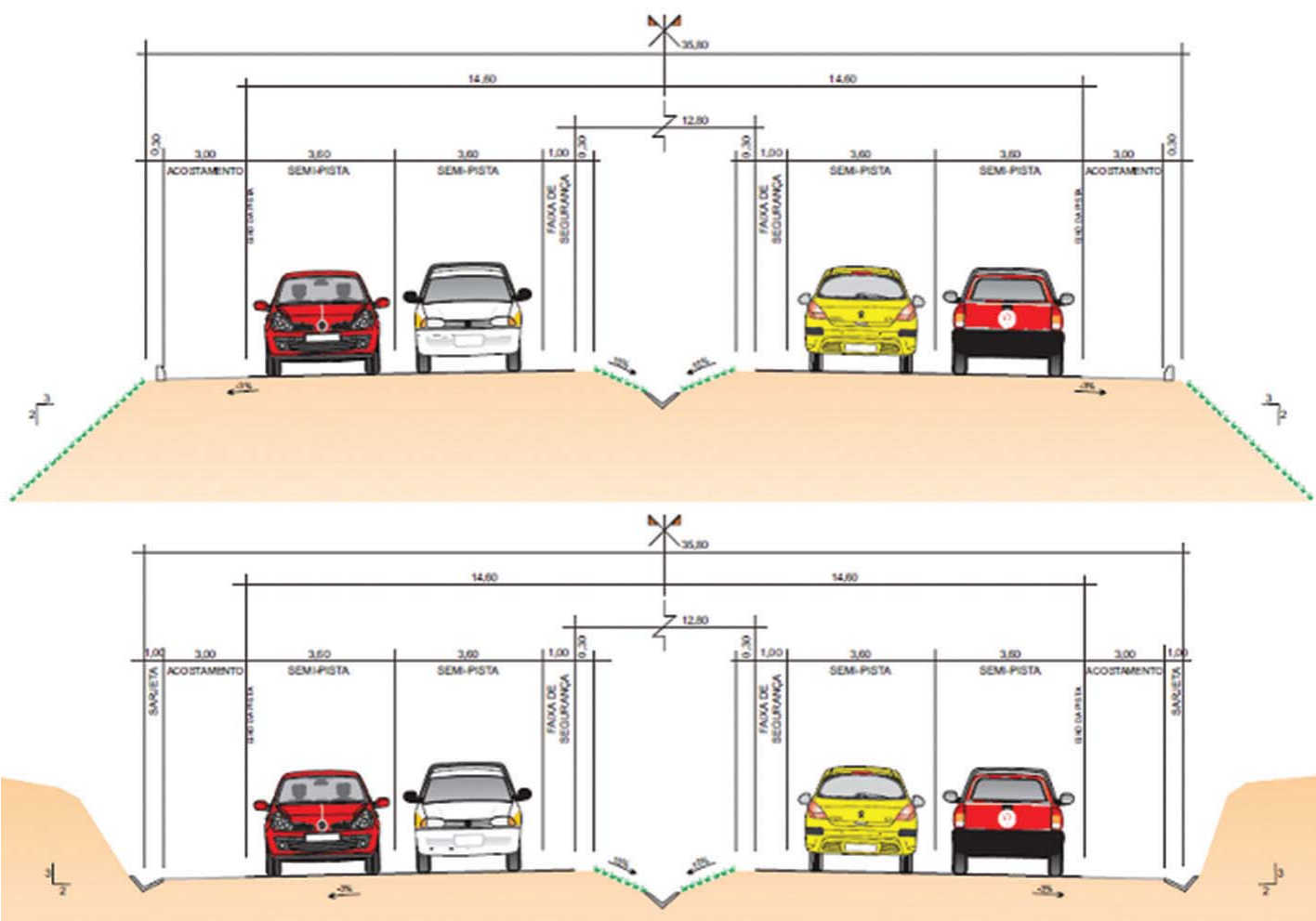
Seção transversal – Variante à BA-001
