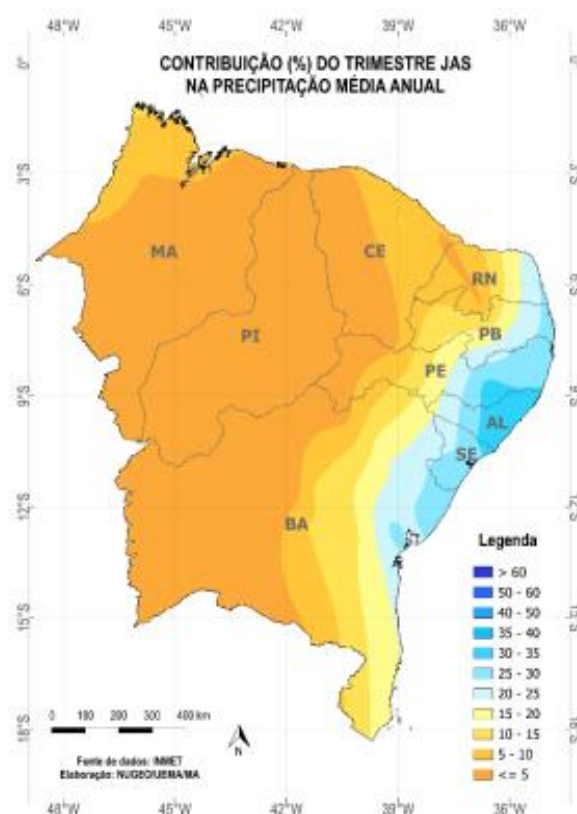
Figura 3 - Contribuição percentual do trimestre JAS na precipitação média anual para a Região Nordeste do Brasil. (Fonte: Climatologia INMET - 1991 a 2020).
