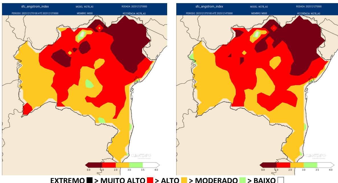
Figura 2 – Risco de fogo obtido pela umidade relativa e temperatura das 13 horas local. Cálculo: FRA = 0,06 \times UR\%13h - 0,1 \times (T13h - 27) Sempre que FRA < 2,5 é dado o alerta. Fonte de dados: Climatempo
