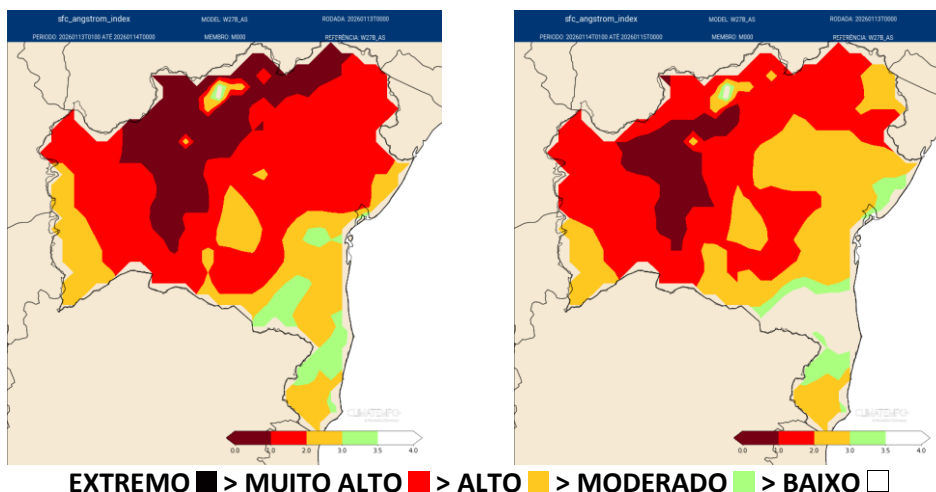
Figura 2 – Risco de fogo obtido pela umidade relativa e temperatura das 13 horas local.
