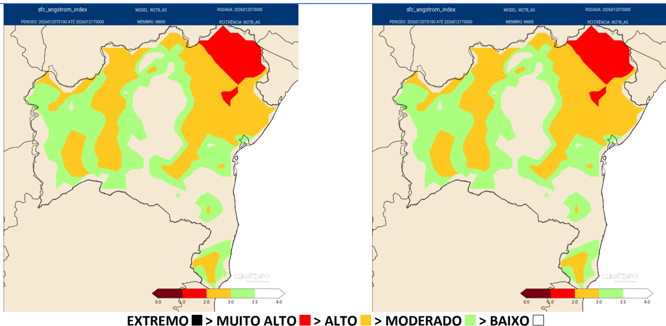
Figura 2 – Risco de fogo obtido pela umidade relativa e temperatura das 13 horas local. Cálculo: FRA = 0,06 \times UR\%13h - 0,1 \times (T13h - 27) Sempre que FRA < 2,5 é dado o alerta. Fonte de dados: Climatempo
