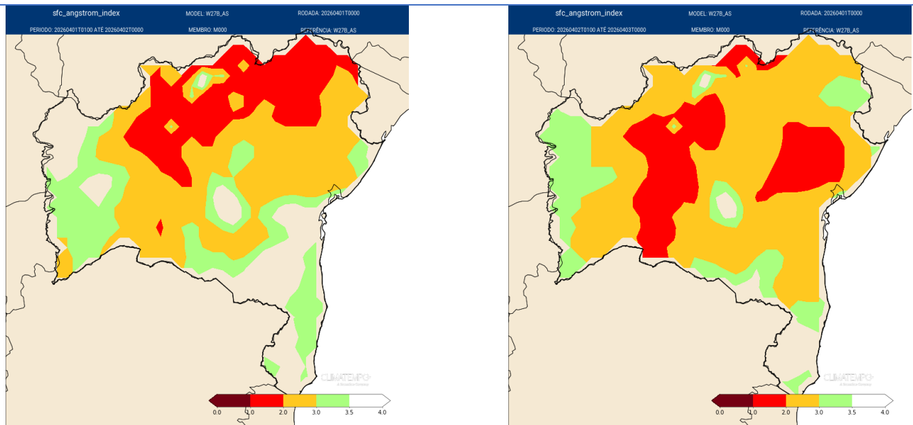
EXTREMO ■ > MUITO ALTO ■ > ALTO ■ > MODERADO ■ > BAIXO □ Figura 2 – Risco de fogo obtido pela umidade relativa e temperatura das 13 horas local. Cálculo: FRA = 0,06 x UR%13h – 0,1 x (T13h – 27) Sempre que FRA < 2,5 é dado o alerta. Fonte de dados: Climatempo.
