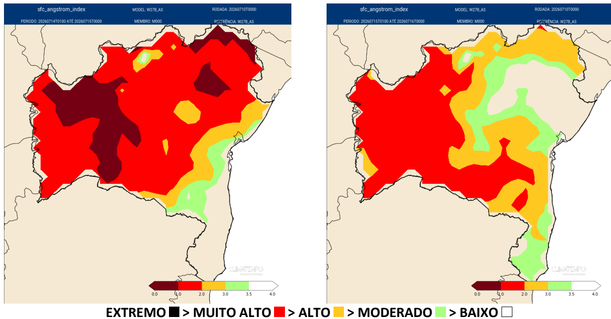
Figura 2 – Risco de fogo obtido pela umidade relativa e temperatura das 13 horas local. Cálculo: FRA = 0,06 \times UR_{13h} - 0,1 \times (T_{13h} - 27) Sempre que FRA < 2,5 é dado o alerta. Fonte de dados: Climatempo.
