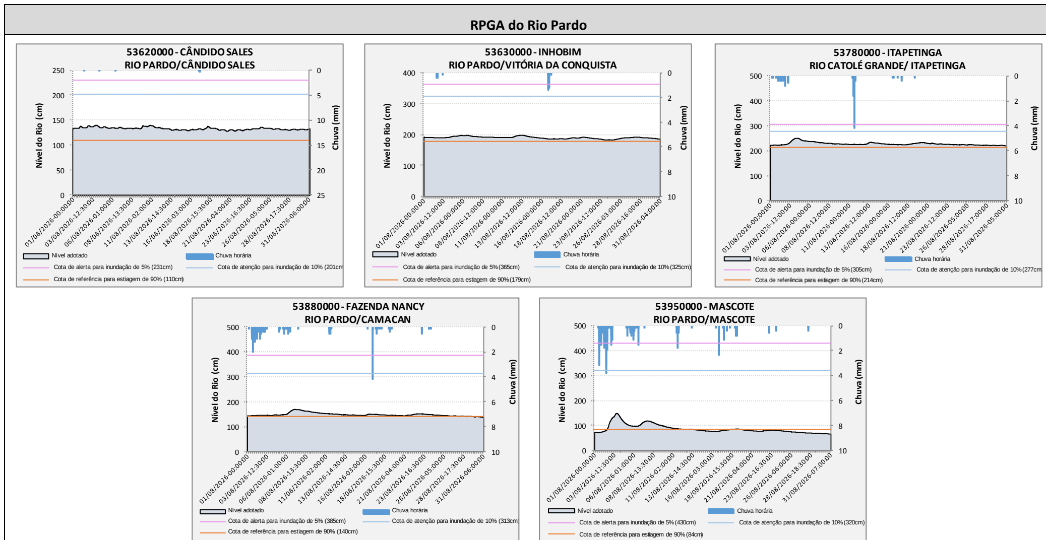
Figura 24 – Gráficos com o comportamento do nível dos rios na RPGA do Rio Pardo ao longo do mês de agosto de 2026
