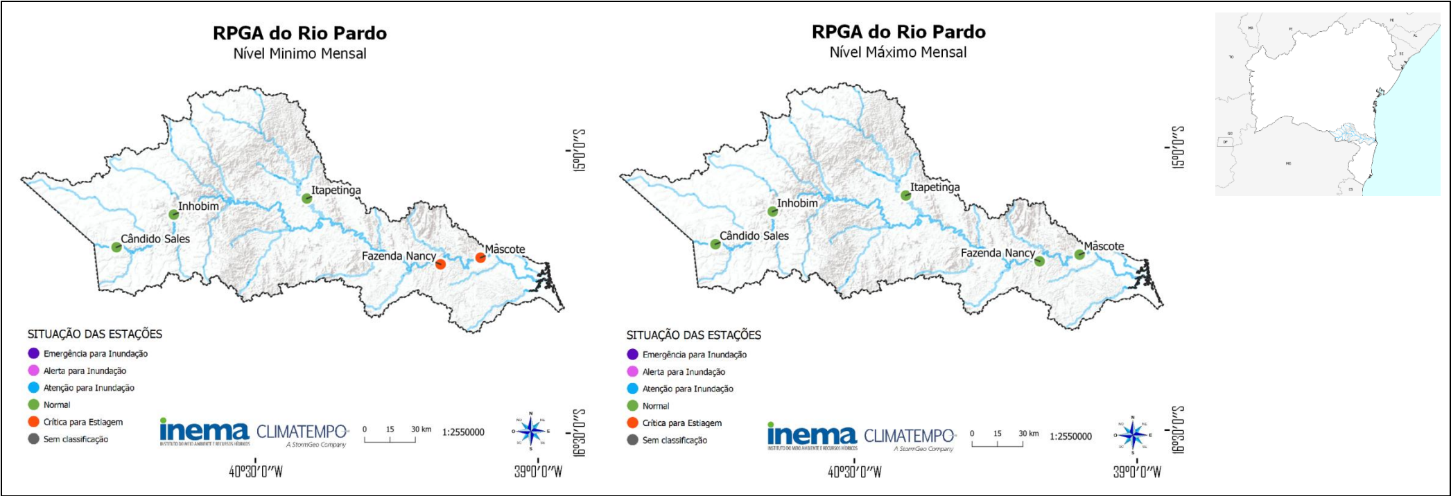
Figura 23 – Situação do nível dos rios na RPGA do Rio Pardo ao longo do mês de agosto de 2026
