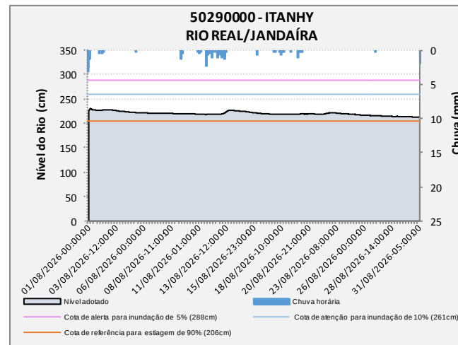
Figura 12 – Gráficos com o comportamento do nível dos rios na RPGA do Rio Real ao longo do mês de agosto de 2026.
