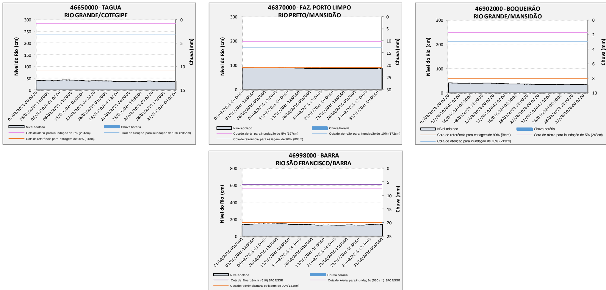
Figura 8 – Gráficos com o comportamento do nível dos rios na RPGA do Rio Grande ao longo do mês de agosto de 2026.
