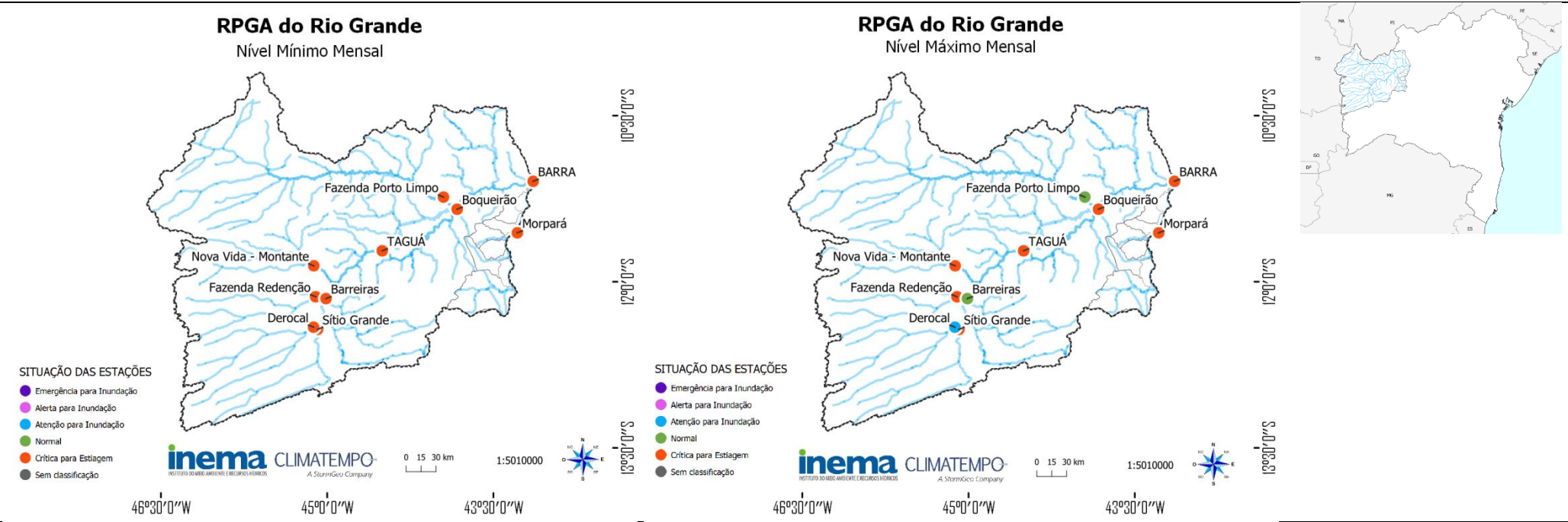
Figura 7 – Situação do nível dos rios na RPGA do Rio Grande ao longo do mês de agosto de 2026.
