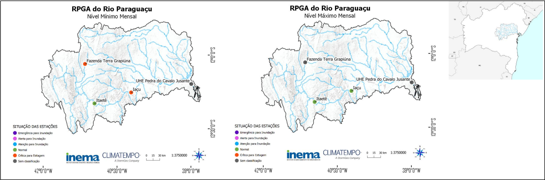
Figura 17 – Situação do nível dos rios na RPGA do Rio Paraguaçu ao longo do mês de agosto de 2026.
