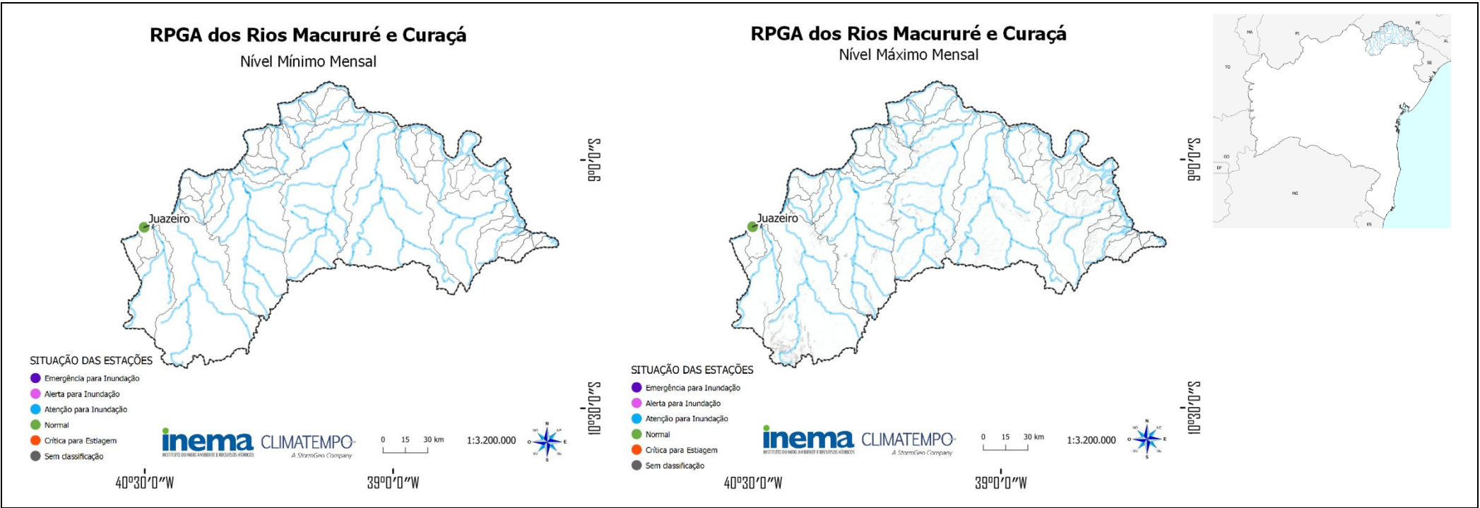
Figura 9 – Situação do nível dos rios na RPGA do Rios Macururé e Curaçá – Rio São Francisco ao longo do mês de agosto de 2026.
