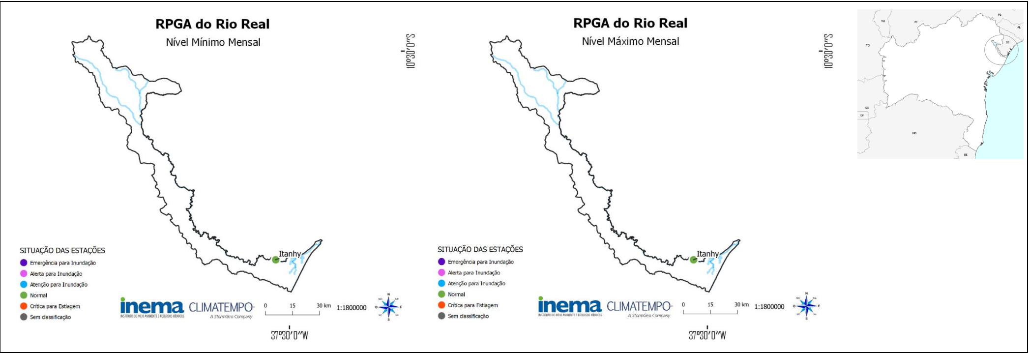
Figura 11 – Situação do nível dos rios na RPGA do Rio Real ao longo do mês de agosto de 2026.
