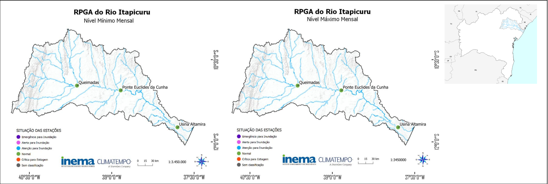
Figura 13 – Situação do nível dos rios na RPGA do Rio Itapicuru ao longo do mês de agosto de 2026.
