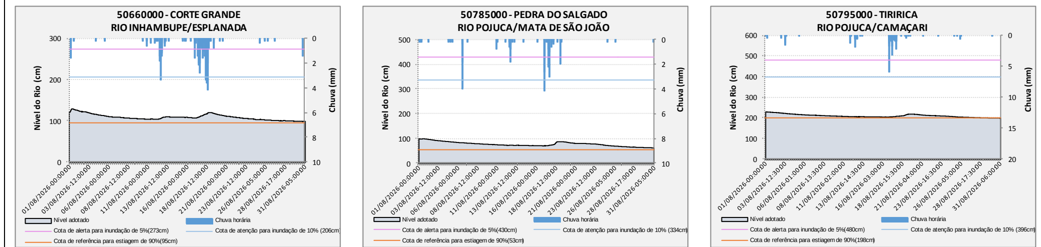
Figura 16 – Gráficos com o comportamento do nível dos rios na RPGA do Recôncavo Norte e Inhambupe ao longo do mês de agosto de 2026.
