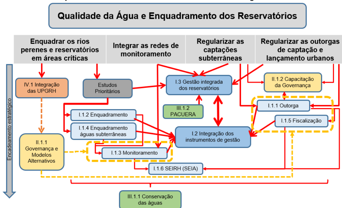
Figura 9.11 - Fluxograma da estratégia de regularização e monitoramento da Qualidade da Água e Enquadramento dos Reservatórios – Modelos alternativos de gestão
