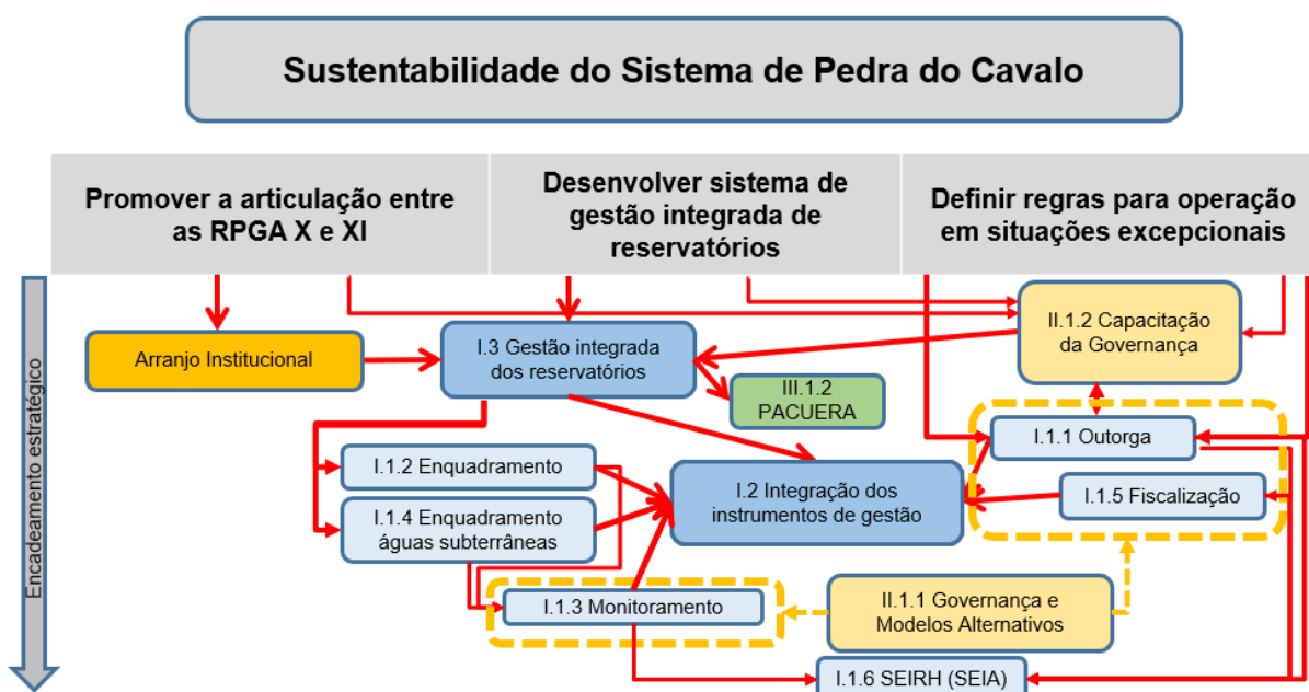
Figura 9.16 - Fluxograma da estratégia de Sustentabilidade do Sistema de Pedra do Cavalo – Modelos alternativos de gestão
