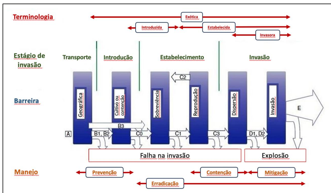
Figura 2 - Modelo conceitual unificado de invasões biológicas (adaptado de Blackburn et al. 2011).
