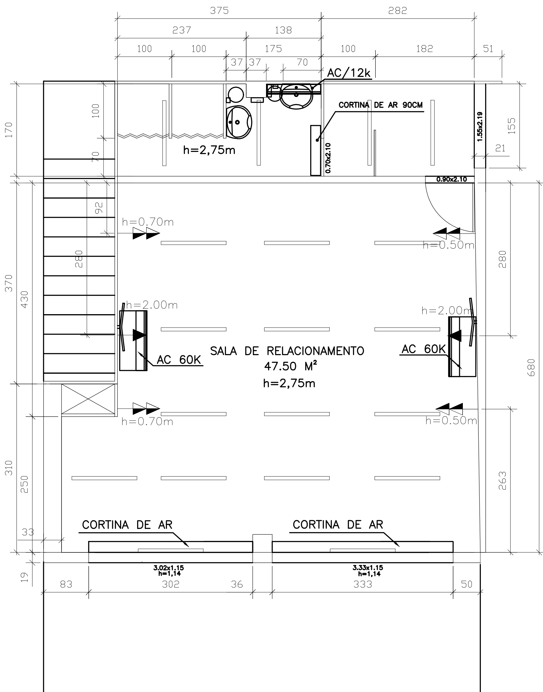
ESTÚDIO CAMPO GRANDE – 2º ANDAR PONTOS DE LUZ E TOMADAS
