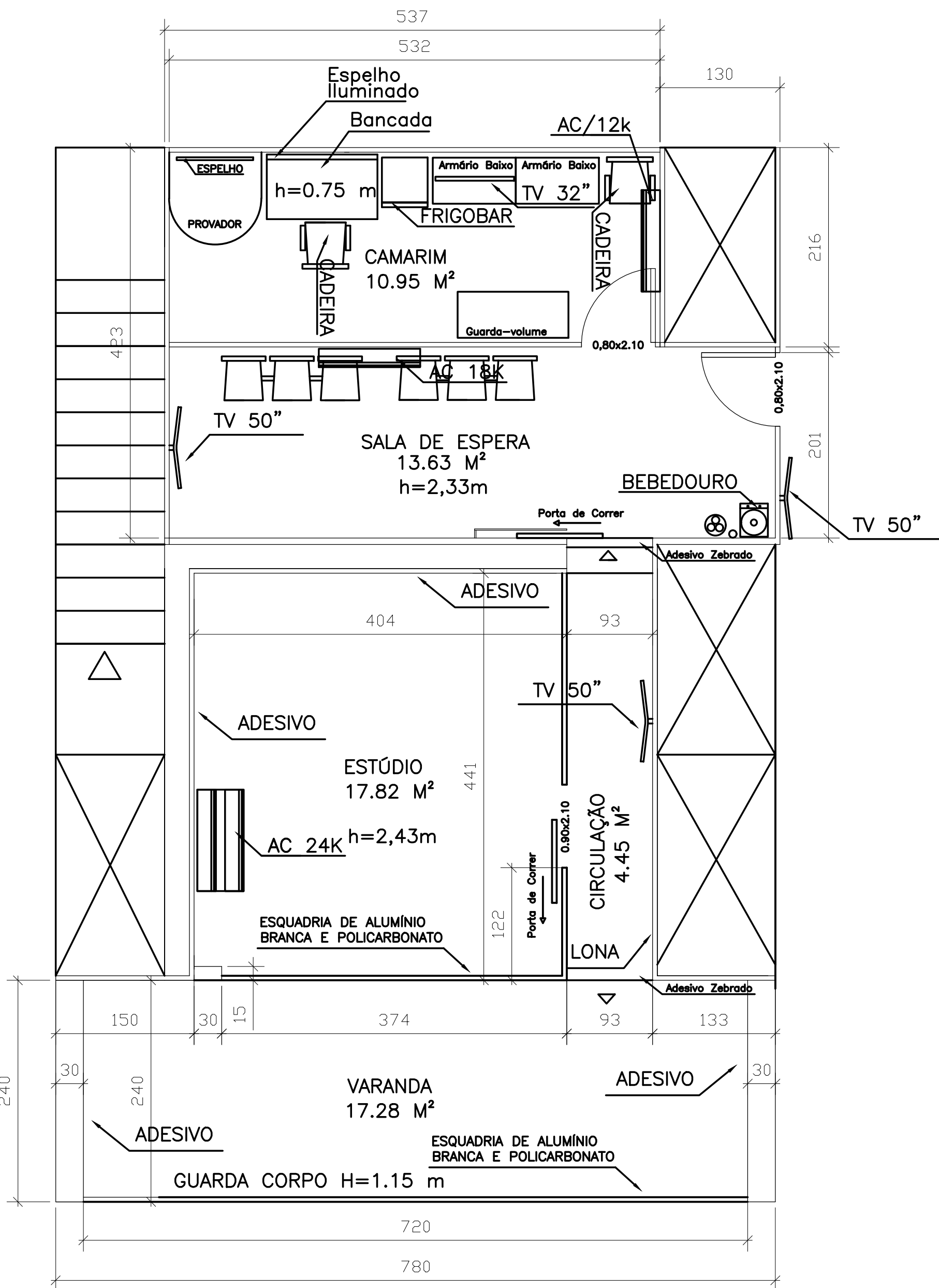
ESTÚDIO CAMPO GRANDE – 1º ANDAR
