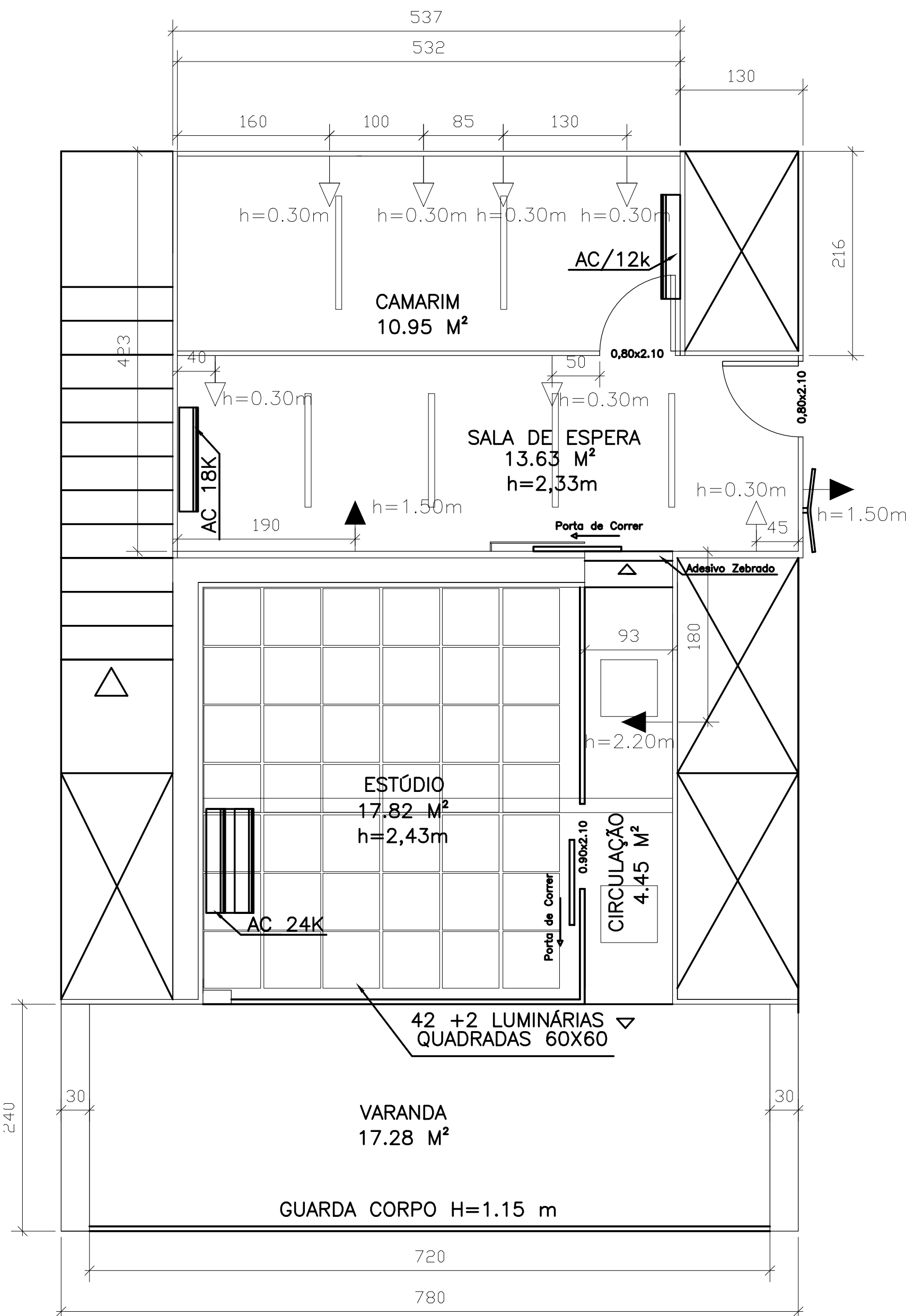
ESTÚDIO CAMPO GRANDE – 1º ANDAR PONTOS DE LUZ E TOMADAS
