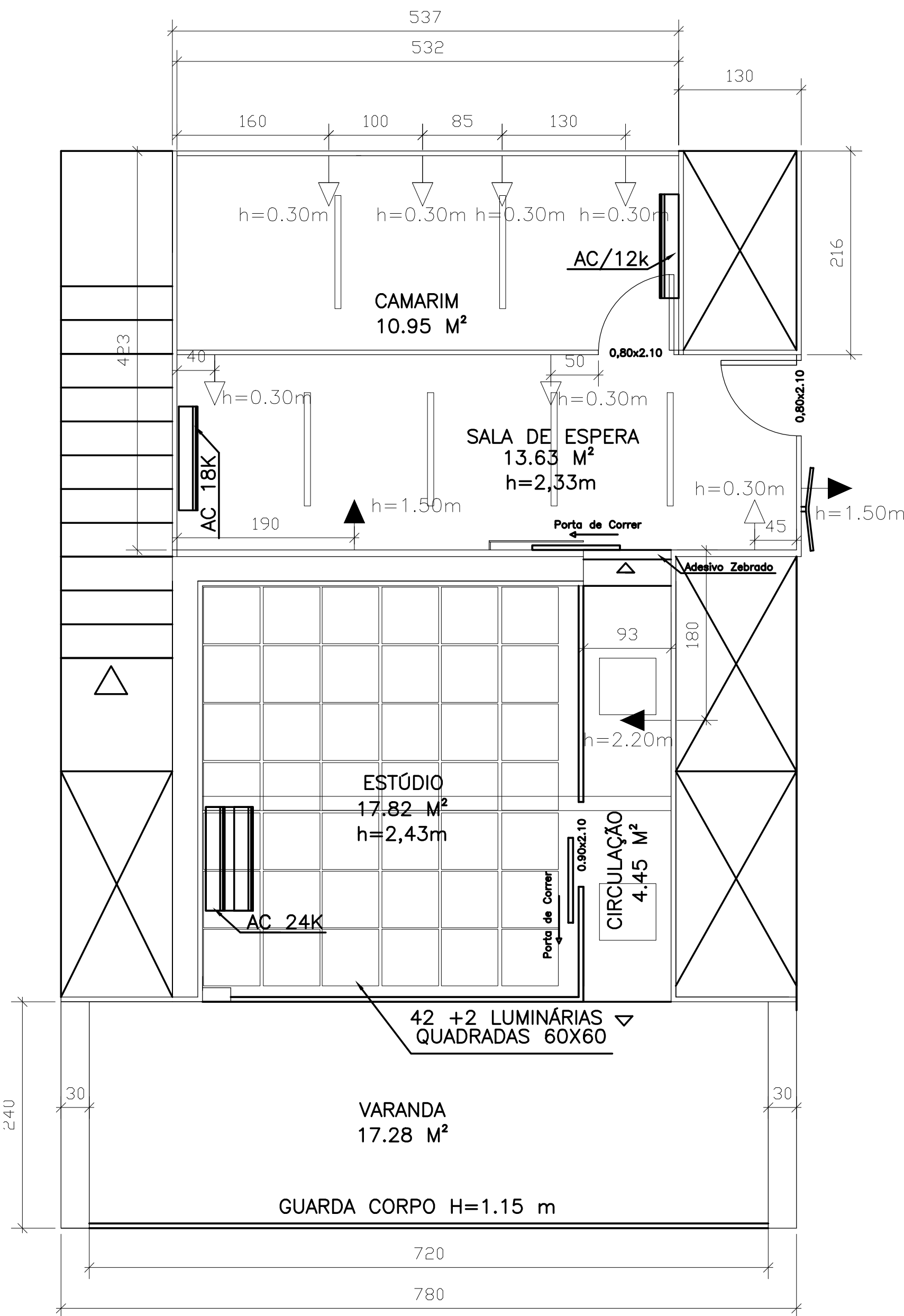
ESTÚDIO CAMPO GRANDE – 1º ANDAR PONTOS DE LUZ E TOMADAS
