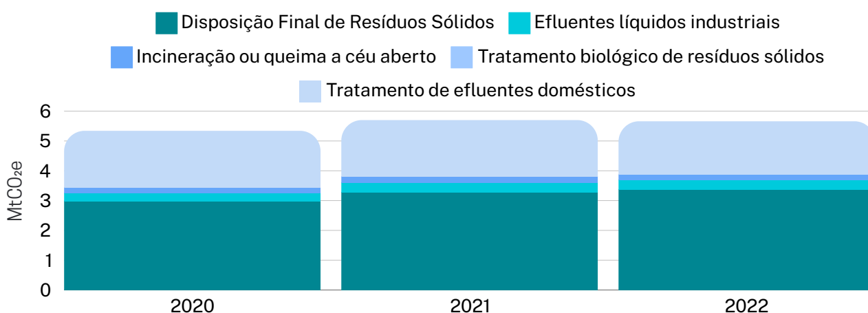
Figura 16. Emissões de GEE por categoria emissora do setor Resíduos (ano referência 2020-2022).
