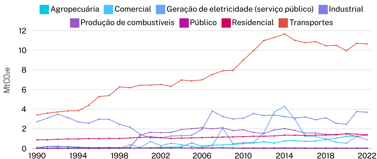
Figura 28. Emissões de GEE pela Queima de Combustíveis no Setor Energia (ano referência 1990-2022).
