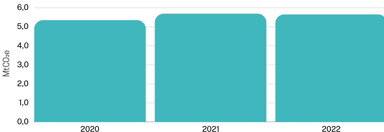
Figura 15. Emissões de GEE do setor Resíduos (ano referência 2020-2022).
