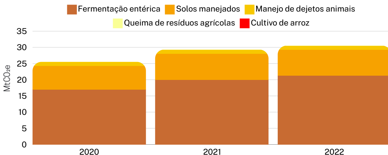
Figura 32. Emissões de GEE por categoria emissora do setor Agropecuária (ano referência 2020-2022).
