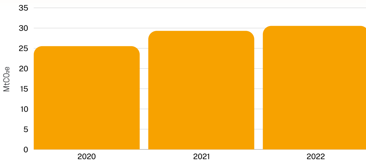
Figura 31. Emissões de GEE do setor Agropecuária (ano referência 2020-2022).
