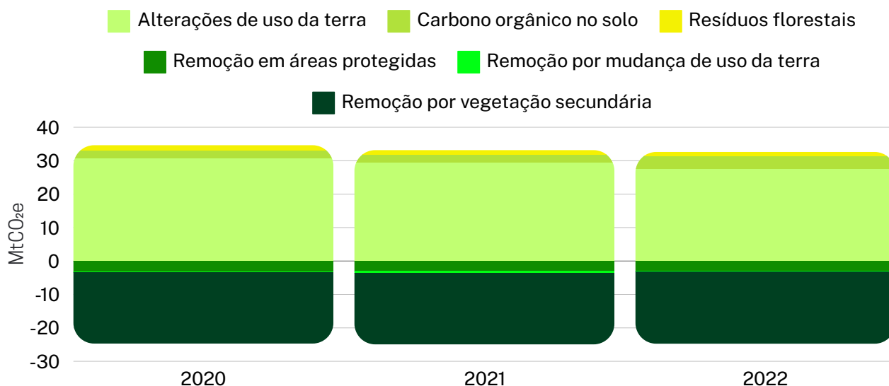
Figura 38. Emissões e remoções de GEE por categoria do setor Mudanças de Uso da Terra e Floresta (ano referência 2020-2022).
