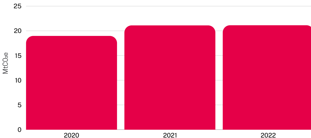
Figura 22. Emissões de GEE do setor Energia (ano referência 2020-2022).
