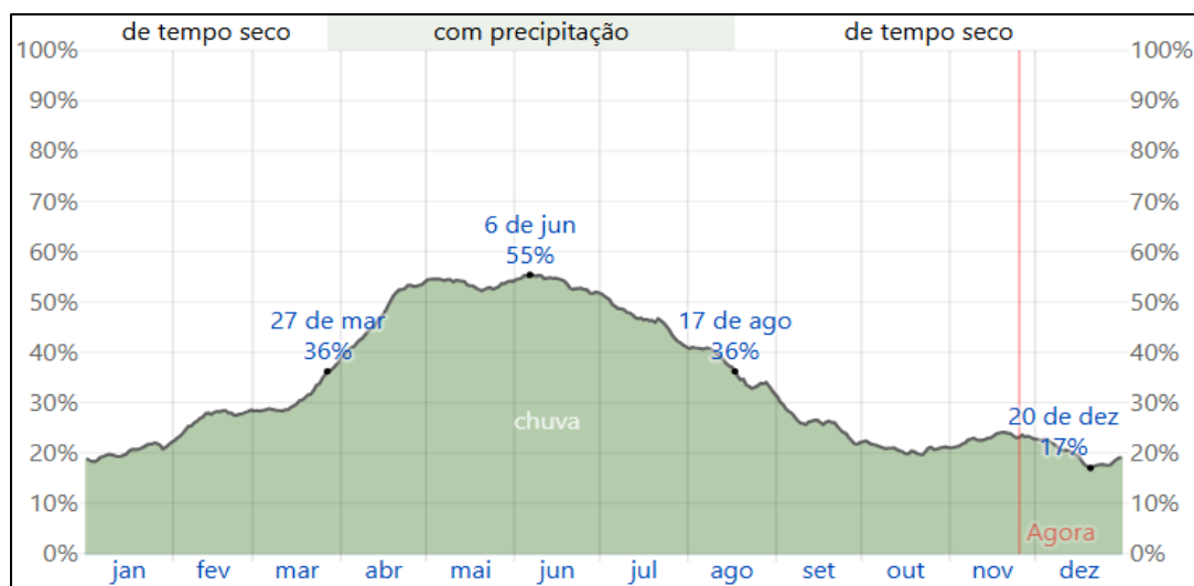
Figura 12 – Probabilidade de Precipitação em Abril em Camaçari. Fonte: weatherspark.
