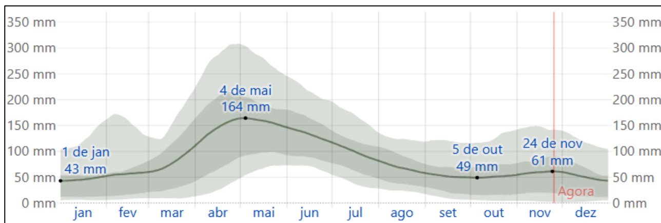
Figura 9 – Precipitação média(linha contínua) acumulada em Camaçari
