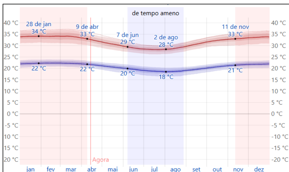
Figura 11 – Temperaturas máxima, mínima, média em Camaçari. Fonte: weatherspark.
