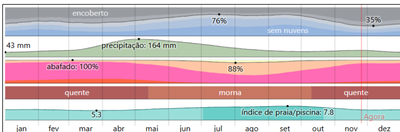
Figura 10 – Clima em Camaçari. Fonte: weatherspark.
