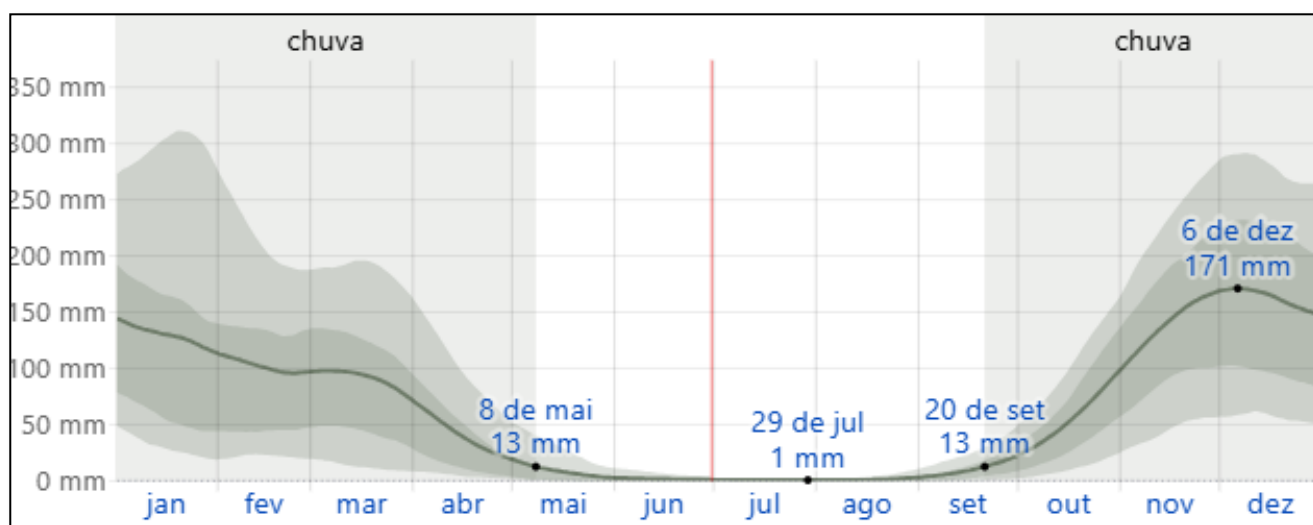
Figura 8 – Precipitação média(linha continua) acumulada. Fonte: Weatherspark.
