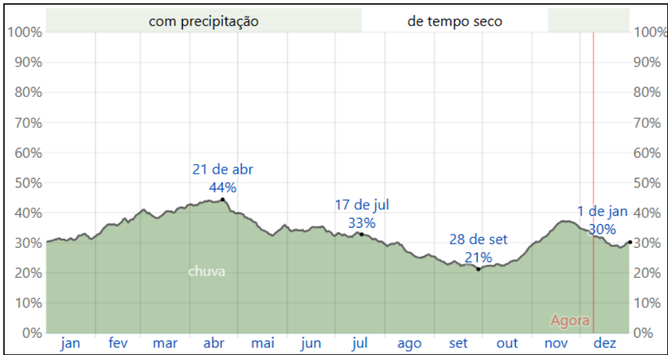
Figura 8 – Probabilidade de Precipitação em Jequié. FONTE: WEATHERSPARK.
