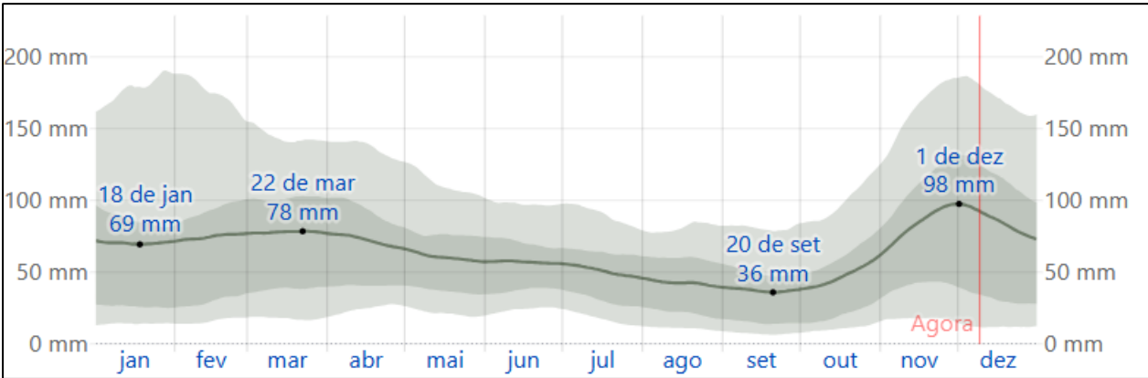
Figura 5 – Precipitação média(linha contínua) acumulada em Jequié
