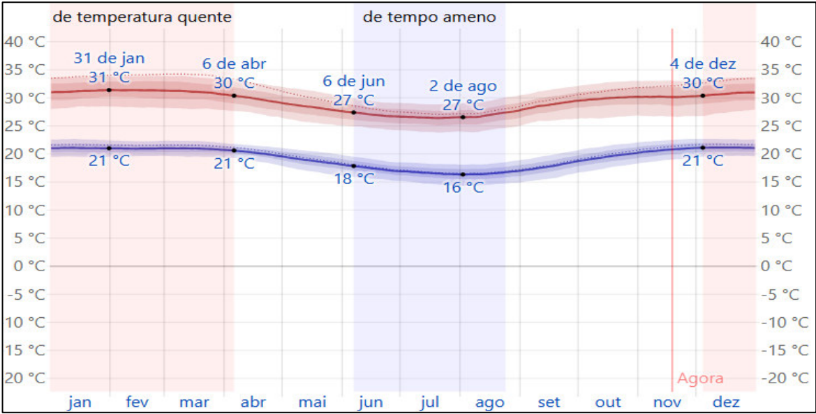
Figura 9 – Temperaturas máxima, mínima, média em Pau Brasil. FONTE: WEATHERSPARK.
