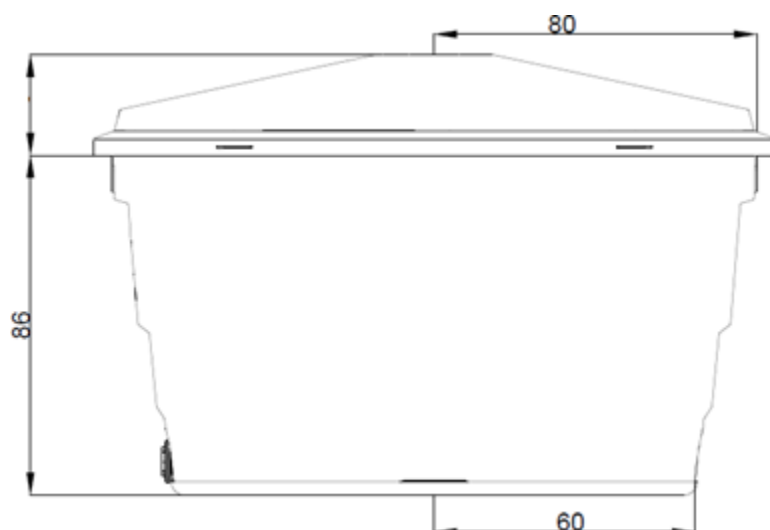
Fig. 1: Dimensões da caixa d'água de 1000 L (imagem meramente ilustrativa)
