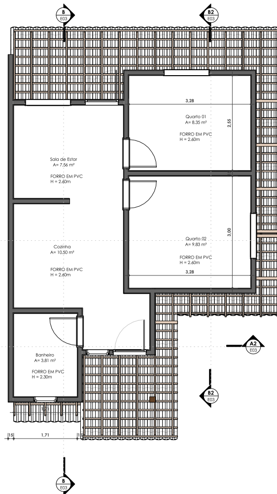
Térreo - Planta de forro ESC: 1 : 50
