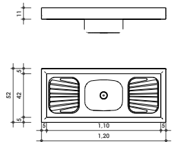
Detalhamento Pia Cozinha ESC: 1 : 25
