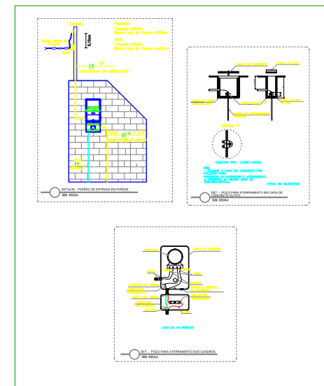
DETALHES PADRÃO DE ENTRADA
