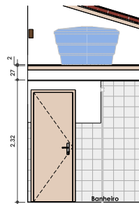
Sanit. Elev. C ESC: 1 : 50
