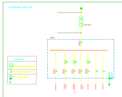
DETALHES QUADRO DE DISTRIBUIÇÃO GERAL
