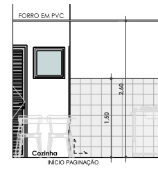
Cozinha e Sala Elev. D ESC: 1 : 50
