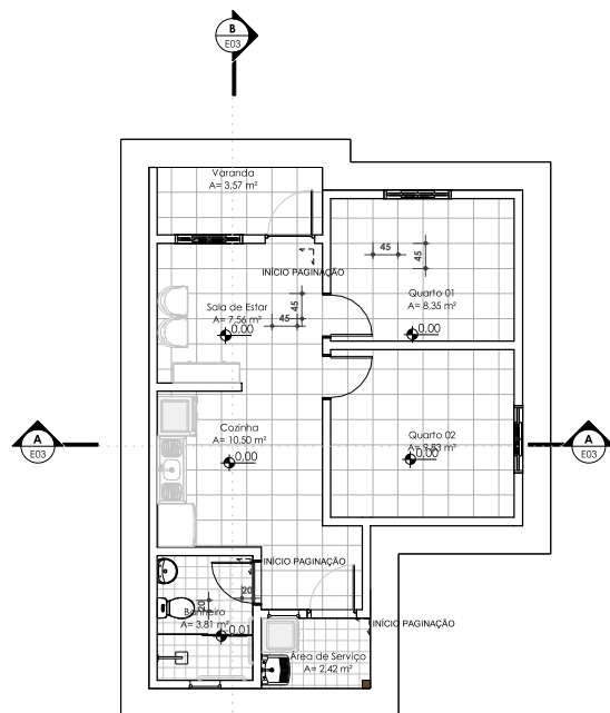
Térreo - Planta de Piso ESC: 1 : 75
