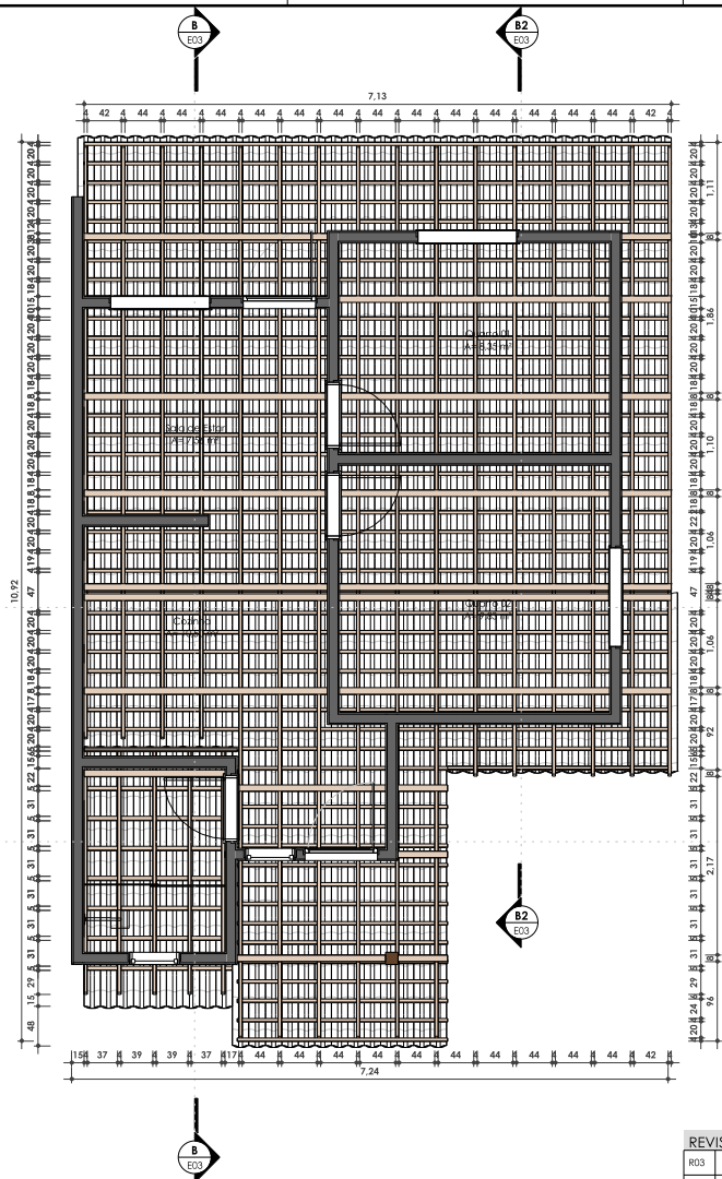
Térreo - Madeiramento ESC: 1 : 50
