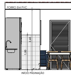
Cozinha e Sala Elev. B ESC: 1 : 50
