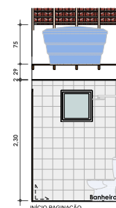
Sanit. Elev. D ESC: 1 : 50
