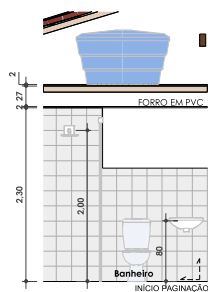
Sanit. Elev. A ESC: 1 : 50
