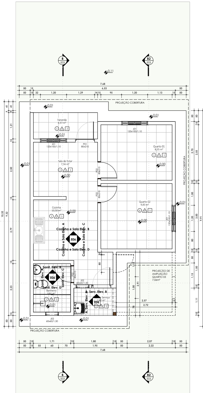
Térreo - Executivo ESC: 1 : 50
