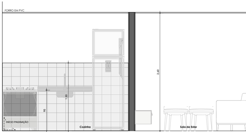
Cozinha e Sala Elev. A ESC: 1 : 25
