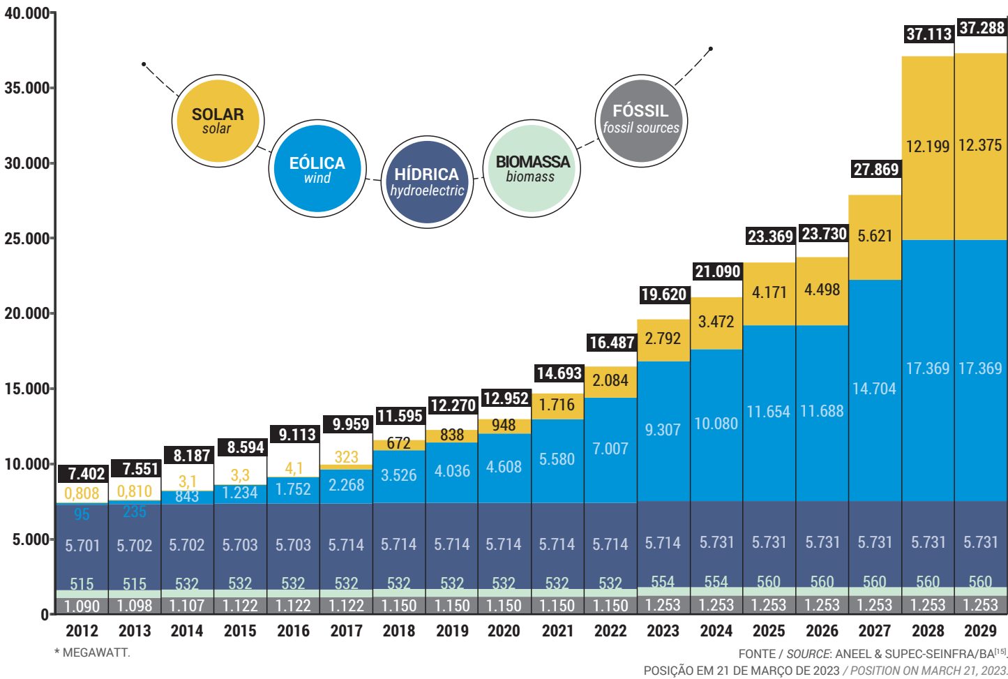
GRÁFICO 1.3 Bahia: Evolução da capacidade instalada por fonte em MW*. CHART 1.3 Bahia: Evolution of installed capacity by source in MW*.
