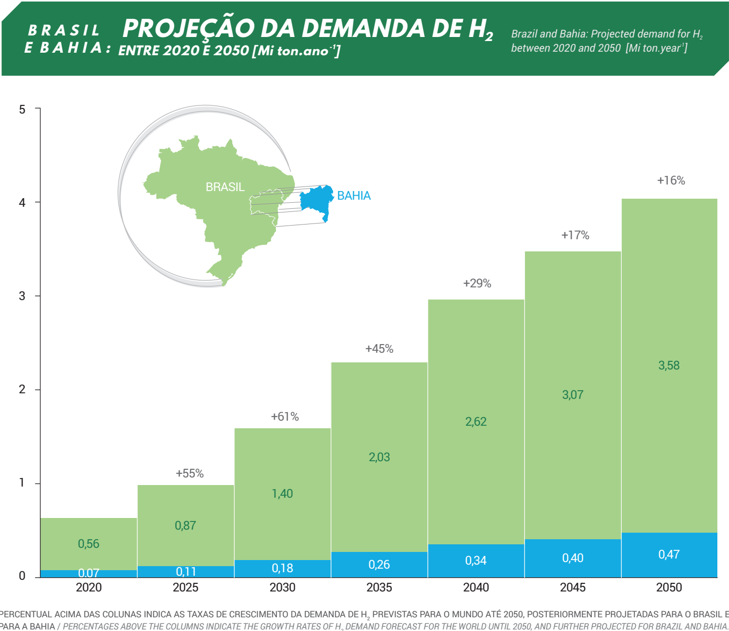
GRÁFICO 7.4 Brasil e Bahia: Projeção da demanda de H 2 entre 2020 e 2050. CHART 7.4 Brazil and Bahia: Projected demand for H 2 between 2020 and 2050.
