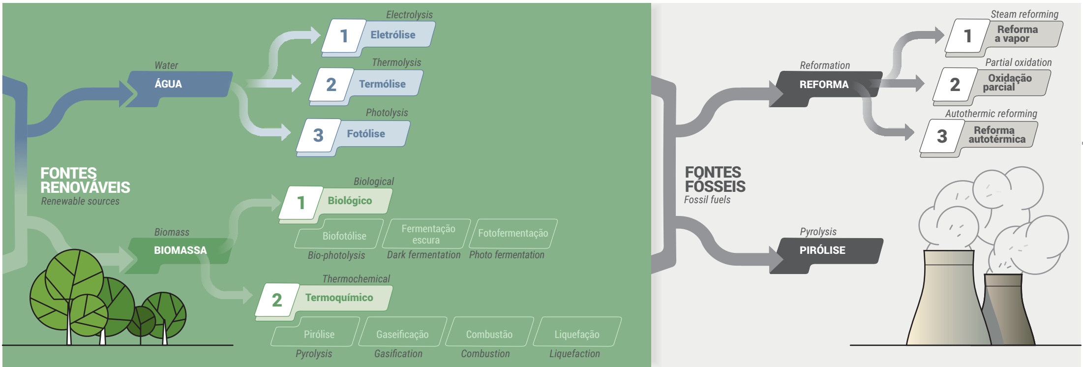
FIGURA 2.7 Rotas tecnológicas de produção de H_2 a partir de fontes fósseis e renováveis. FIGURE 2.7 Technological routes to H_2 production from fossil and renewable sources.
