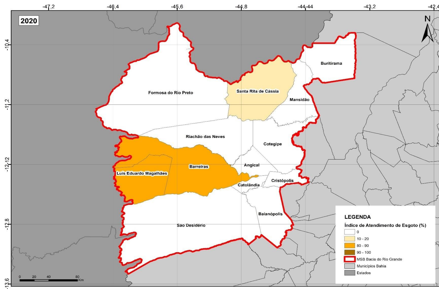
Figura 13 – Cenarização do índice de atendimento por esgotamento sanitário da MSB/BRG – Situação atual (2020)
