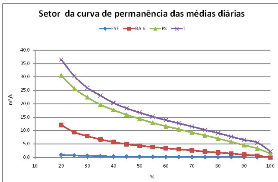
Figura 4.42 - Curvas de permanência das vazões médias diárias para as estações (20% a 100%)
