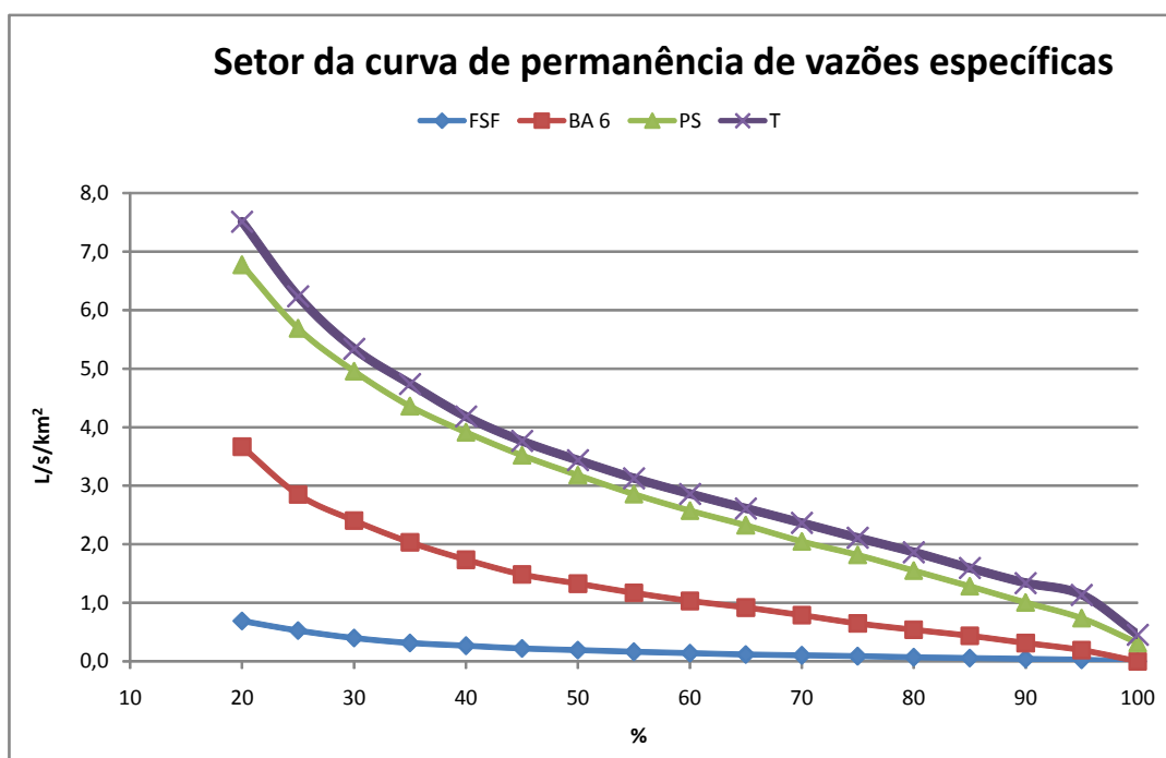
Figura 4.46 - Curvas de permanência das vazões específicas para as estações (20% a 100%)
