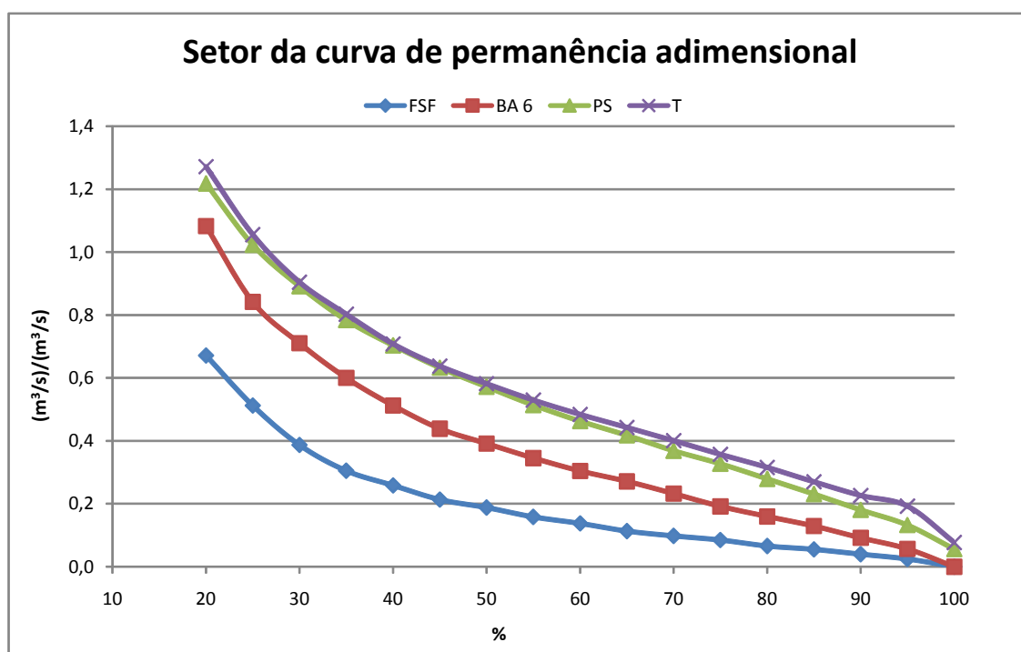
Figura 4.44 - Curvas de permanência adimensionais para as estações (20% a 100%)
