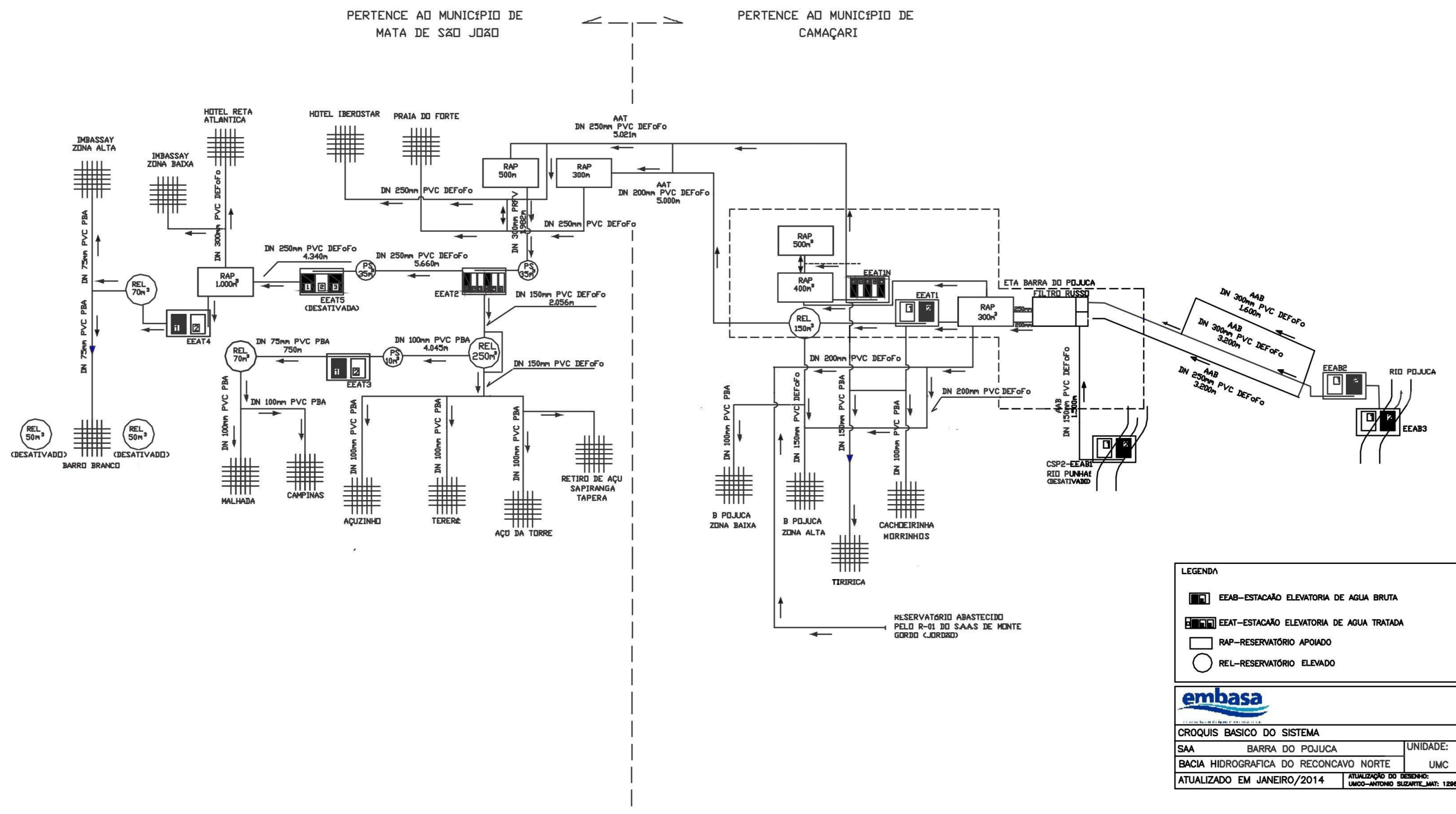
Figura 4.27 – Croqui esquemático do SIAA de Barra do Pojuca Fonte: Adaptado de EMBASA, 2014.
