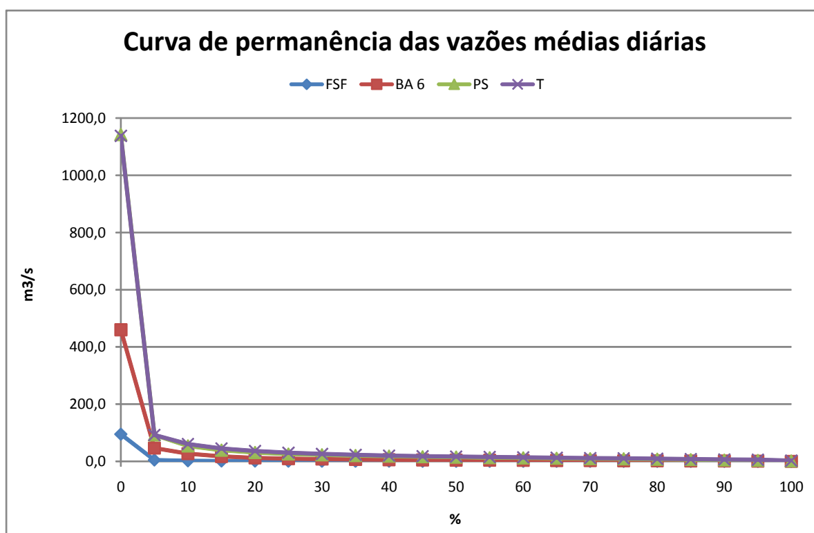
Figura 4.41 - Curvas de permanência das vazões médias diárias para as estações (0 a 100%)
