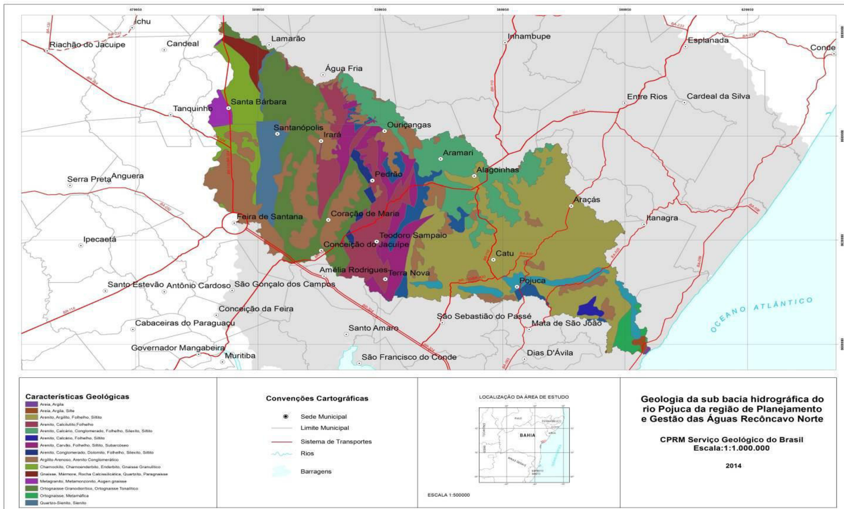
Figura 4.49 – Características geológicas da sub-bacia do rio Pojuca
