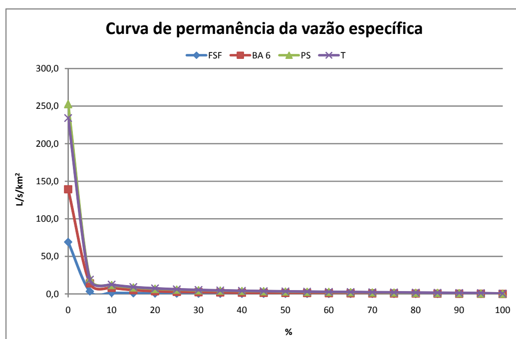
Figura 4.45 - Curvas de permanência da vazões específicas para as estações (0 a 100%)
