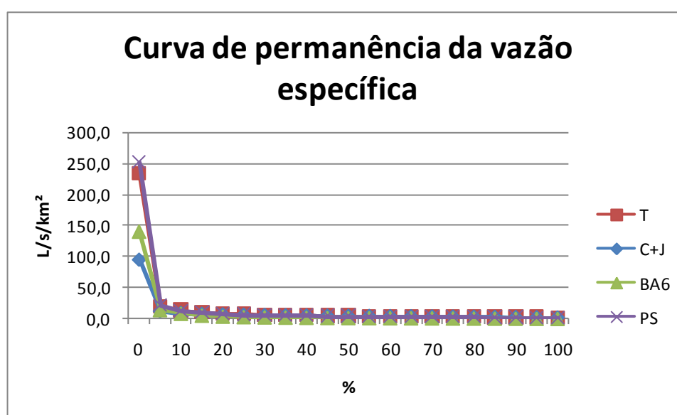
Figura 4.80 - Curva de permanência da vazão específica
