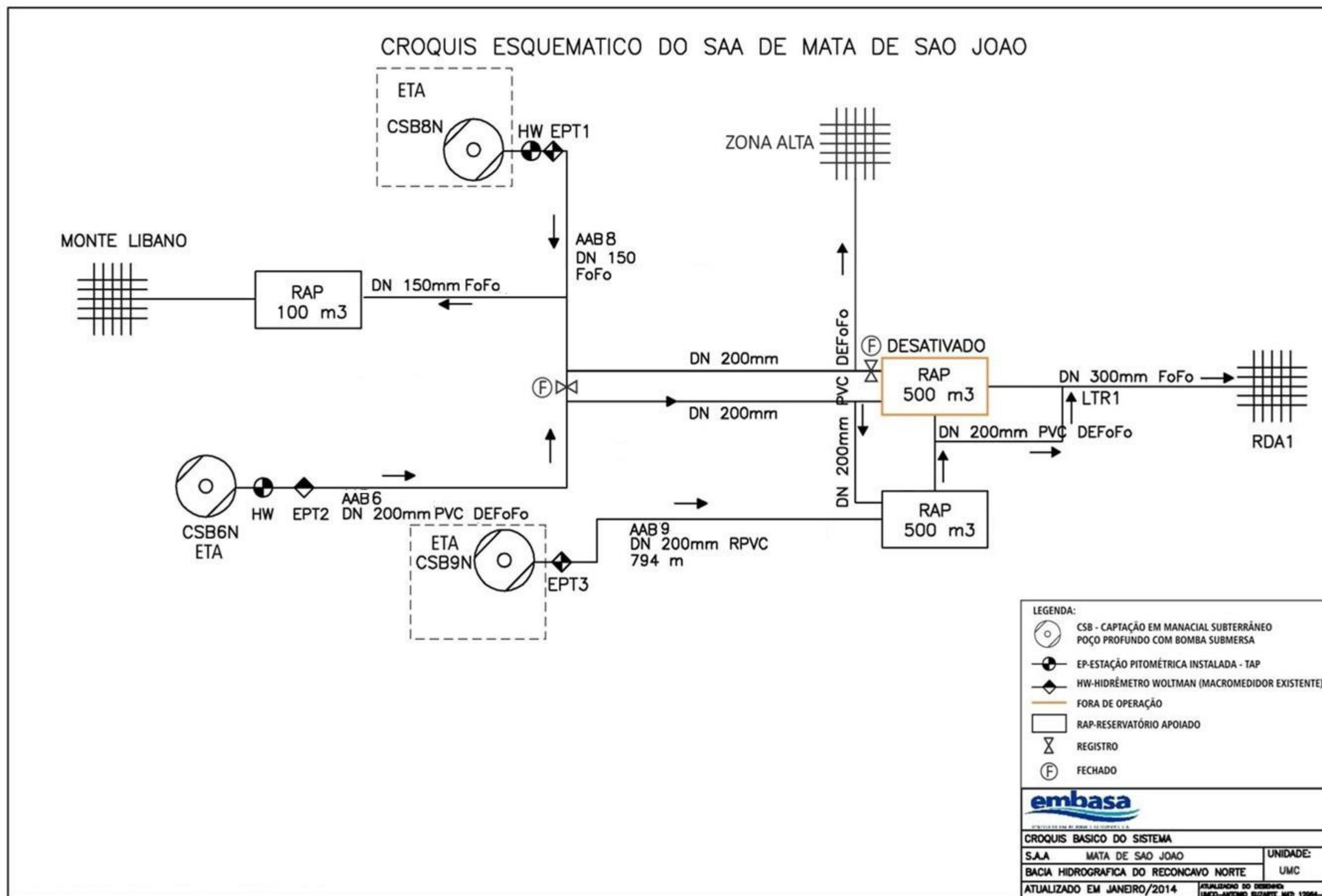
Figura 4.1 - Croqui esquemático do SAA de Mata de São João
