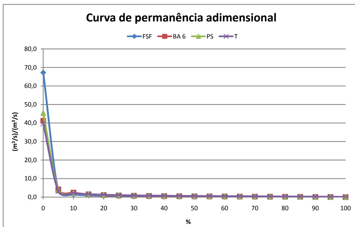
Figura 4.43 - Curvas de permanência adimensionais para as estações (0 a 100%)
