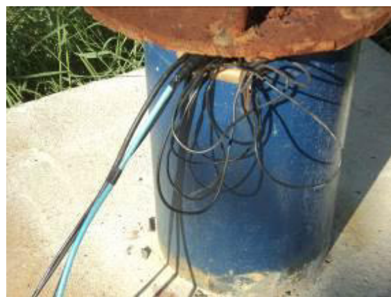
Figura 4.121 - Poço CSB2 – Instalações elétricas expostas
