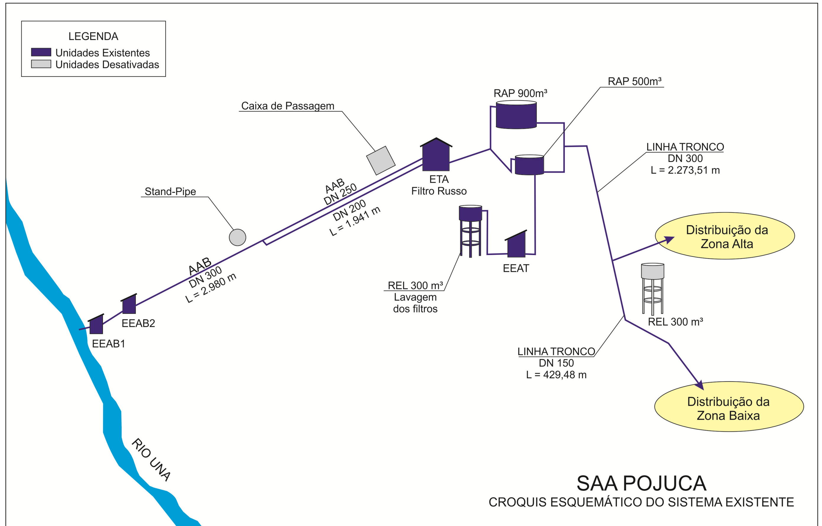
Figura 5.1 – Croqui esquemático do SAA de Pojuca
