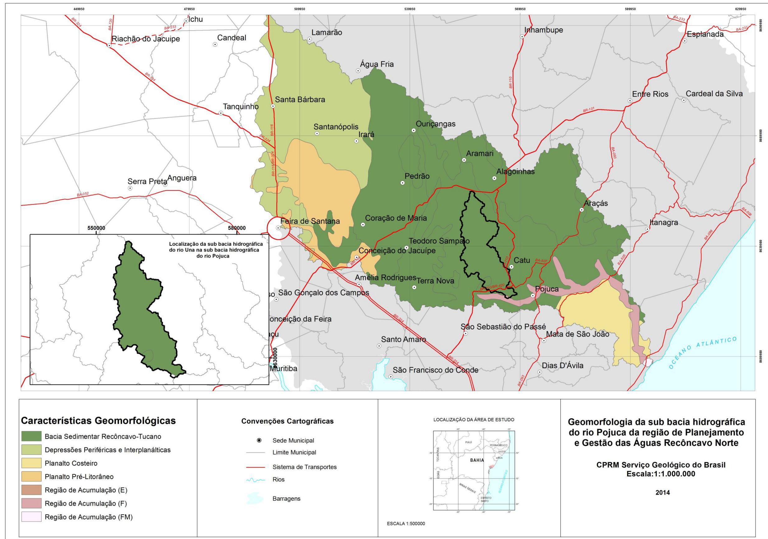
Figura 5.24 – Características geomorfológicas da sub-bacia do rio Pojuca, com destaque à área de drenagem do rio Una
