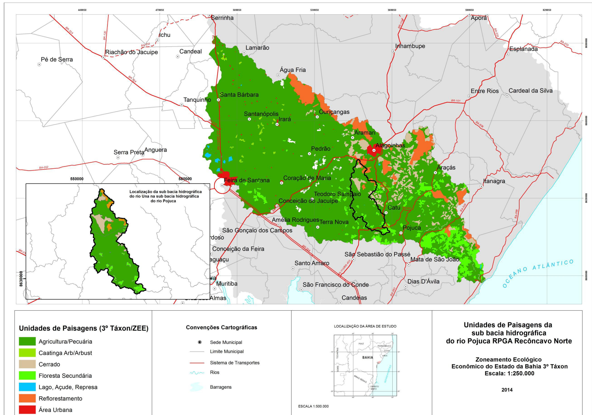
Figura 5.38 – Unidades de paisagem da sub-bacia hidrográfica do rio Pojuca, com destaque à área de drenagem do rio Una
