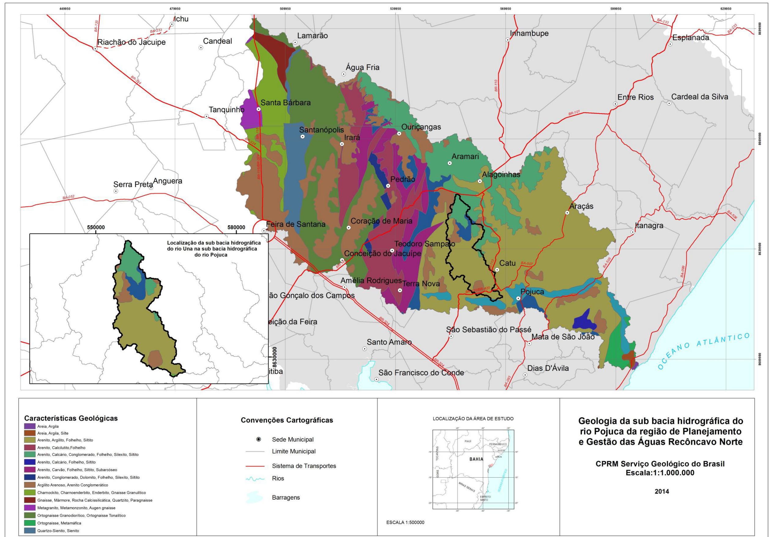
Figura 5.23– Características geológicas da sub-bacia do rio Pojuca, com destaque à área de drenagem do rio Una
