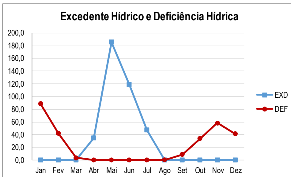
Figura 5.12 - Excedente e deficiência hídrica em Açu da Torre (em mm)
