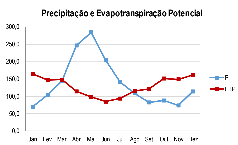
Figura 5.11 - Precipitação e evapotranspiração potencial em Açu da Torre (em mm)
