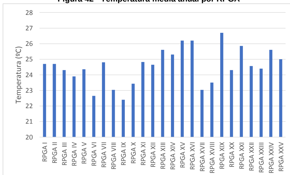
Figura 42 - Temperatura média anual por RPGA
