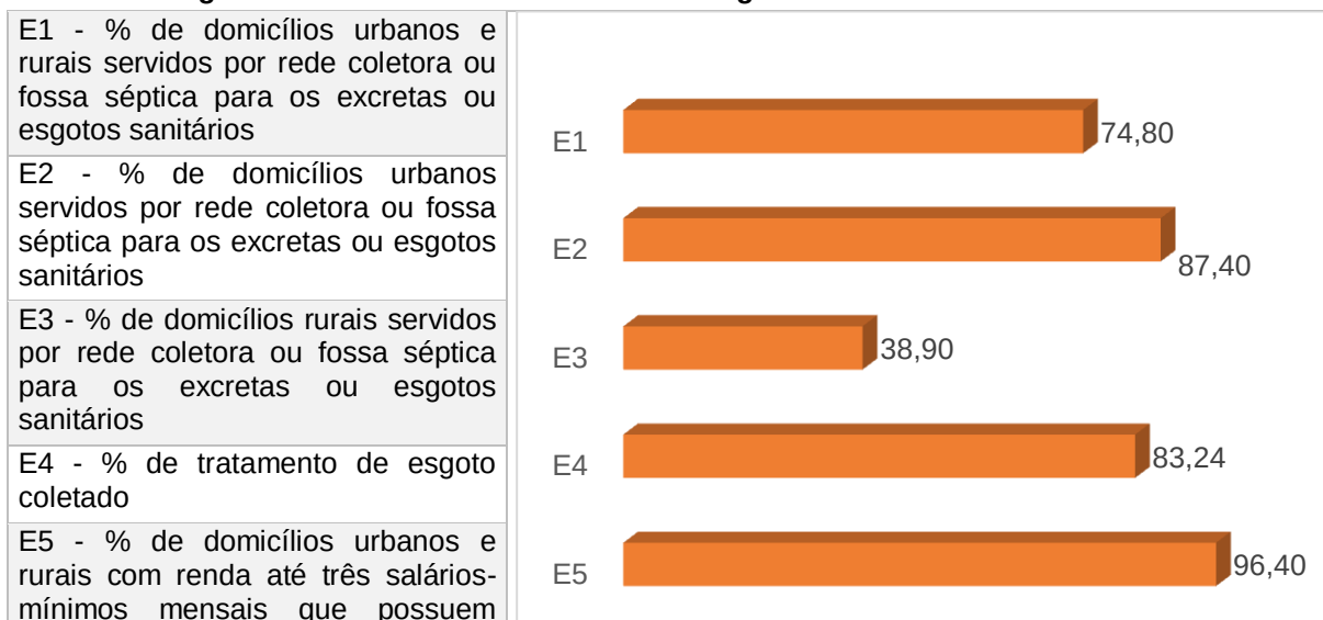
Figura 4 – Gráfico dos indicadores de esgotamento sanitário - PESB/BA
