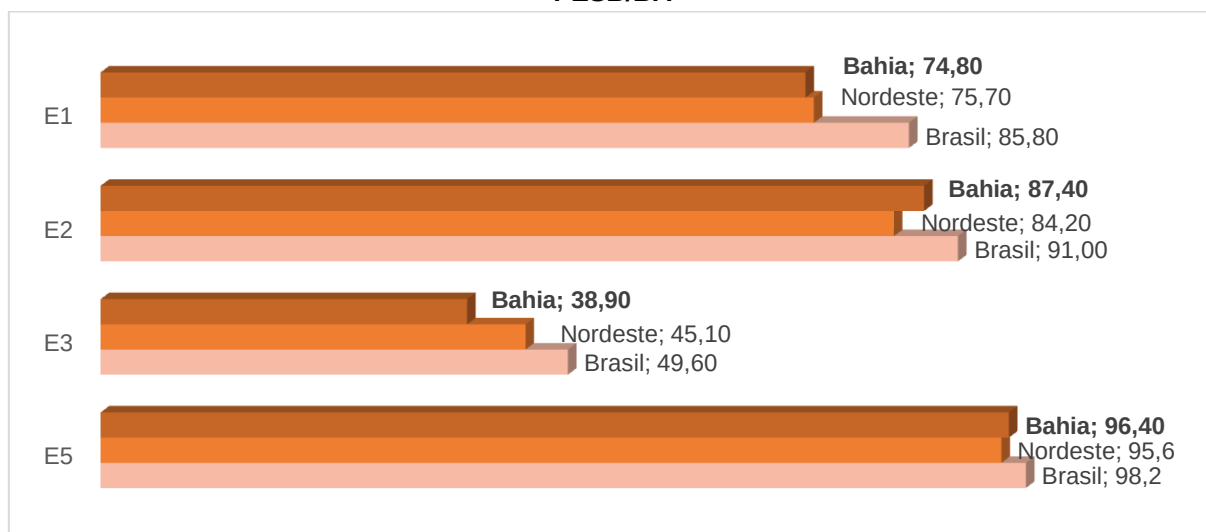
Figura 5 – Gráfico comparativo dos indicadores E1, E2, E3 e E5 entre Bahia, Nordeste e Brasil - PESB/BA
