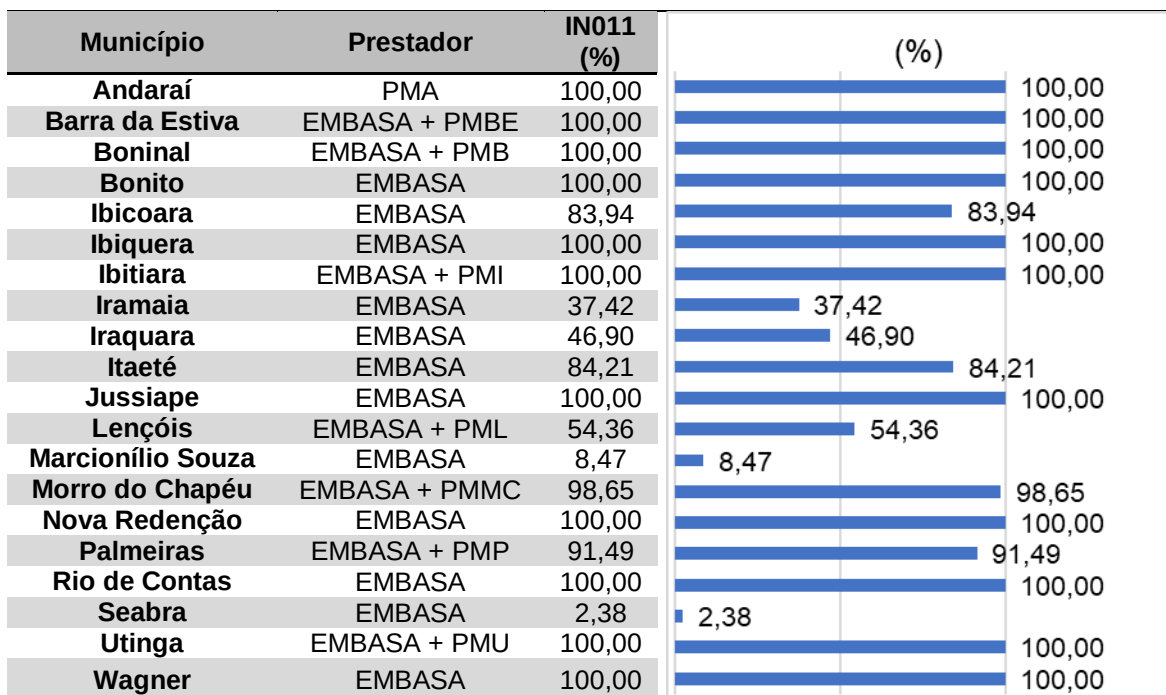
Figura 37 - Índice de Macromedicação (IN011) na MSB da Chapada Diamantina
