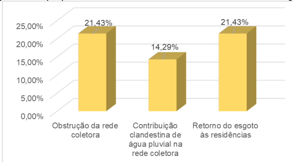
Figura 80 – Principais problemas observados nas redes coletoras da MSB do Piemonte do Paraguaçu
