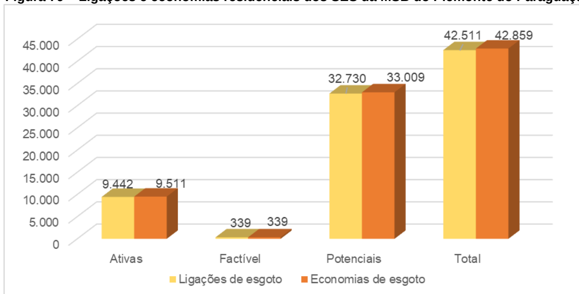
Figura 79 – Ligações e economias residenciais dos SES da MSB do Piemonte do Paraguaçu
