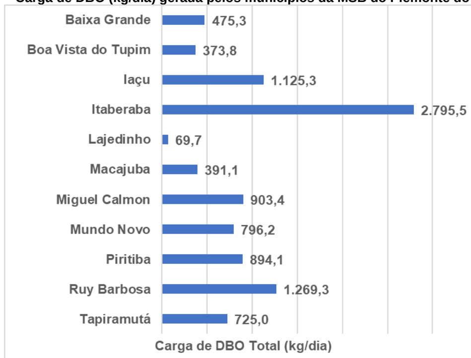
Figura 90 – Carga de DBO (kg/dia) gerada pelos municípios da MSB do Piemonte do Paraguaçu
