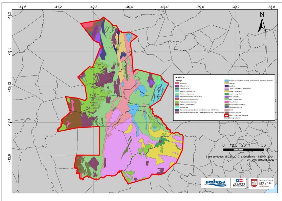
Figura 14 – Mapa geológico da MSB/PIP
