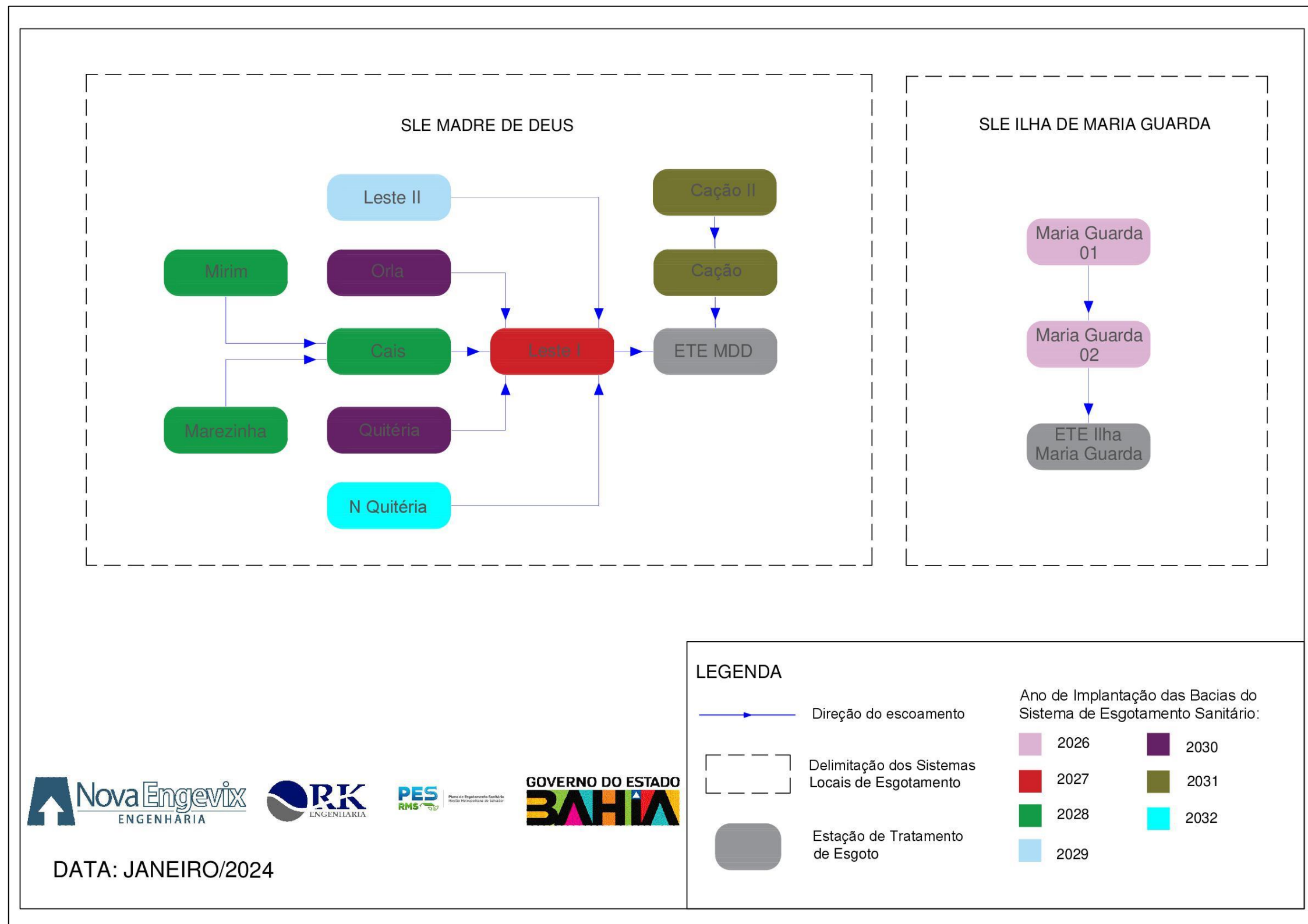
FIGURA 3.1 - Fluxograma da Alternativa Seleccionada
