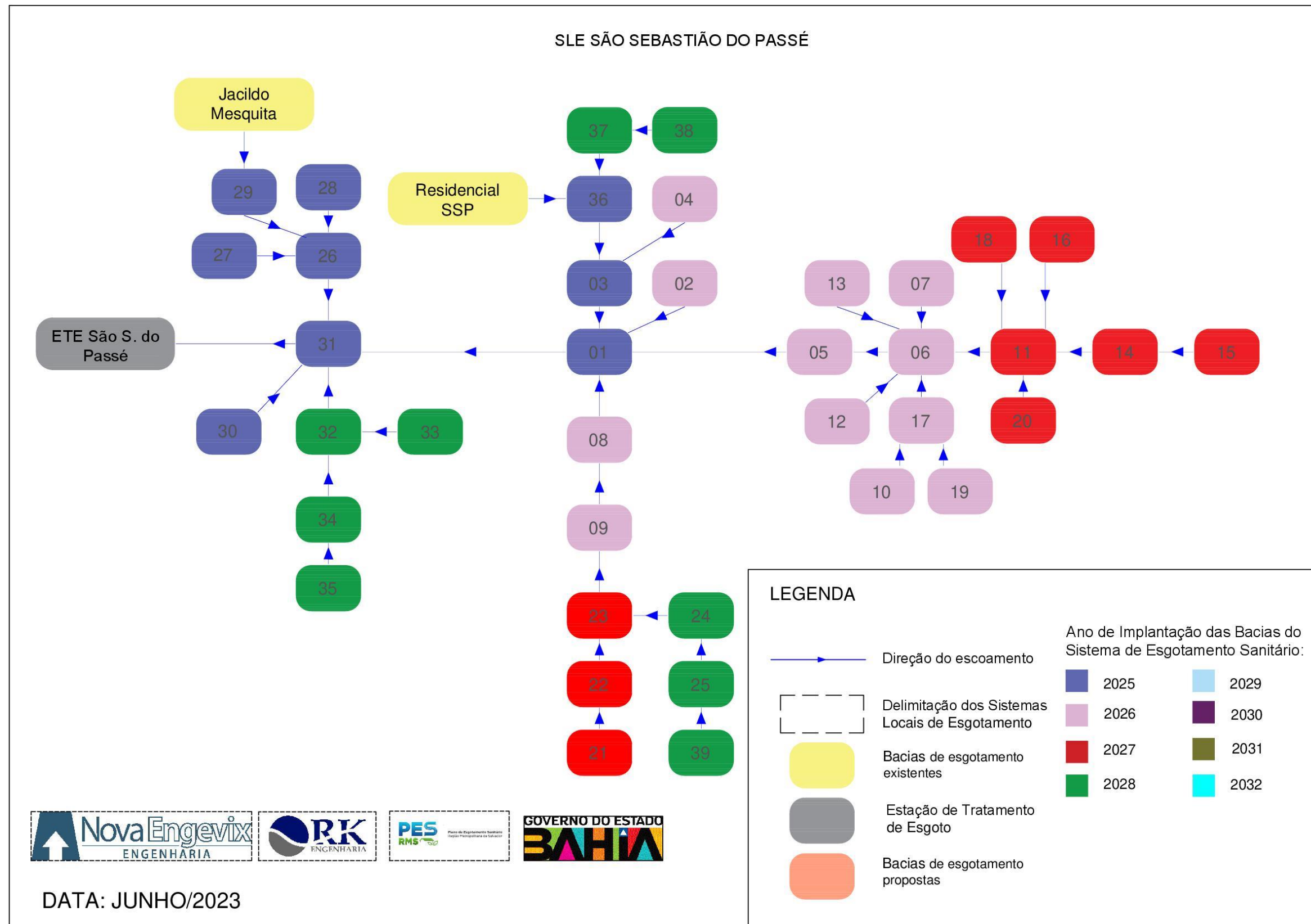
FIGURA 3-1 - Fluxograma da Alternativa Seleccionada Fonte: Consórcio (2023)
