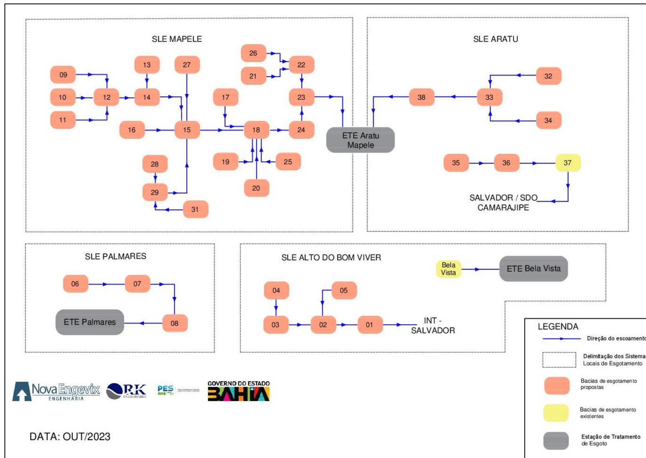
FIGURA 2.2 - Fluxograma das bacias de esgotamento sanitário da Alternativa Seleccionada Fonte: Consórcio (2023).
