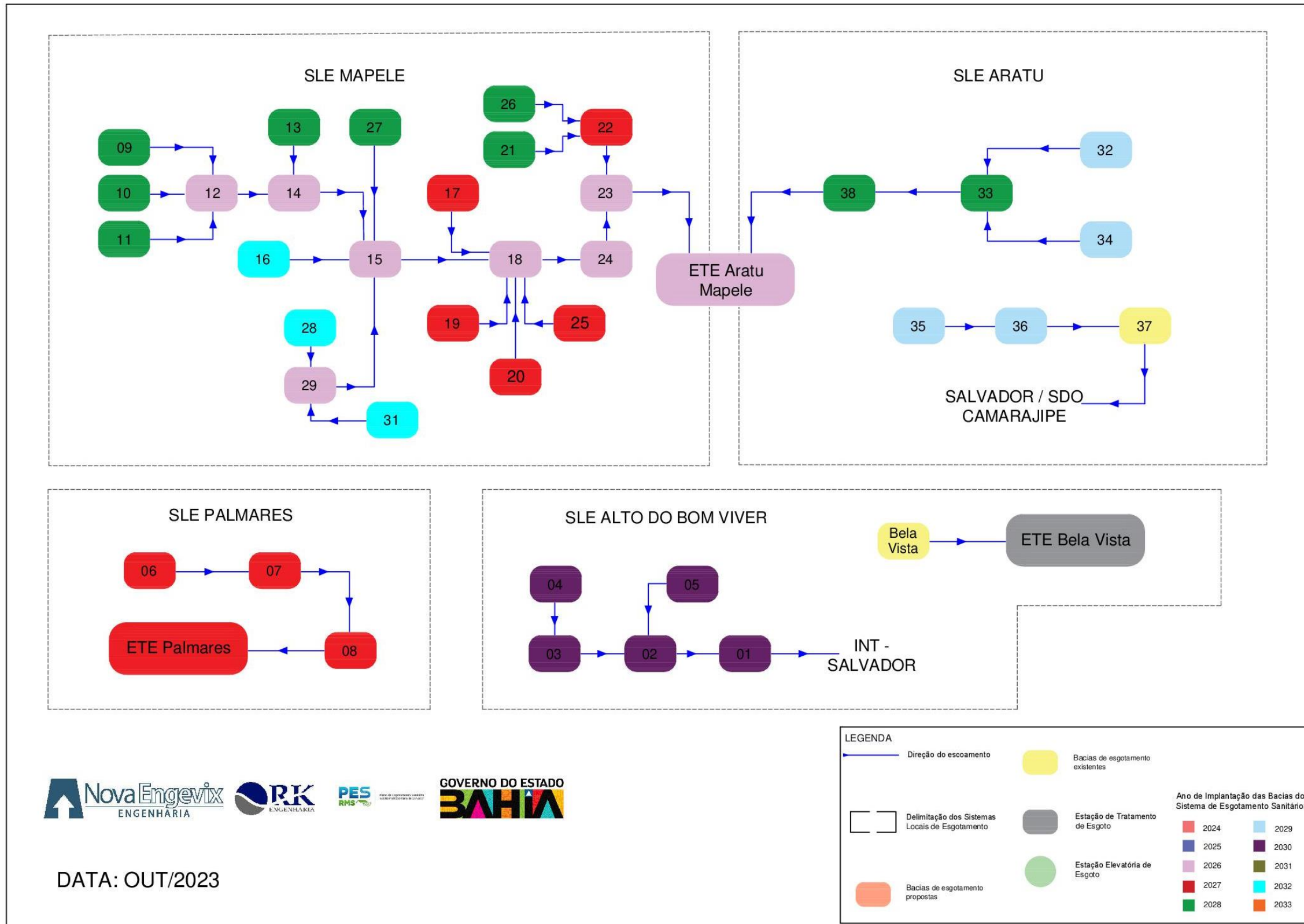
FIGURA 3.2 - Fluxograma da Alternativa Seleccionada Fonte: Consórcio (2023)
