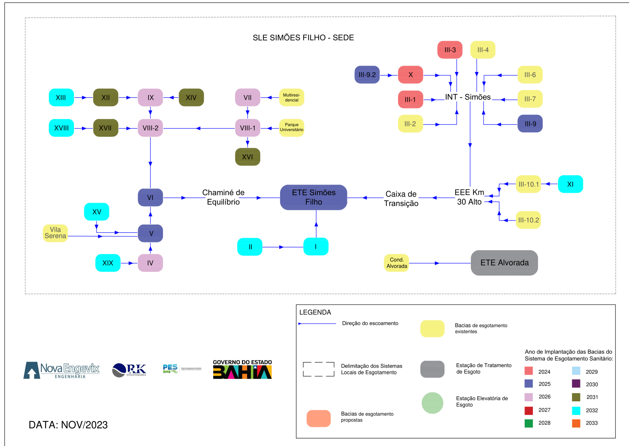
FIGURA 3.1 - Fluxograma da Alternativa Seleccionada Fonte: Consórcio (2023)
