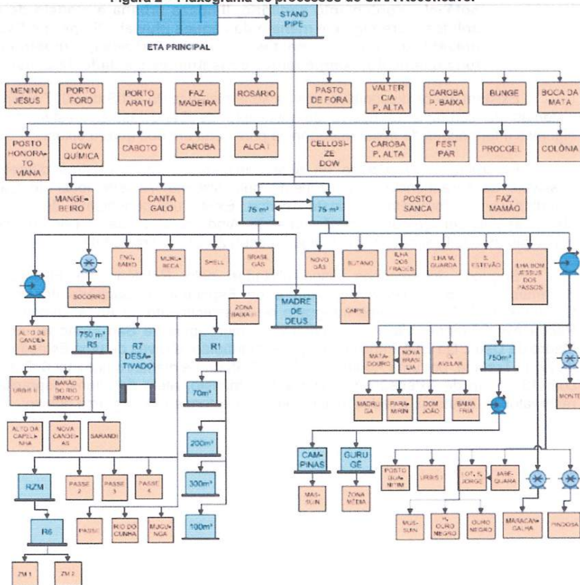
Figura 2 – Fluxograma de processos do SIAA Recôncavo.
