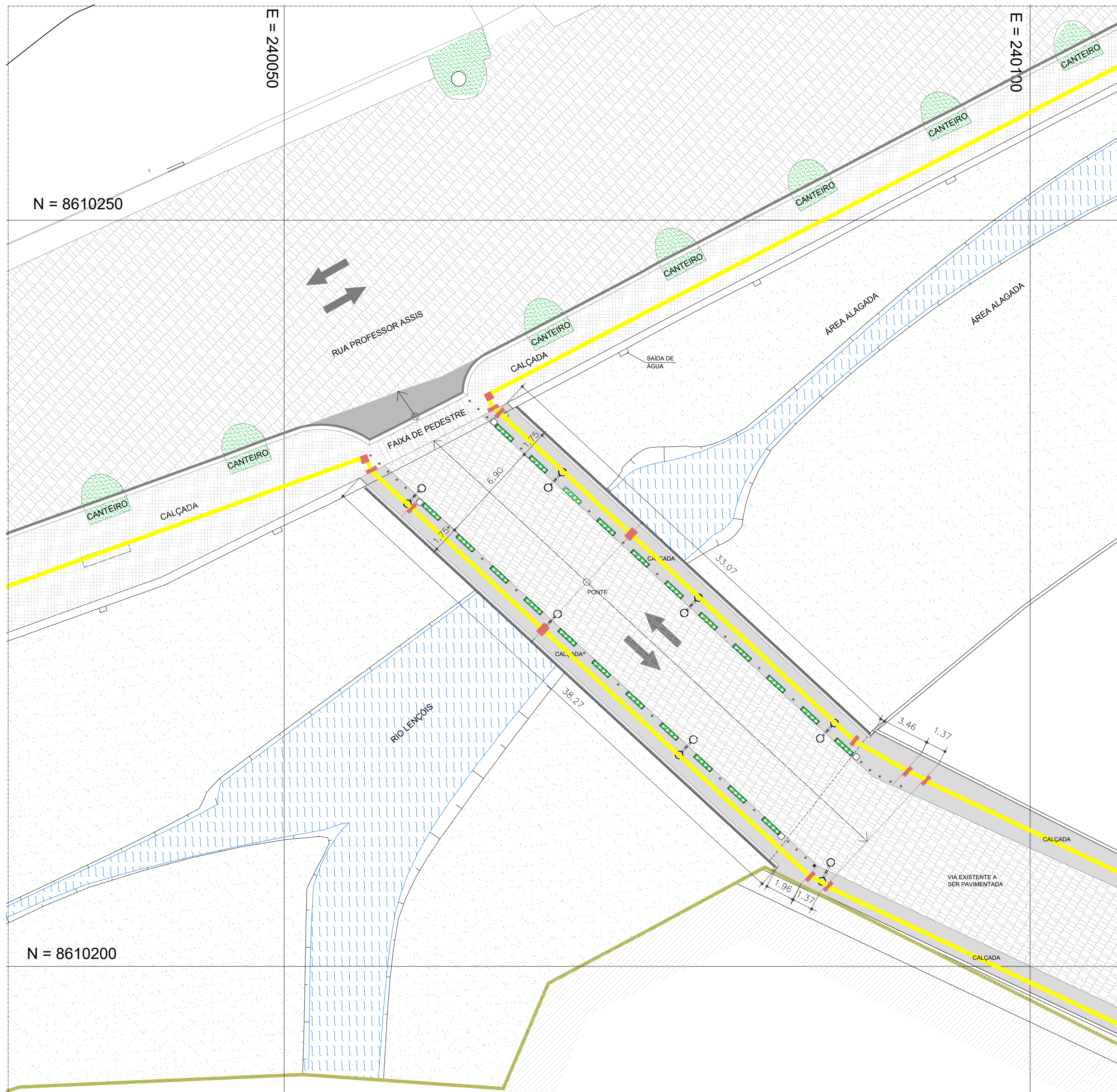
PLANTA BAIXA ESC 1/200
