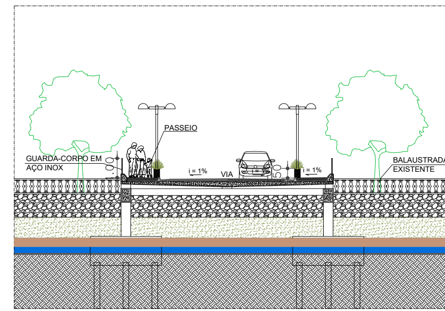
CORTE BB ESC 1/200
