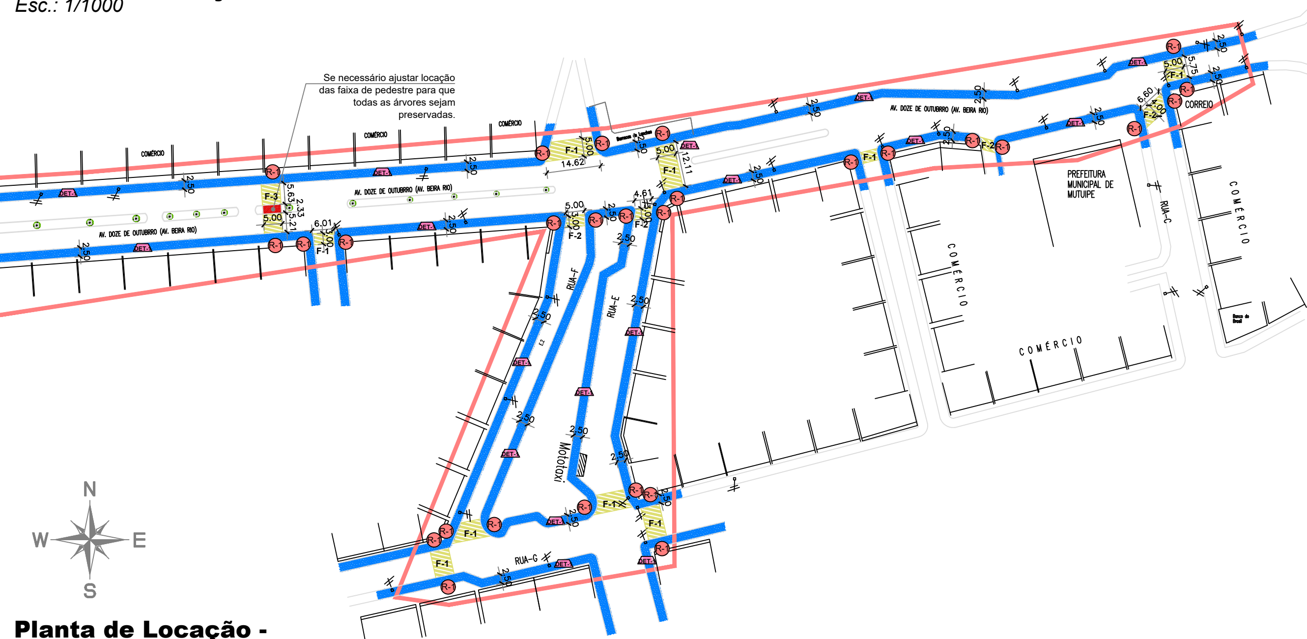
Planta de Localização - Área de intervenção 01 Esc.: 1/1000
