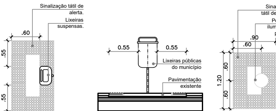
Detalhe-01 Sinalização para lixeiras Esc.: 1/50
