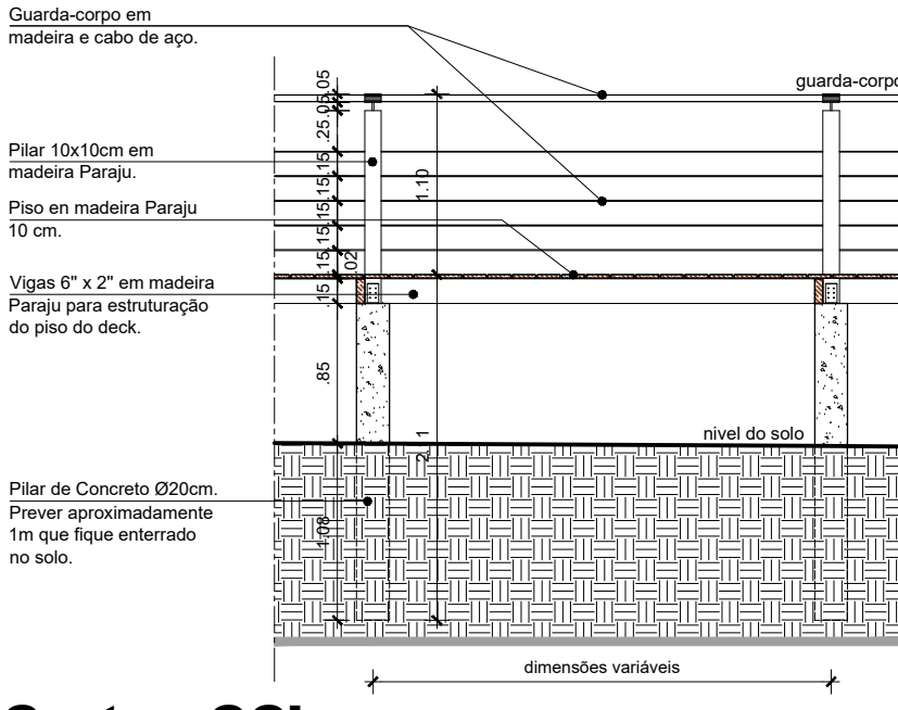
Corte - CC' Esc.: 1/50
