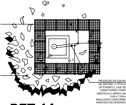
DET-14 Sinalização para árvores Esc.: 1/50
