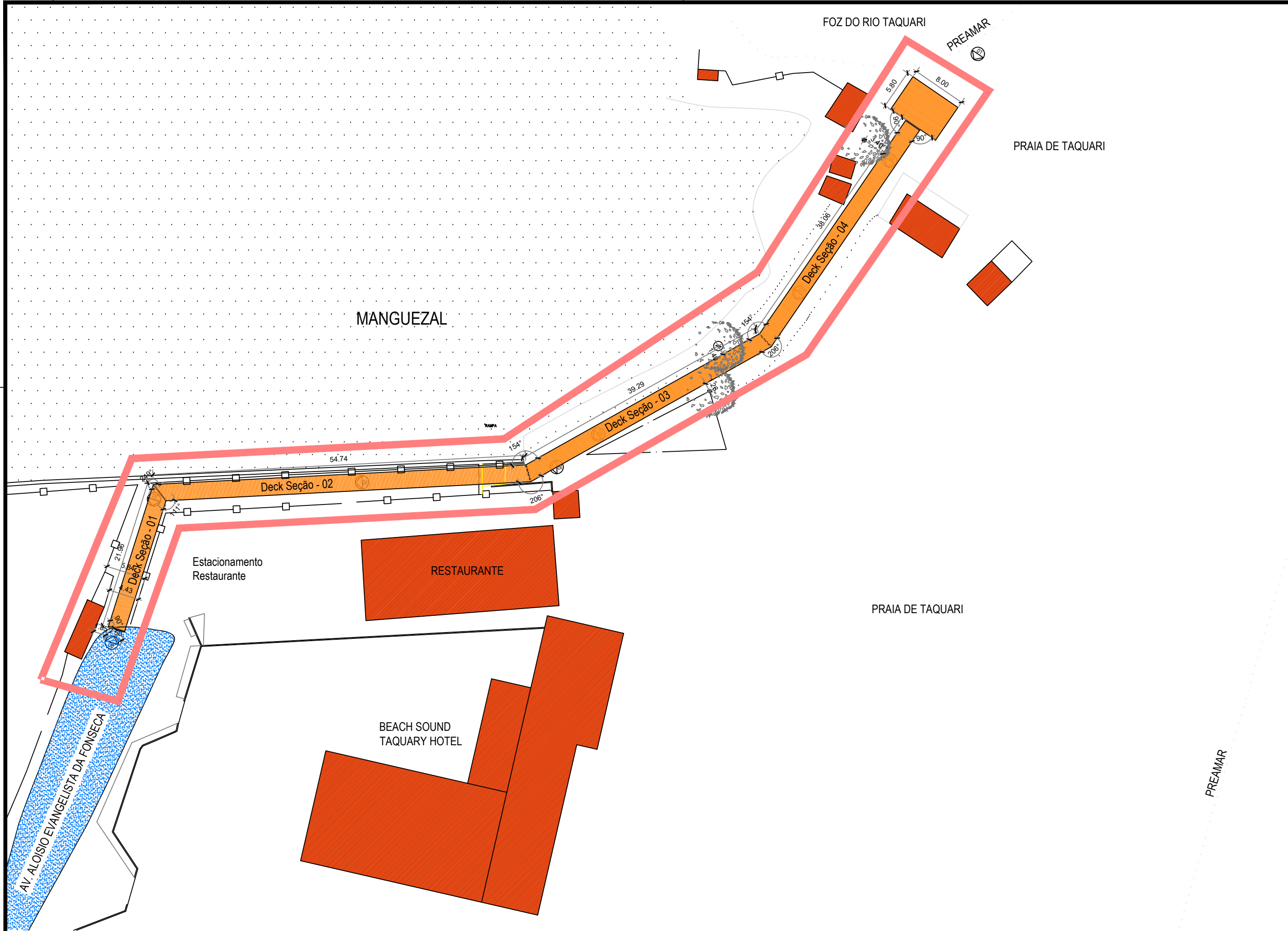
Planta de Locação - Área de interveção Esc.: 1/500
