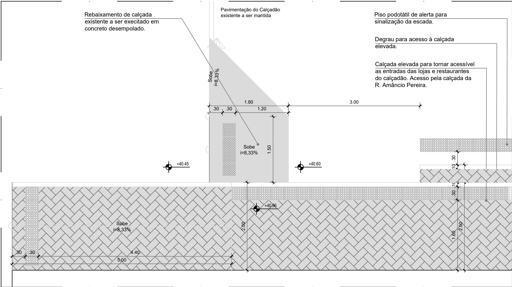
DET-01 - Calçada Elevada Planta Baixa Esc.: 1/500
