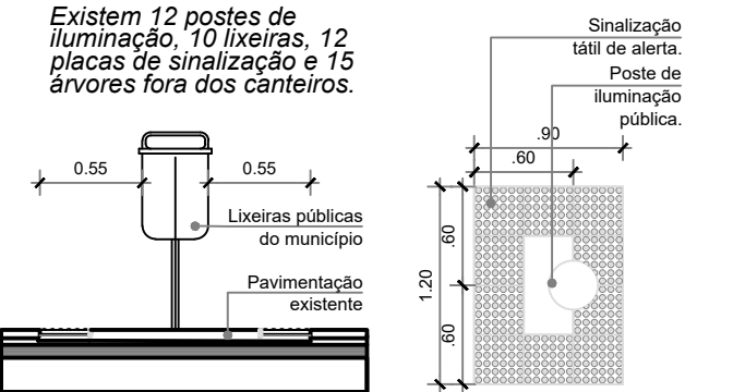
DET-01 Vista Frontal Sinalização para lixeiras Esc.: 1/50
