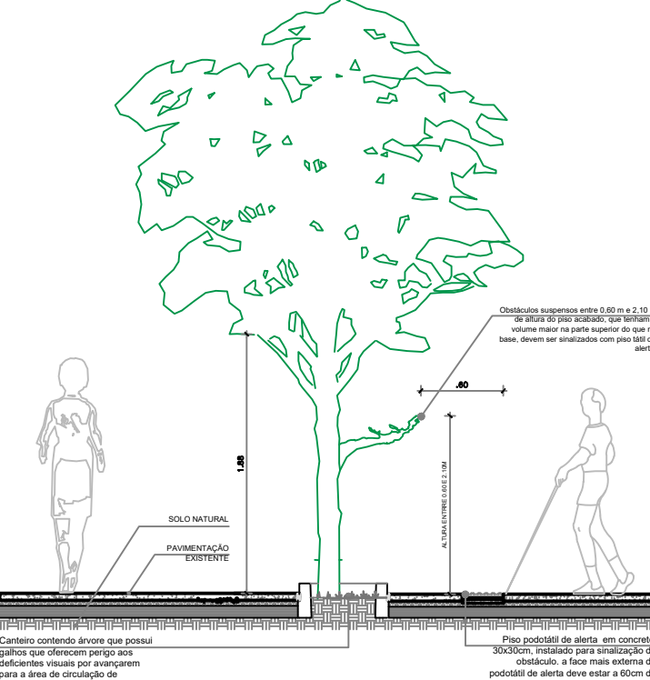
DET-04 Sinalização para árvores - Vista frontal Esc.: 1/50
