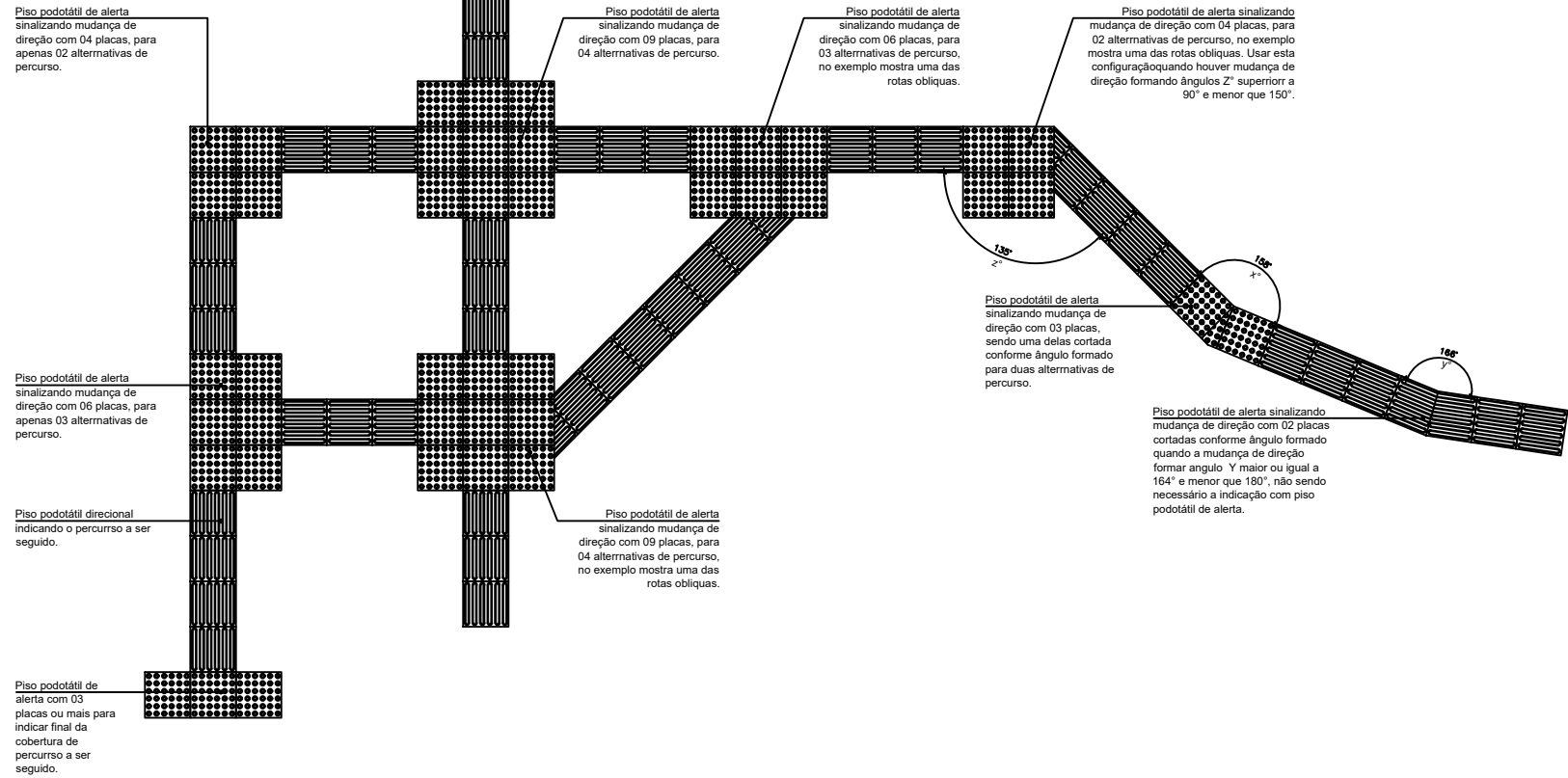
Piso Podotátil - Exemplo de articulação Esc.: 1/25
