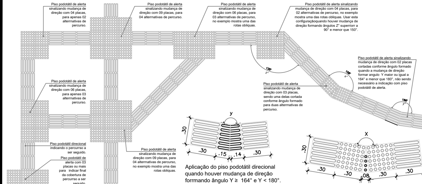
Piso Podotátil - Exemplo de articulação
