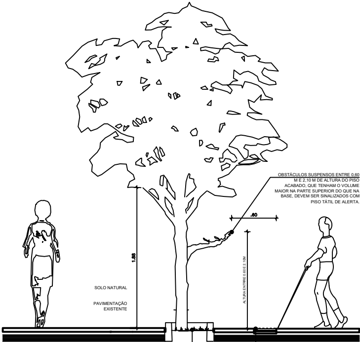
DET-14 Sinalização para árvores Esc.: 1/50
