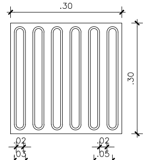
DET-02 Sinalização para postes ilum. Esc.: 1/50
