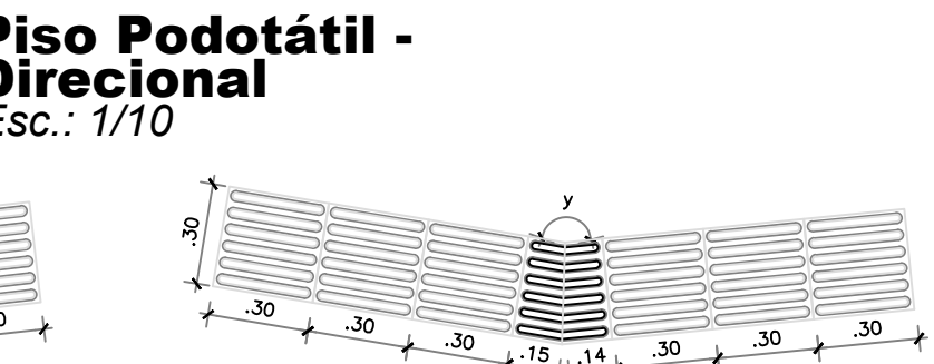
Piso Podotátil - Direcional Esc.: 1/10
