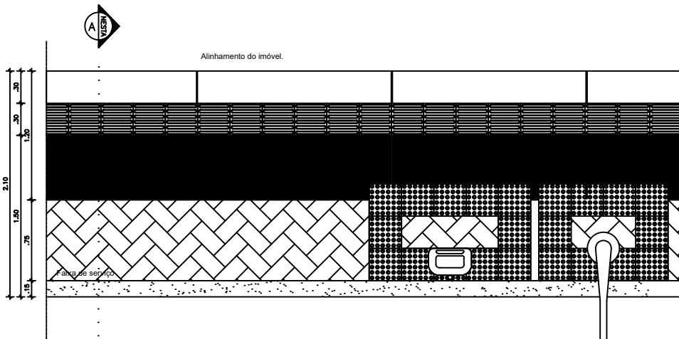
DET-14 Sinalização para árvores - Vista frontal Esc.: 1/50
