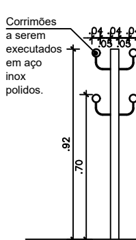
Corte - DET-8 corrimões centrais Esc.: 1/20
