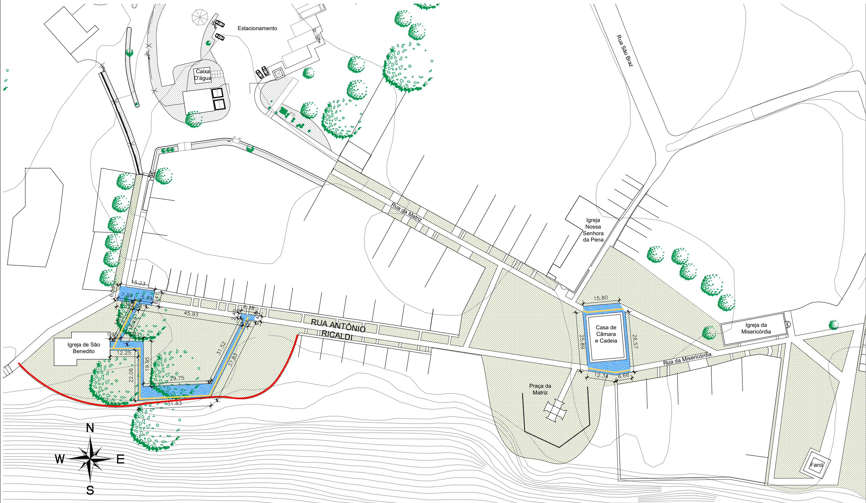
Planta de Localização - Área de intervenção Esc.: 1/1000
