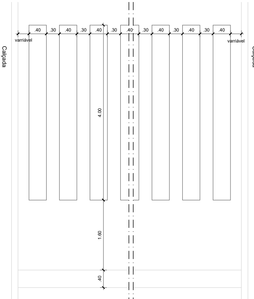
DET-03 - Pintura para faixa de travessia de pedestres Esc.: 1/50
