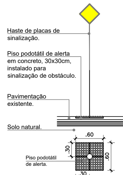
DET-02 Sinalização para placas de sinalização Esc.: 1/50
