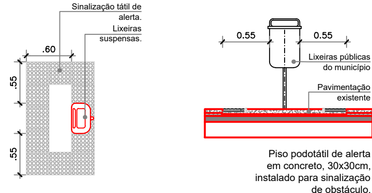
Planta Baixa Vista Frontal Esc.: 1/50
