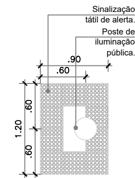
Planta Baixa Esc.: 1/50
