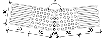
Piso podotátil direcional Mudança de direção tipo 02 Esc.: 1/10
