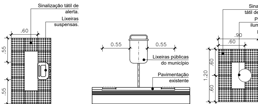
DET-01 Sinalização para lixeiras Esc.: 1/50
