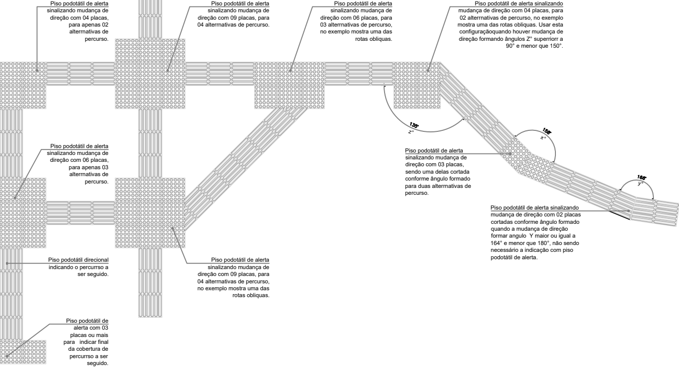
Piso Podotátil - Exemplo de articulação Esc.: 1/25
