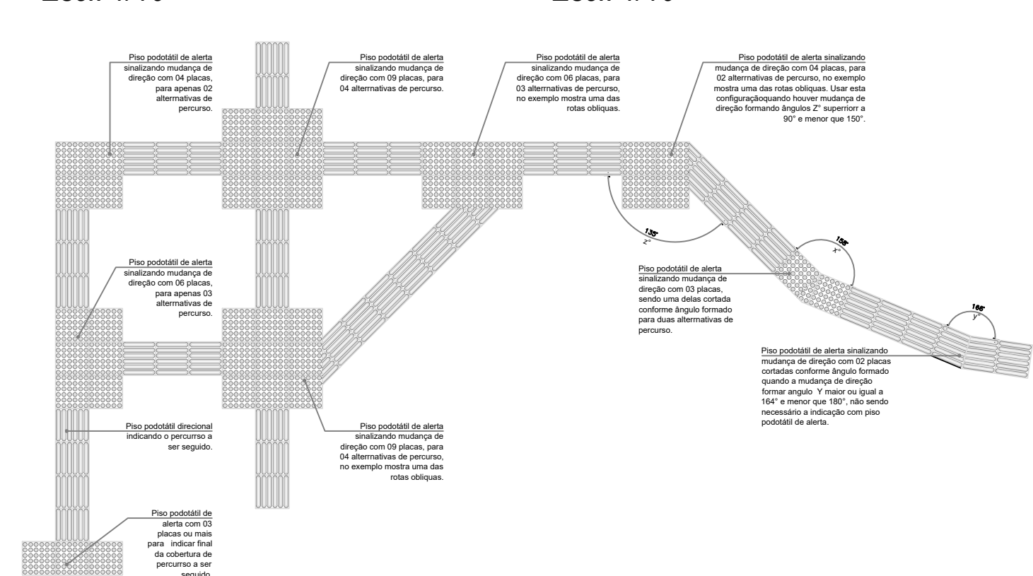
Piso Podotátil - Exemplo de articulação Esc.: 1/25
