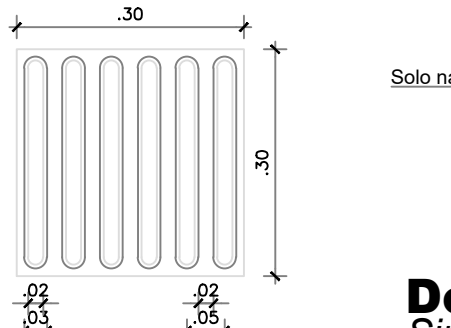
Piso Podotátil - Direcional Esc.: 1/10
