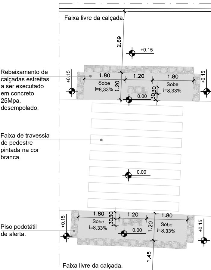
Planta de Baixa - Zona 04 Esc.: 1/100
