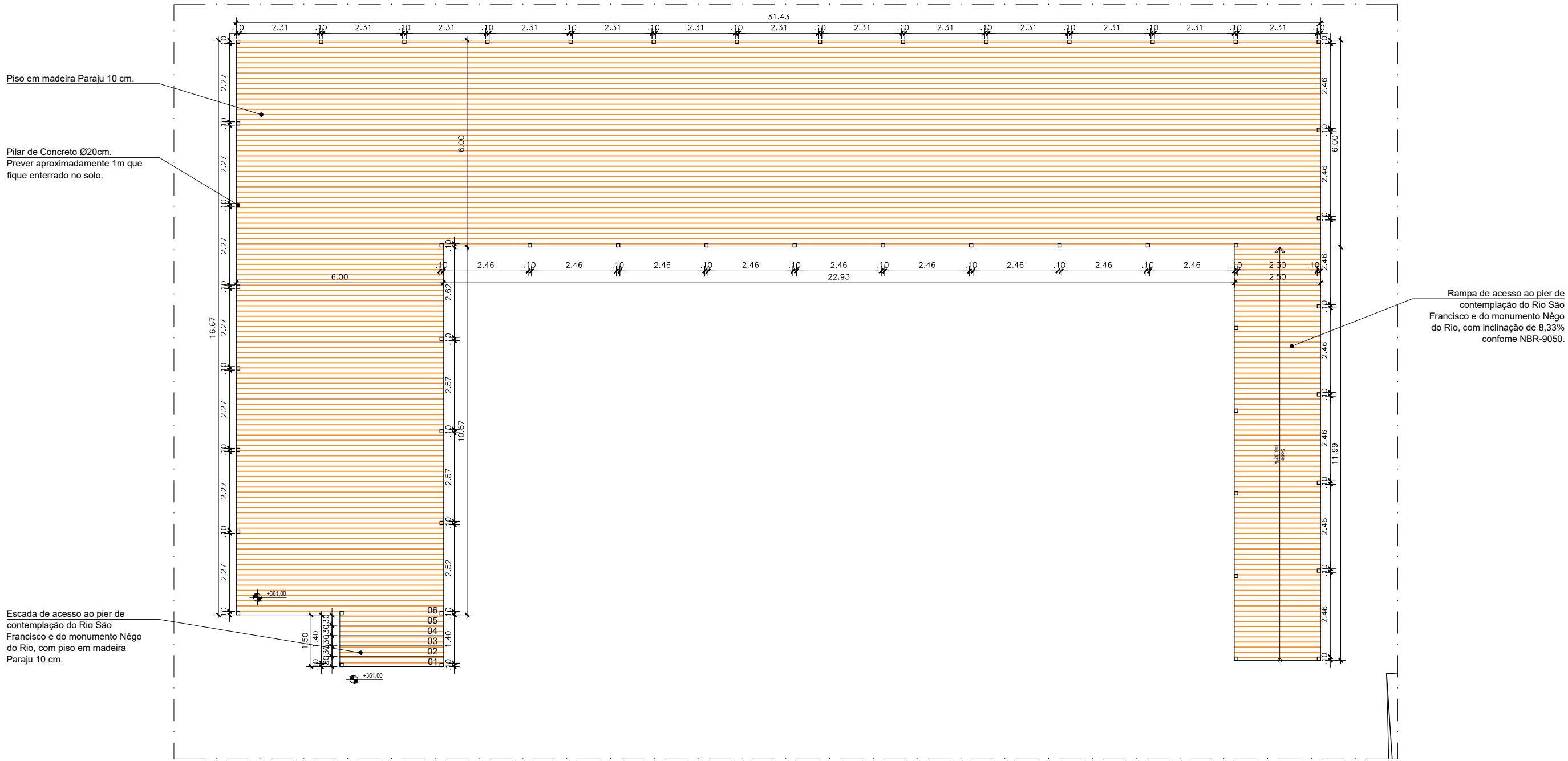
Zona 01 - Planta Baixa Esc.: 1/100
