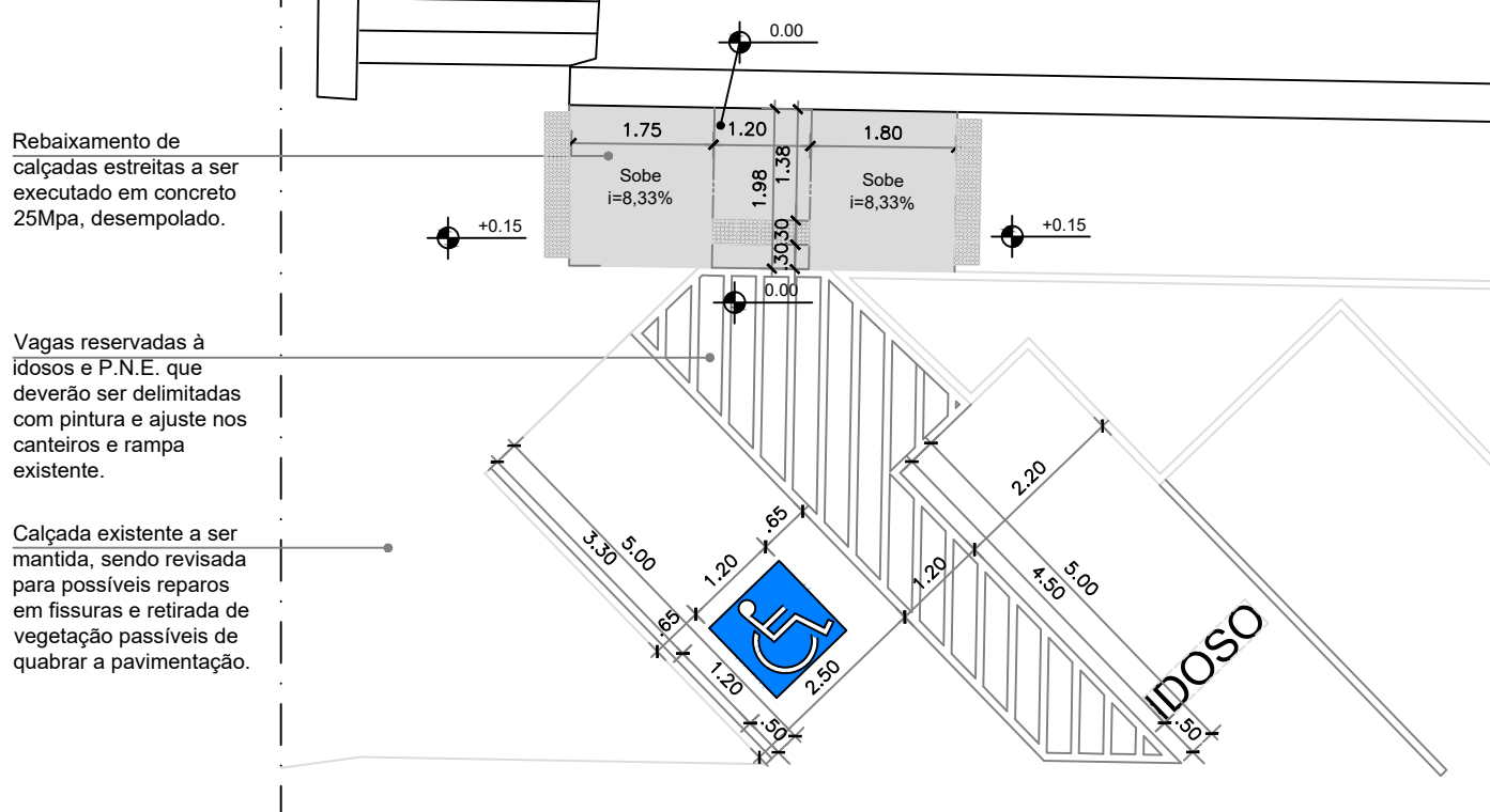
Planta de Baixa - Zona 01 Esc.: 1/100
