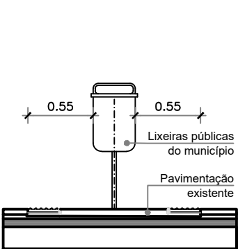
Detalhe-01 Vista Frontal Sinalização para lixeiras Esc.: 1/50
