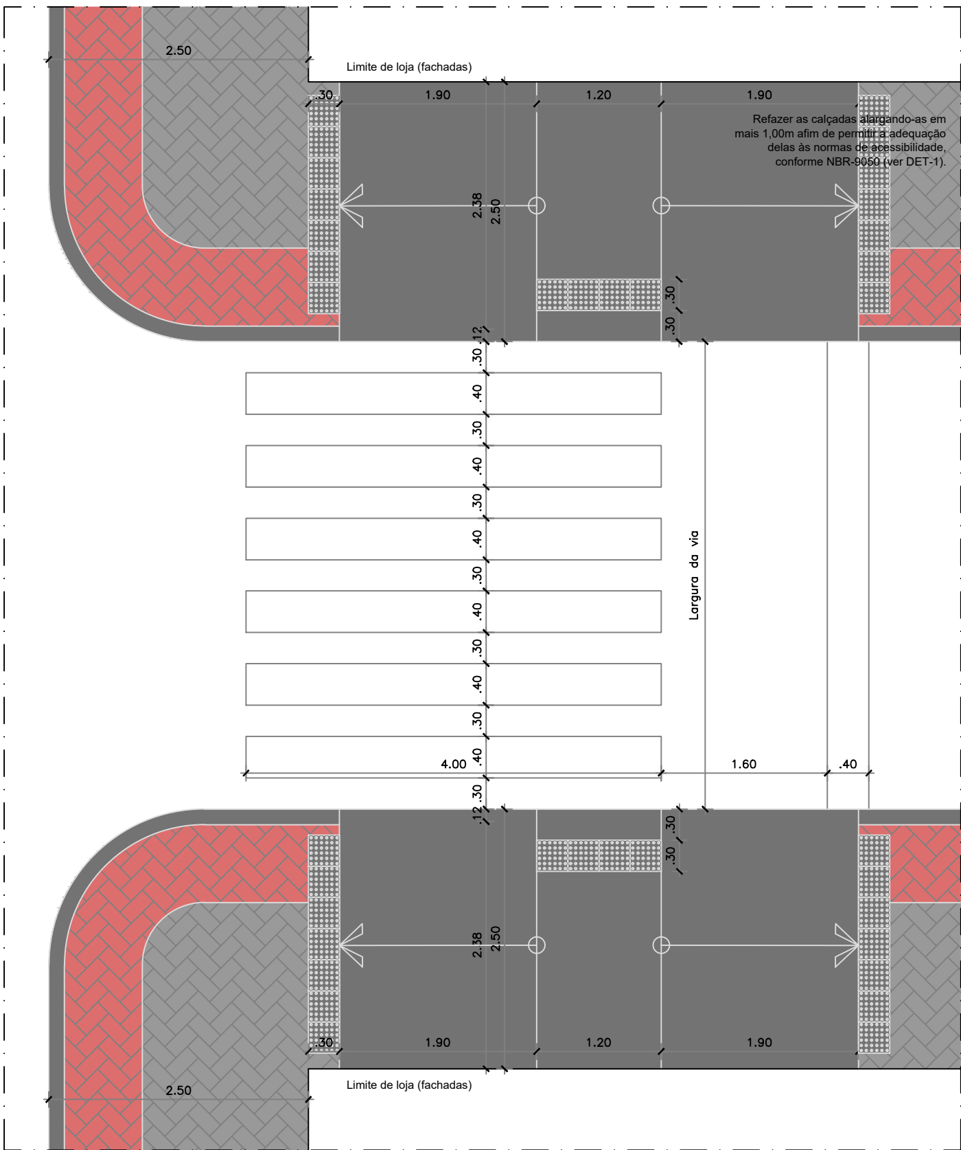
Planta Baixa - F-1
