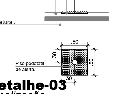
Detalhe-03 Sinalização para placas de sinalização Esc.: 1/50
