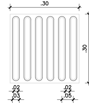
DET-01 Sinalização para postes ilum. Esc.: 1/50 DET-01A Sinalização para postes ilum. com lixeiras Esc.: 1/50
