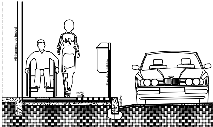
EXEMPLO CALÇADA Corte AA' Esc.: 1/50
