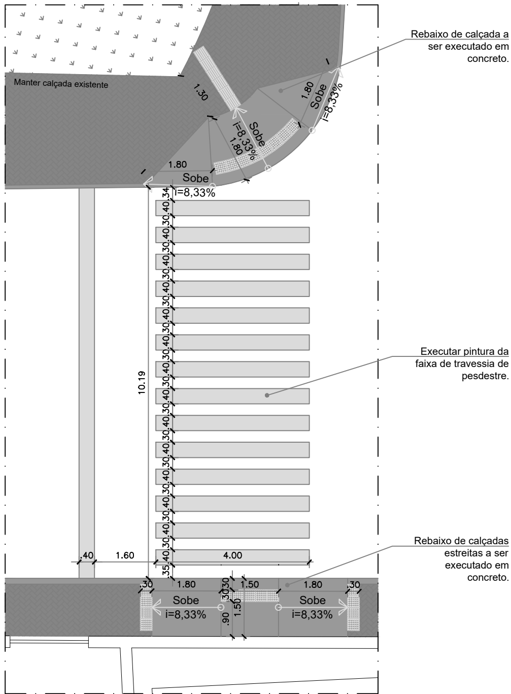
DET-01 Faixa de travessia de pedestes e ebaixamento de calçadas Esc.: 1/100
