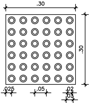
DET-10 Sinalização para lixeiras Esc.: 1/50
