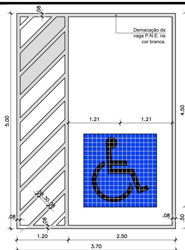
Det-04 Pintura de vaga de estacion. p/ P.N.E. Esc.: 1/50
