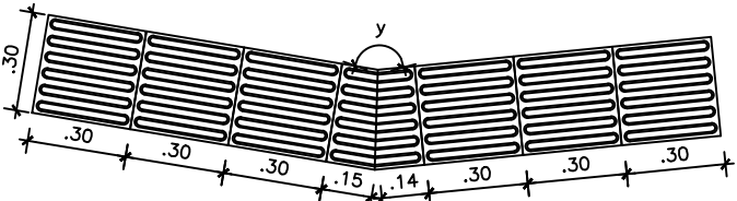
Piso podotátil direcional Mudança de direção tipo 02 Esc.: 1/10
