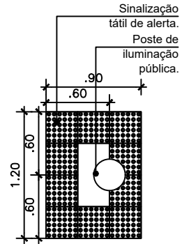
DET-11 Sinalização para postes ilum. Esc.: 1/50
