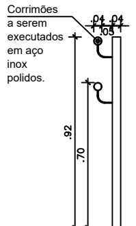
Corte - DET-7 (para corrimões das extremidades de escada e rampas) Esc.: 1/20
