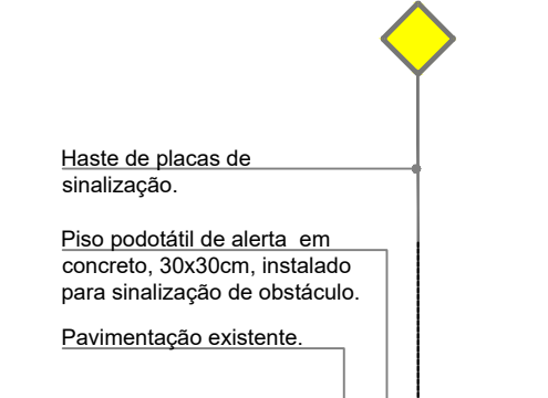
DET-03 Sinalização para placas de sinalização Esc.: 1/50
