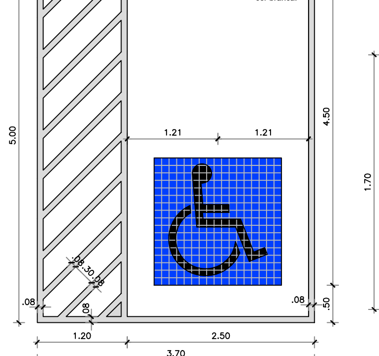
Detalhe-07 Pintura de vaga de estacionamento para P.N.E. Esc.: 1/50
