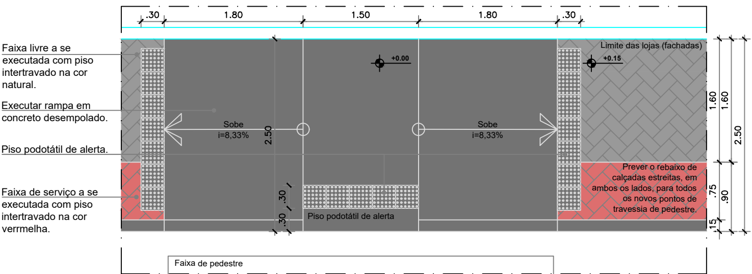
Planta Baixa - R-1 Esc.: 1/50
