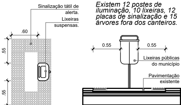
DET-01 Sinalização para lixeiras Esc.: 1/50
