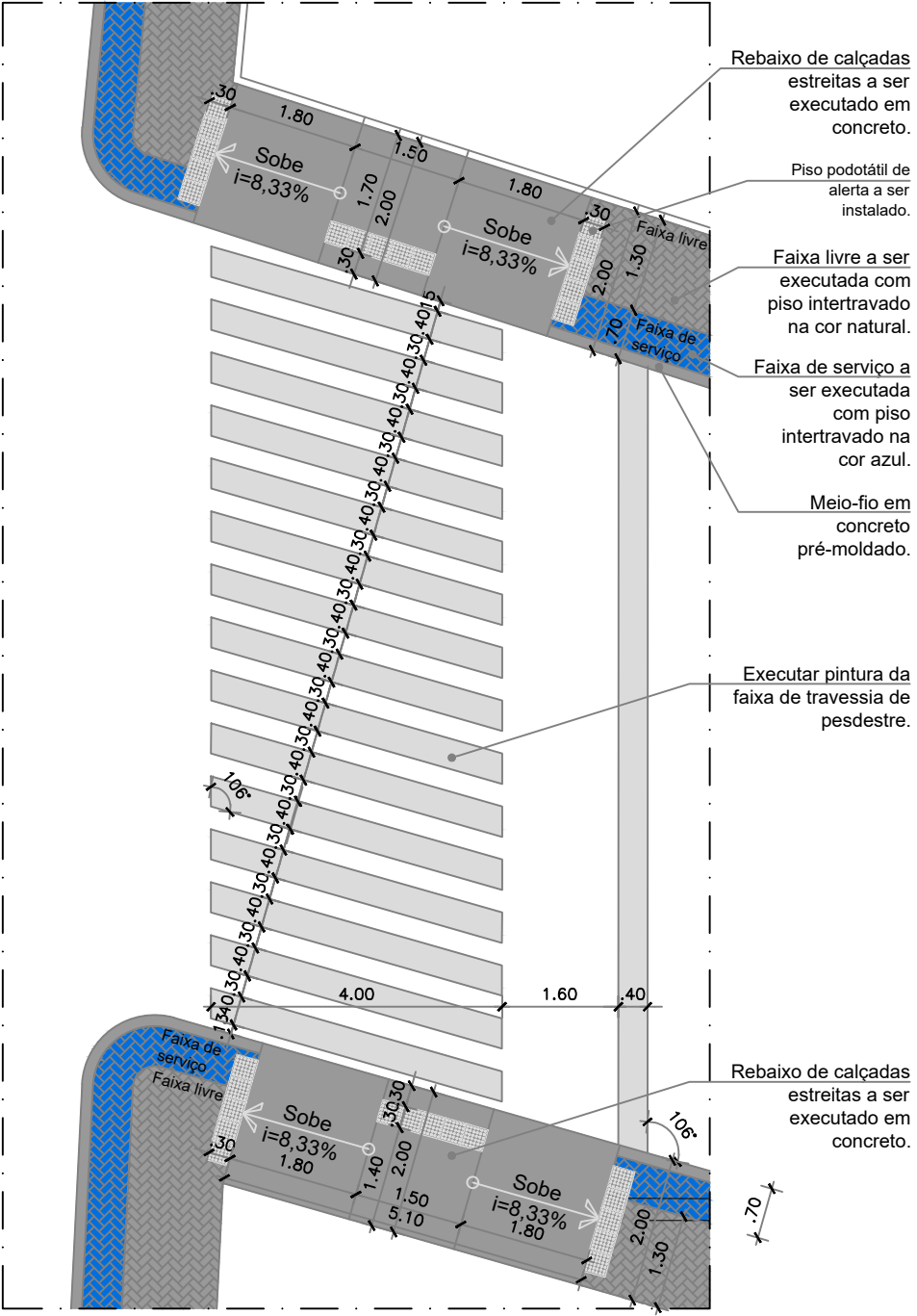
DET-03 Faixa de travessia de pedestes e ebaixamento de calçadas Esc.: 1/100
