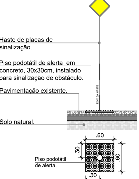
DET-03 Sinalização para placas de sinalização Esc.: 1/50
