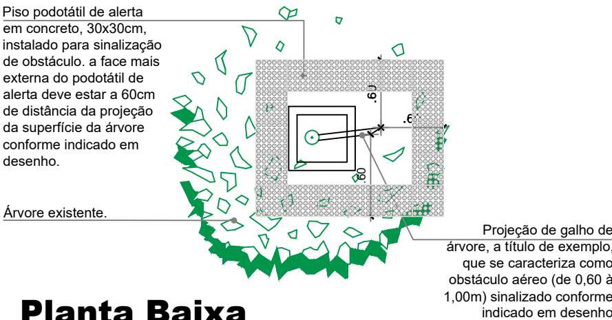
Planta Baixa Esc.: 1/50
