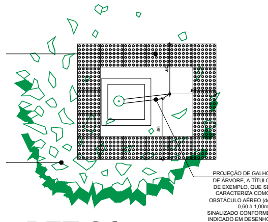
DET-04 Sinalização para árvores Esc.: 1/50
