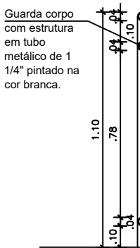
Corte DET-9 Esc.: 1/20
