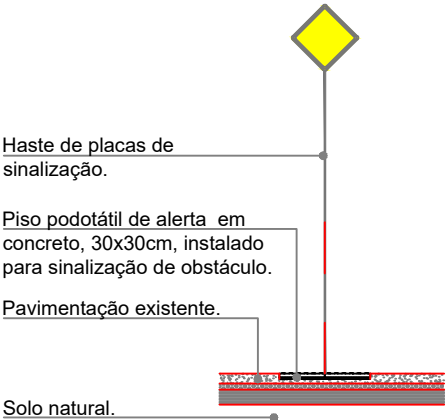
Vista Frontal Esc.: 1/50
