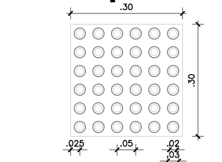
Piso Podotátil - Alerta Esc.: 1/10
