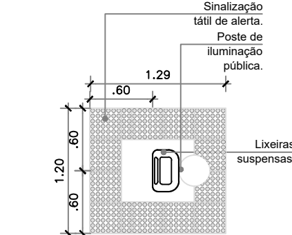
DET-01 Sinalização para postes ilum. Esc.: 1/50 DET-01A Sinalização para postes ilum. com lixeiras Esc.: 1/50
