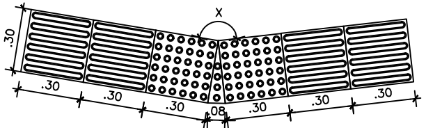
Piso podotátil direcional Mudança de direção tipo 01 Esc.: 1/10
