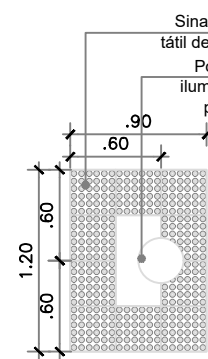
Detalhe-02 Sinalização para postes ilum. Esc.: 1/50
