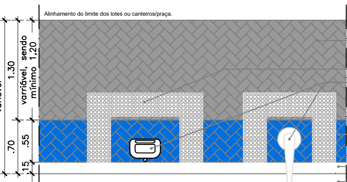
Pavimentação das Calçadas Sinalização para placas de sinalização Esc.: 1/50
