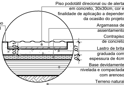
Detalhe 05 - Instalação de piso podotátil Esc.: 1/10
