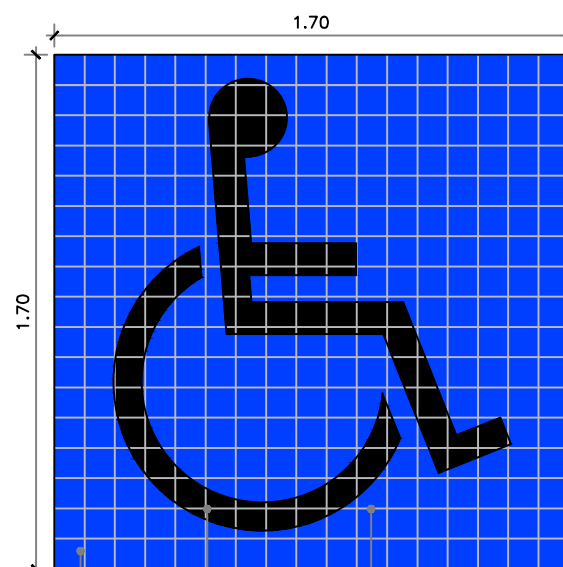
Det-05 Pintura do símbolo intenacioanal parra acesso a P.N.E. Esc.: 1/25
