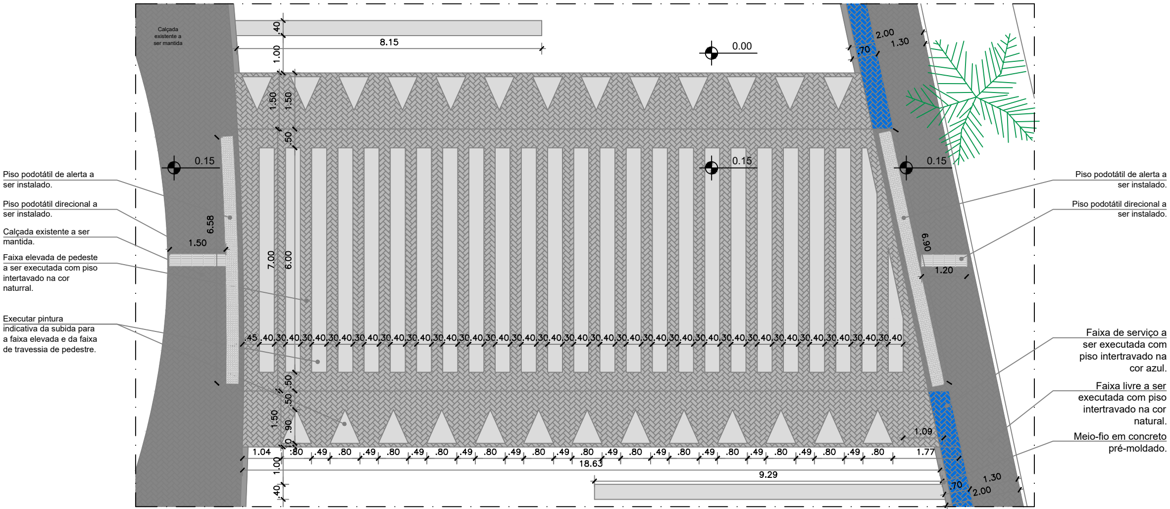
DET-02 Faixa de travessia de pedestes elevada Esc.: 1/100
