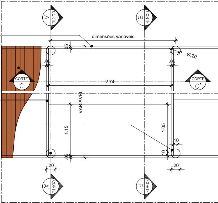
Planta baixa Deck Esc.: 1/50
