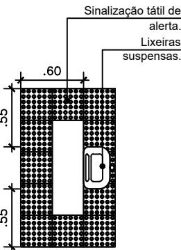
DET-10 Sinalização para lixeiras Esc.: 1/50
