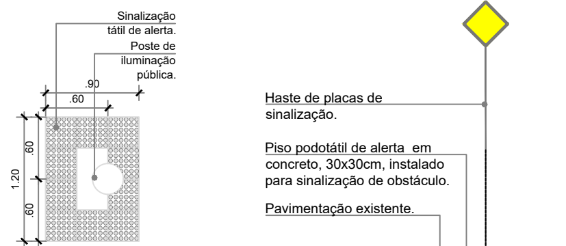
DET-02 Sinalização para postes ilum. Esc.: 1/50
