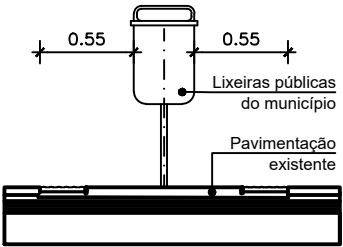
DET-10 Vista Frontal Sinalização para lixeiras Esc.: 1/50
