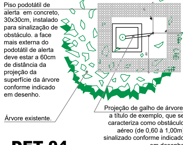
DET-04 Sinalização para árvores Esc.: 1/50
