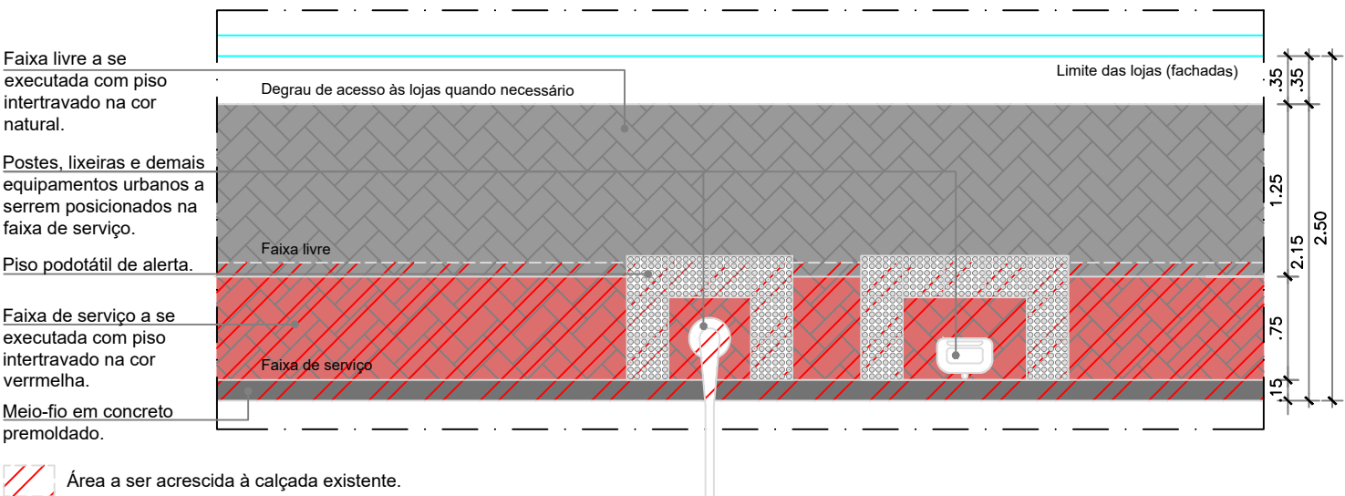
Planta Baixa - DET-1 Esc.: 1/50
