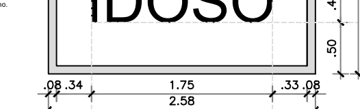
Detalhe-06 Pintura de vaga estacionamento para idoso Esc.: 1/50
