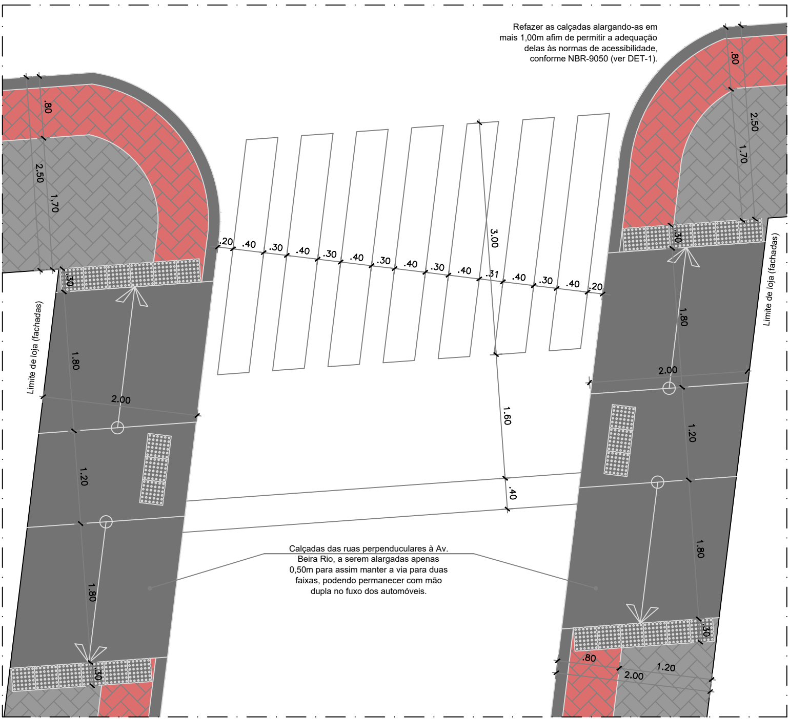
Planta Baixa - DET-2
