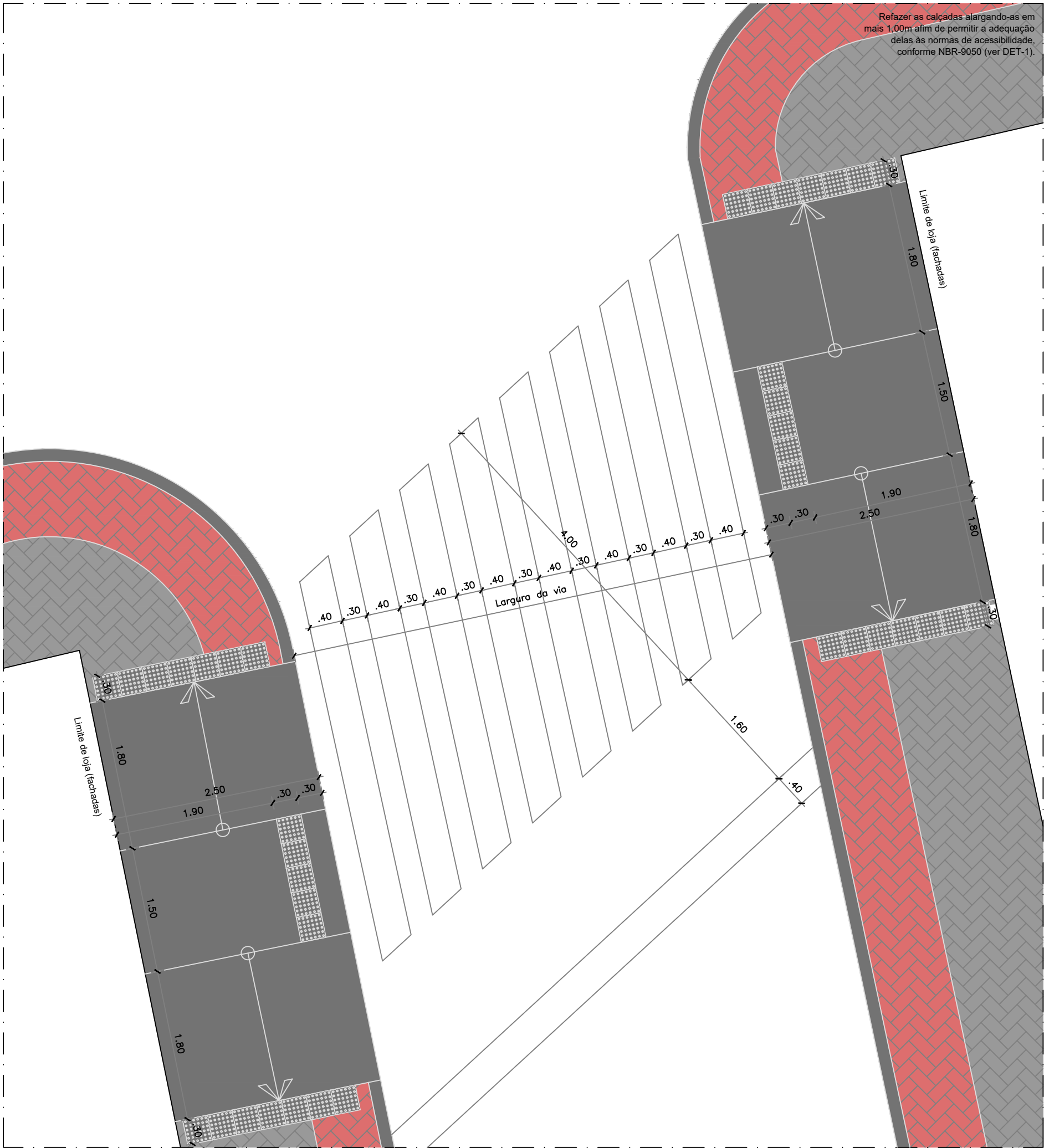
Planta Baixa - F-2
