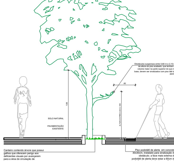
DET-04 Sinalização para árvores - Vista frontal Esc.: 1/50
