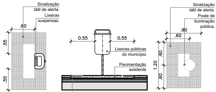
DET-01 Sinalização para lixeiras Esc.: 1/50
