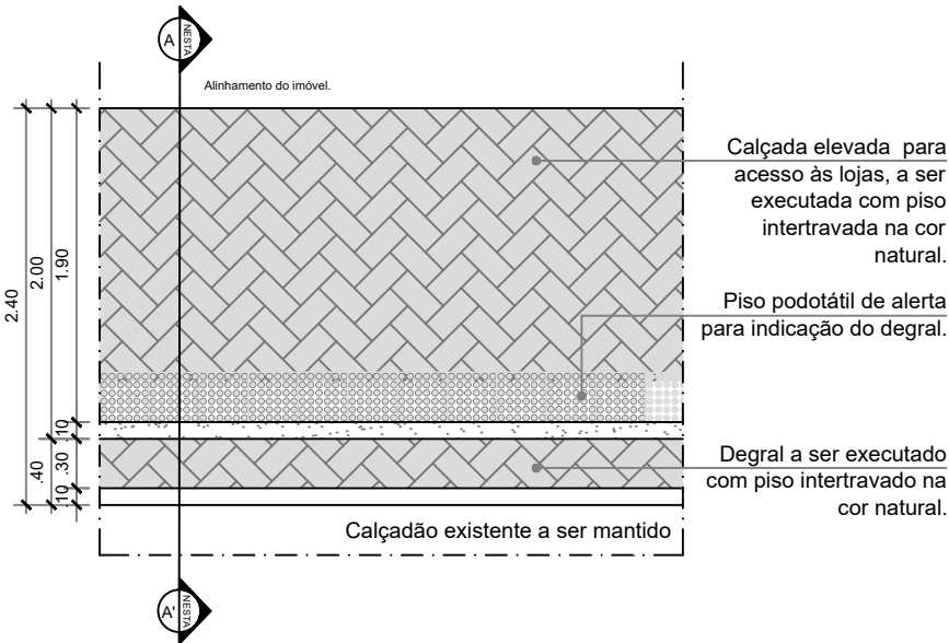
DET-02 - Calçada Elevada Planta Baixa Esc.: 1/50
