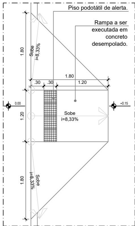
DET-04 Planta Baixa Esc.: 1/50
