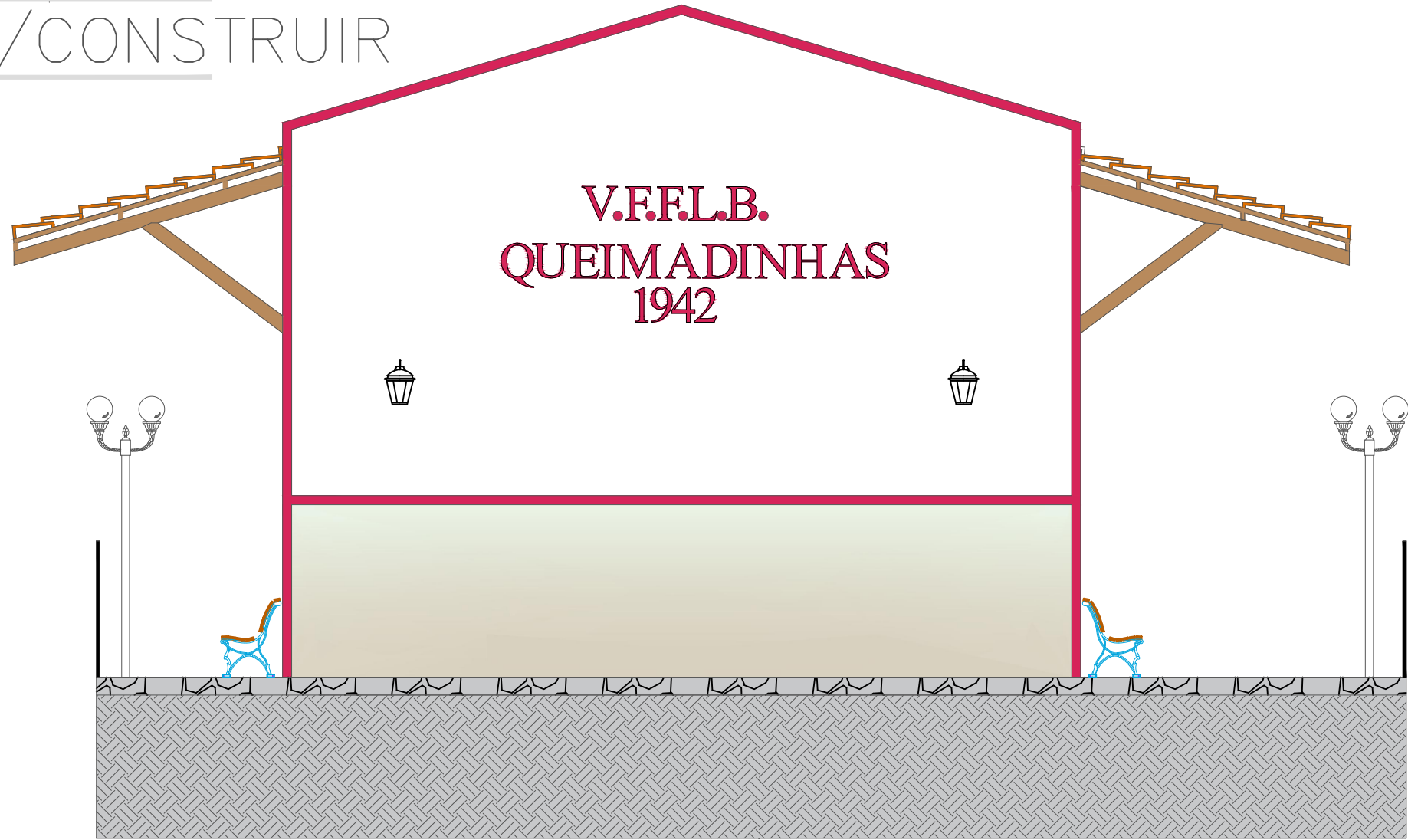
FACHADA NORDESTE ESC. 1:100
