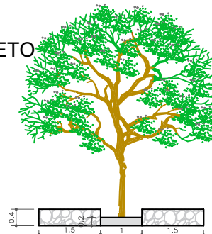
VISTA LATERAL
