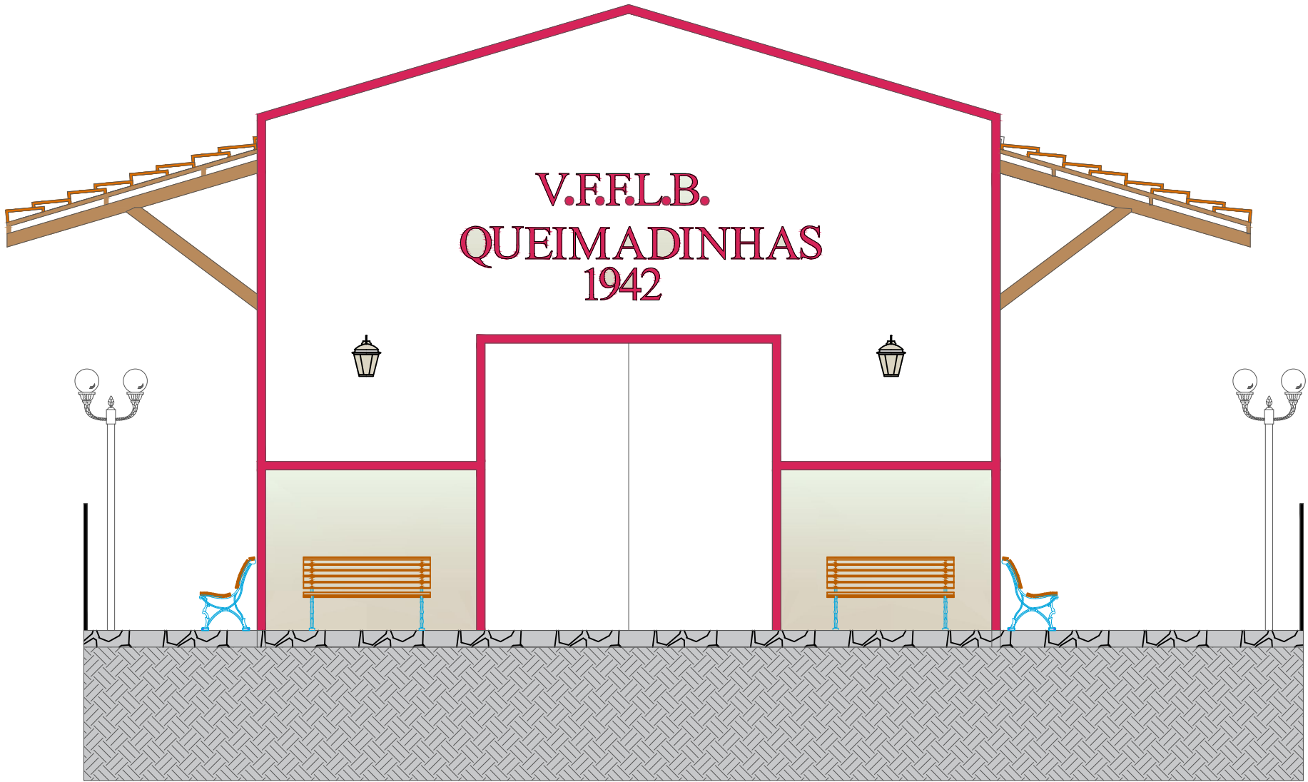
FACHADA SUDOESTE ESC. 1:100
