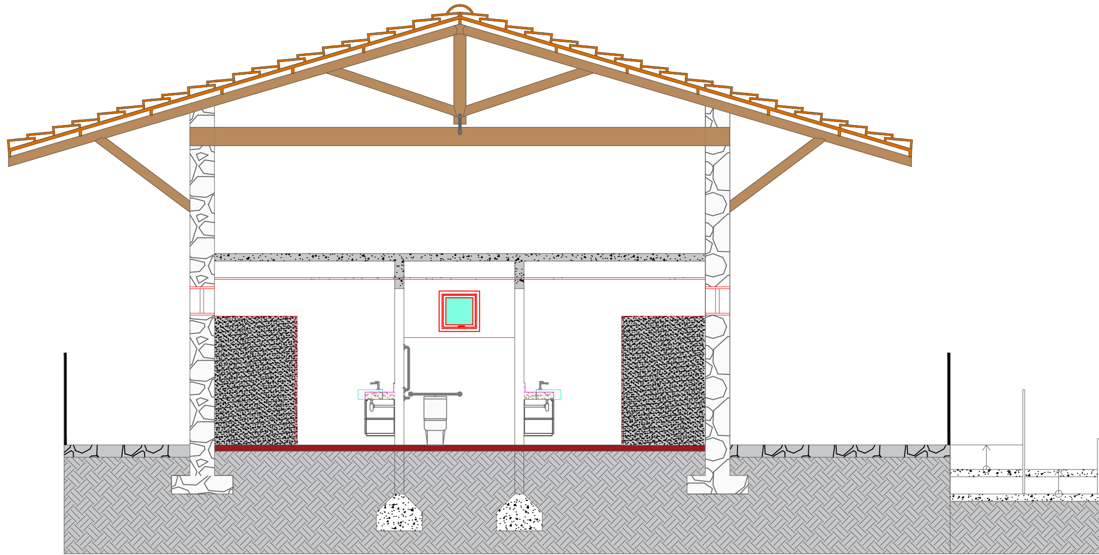
CORTE AA ESC. 1:100
