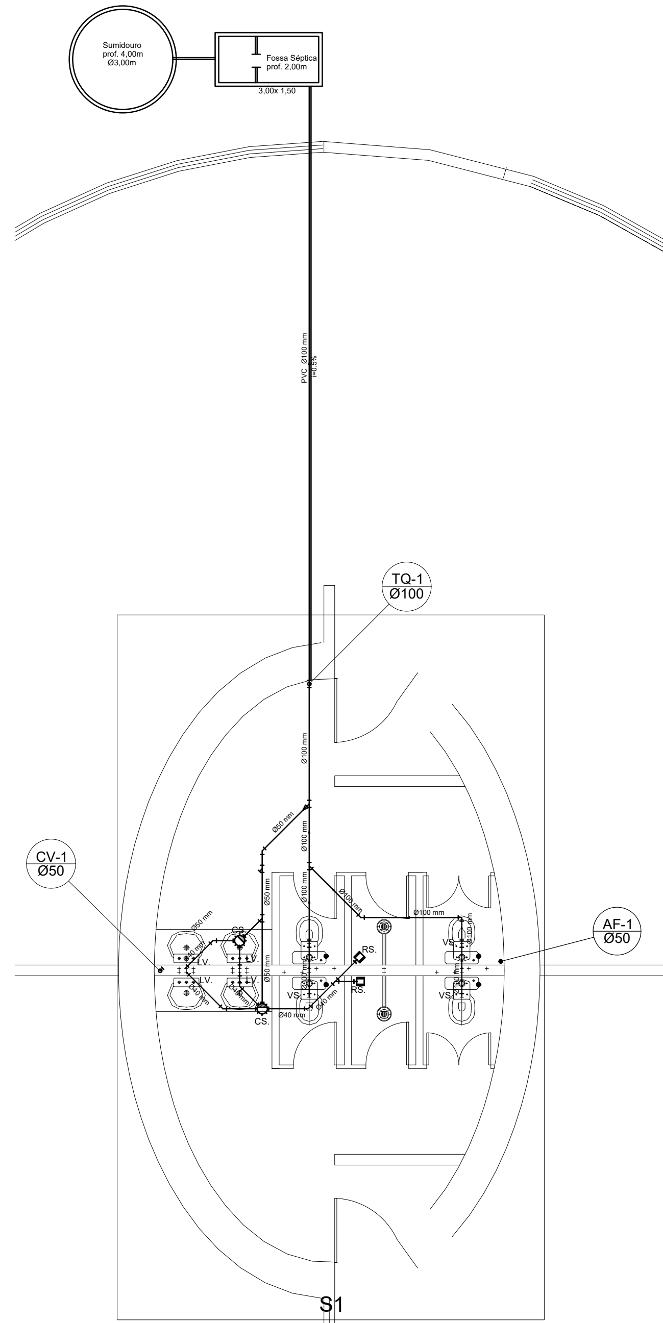
01 PLANTA BAIXA Esc: 1/100 ESGOTO SANITÁRIO TÉRREO
