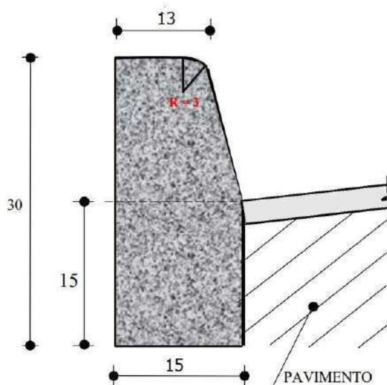
Imagem 3: Dimensões do meio fio a serem utilizados
