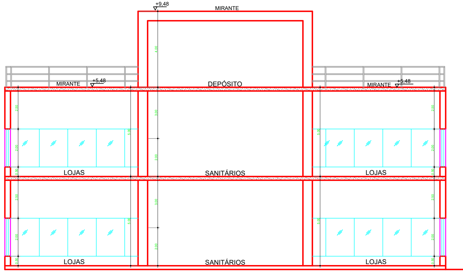
CORTE CC' Esc.: 1/75
