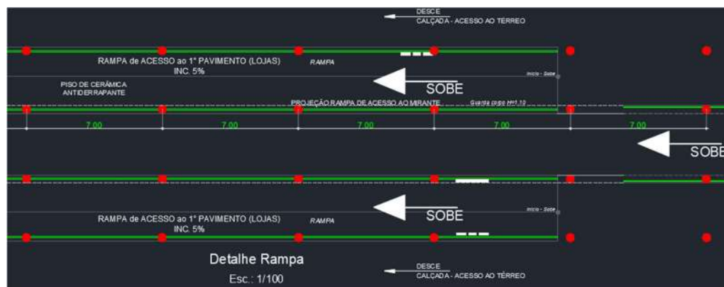
Imagem 3: Detalhe da estrutura da rampa com espaçamento a cada 7,0 m para a dilatação.
