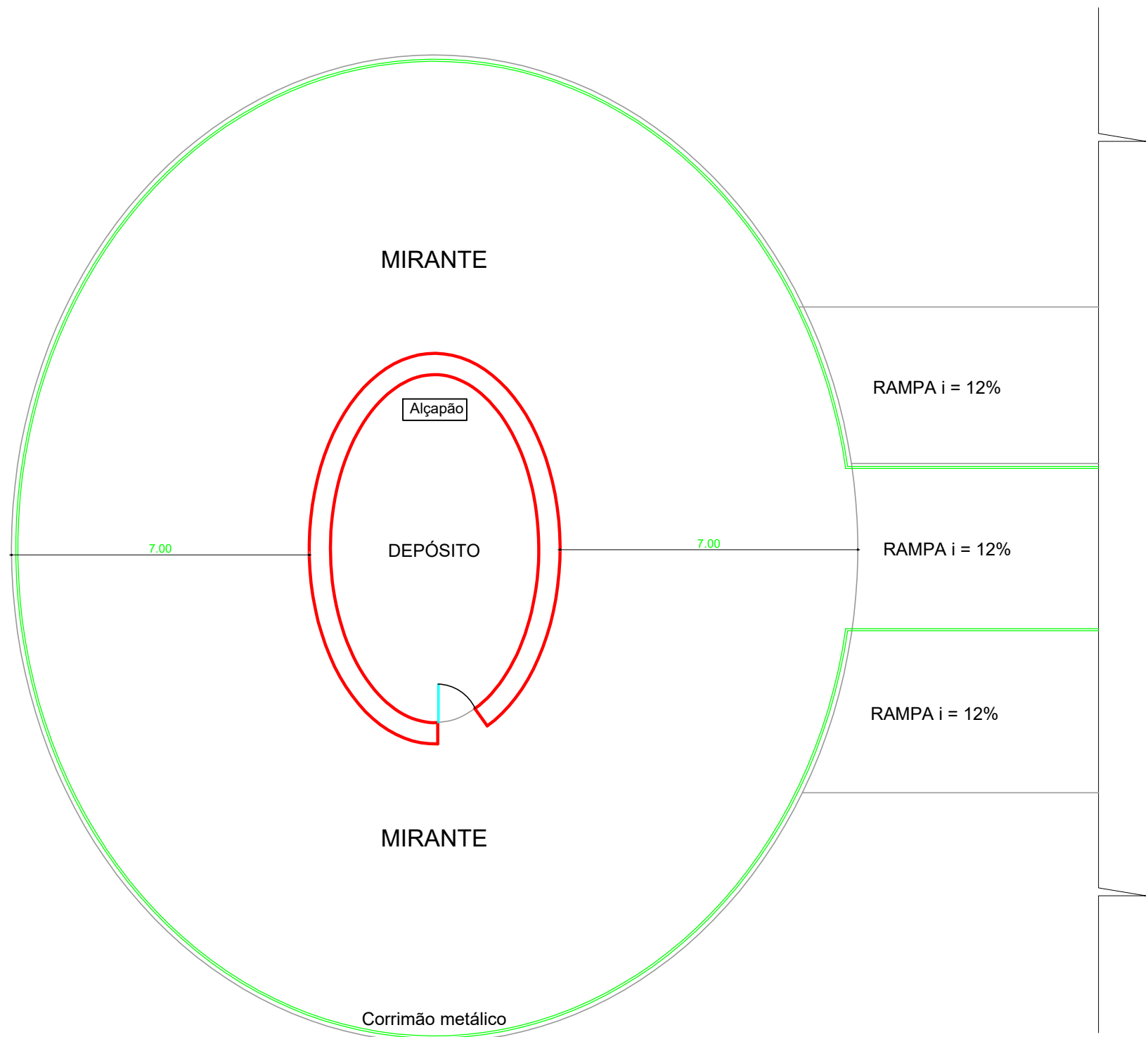
PLANTA BAIXA-2º PAV.-MIRANTE Esc.: 1/125 Área: 394,60m²
