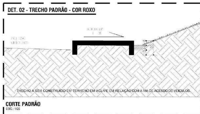
Imagem 4: Utilização canaleta meia cana para conduzir sedimentos e material soltos
