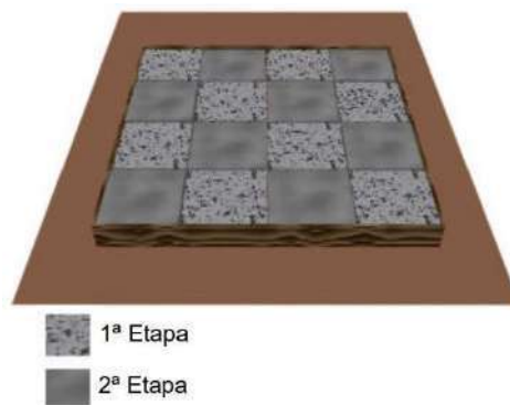
Imagem 2: Quadro de concretagem alternada (fonte: Cehop/orse)
