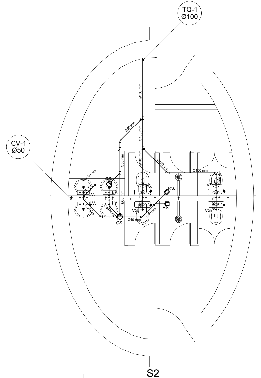
02 PLANTA BAIXA Esc: 1/100 ESGOTO SANITÁRIO 1º PAVIMENTO
